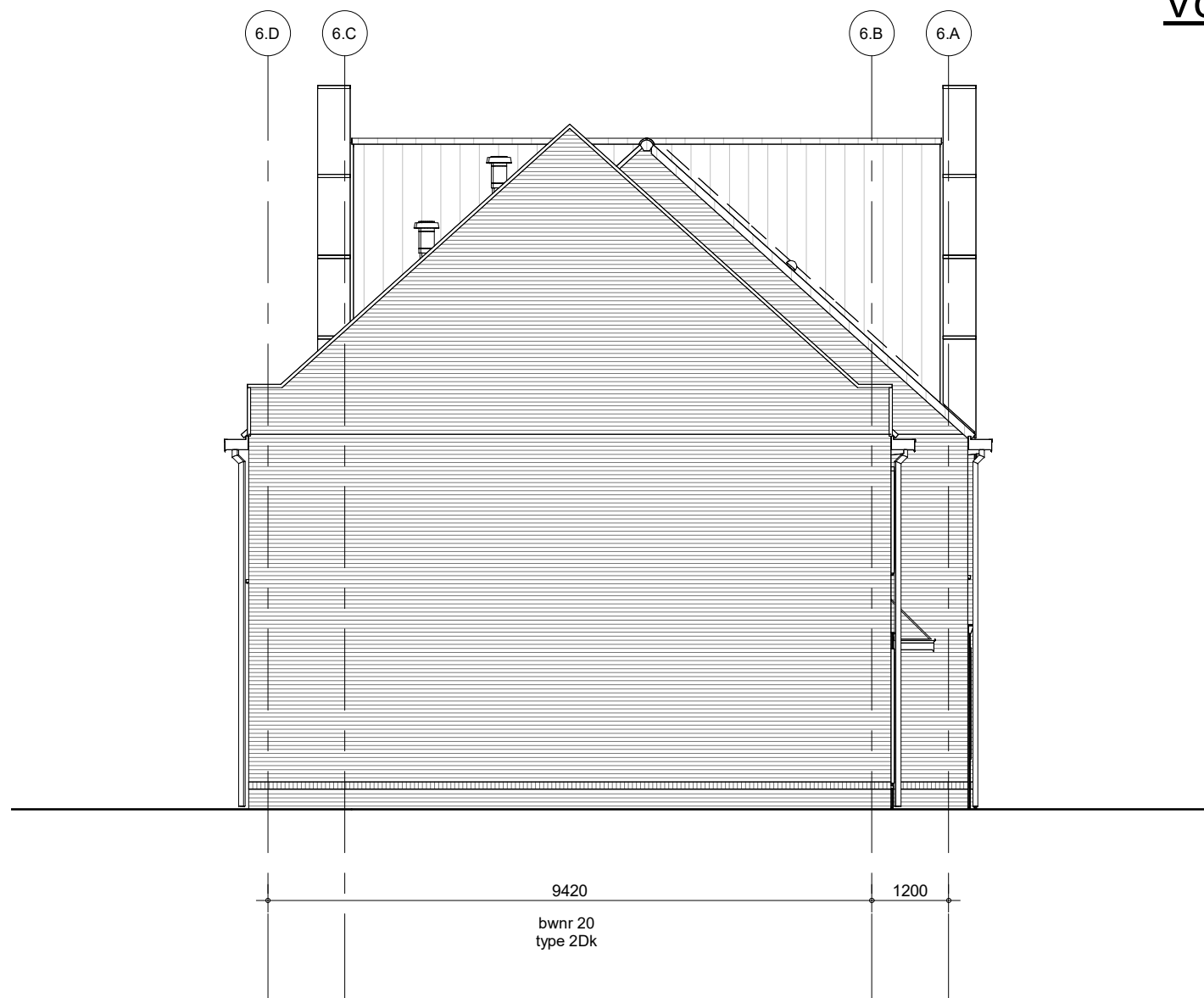
Linkerzijgevel - Blok 06
