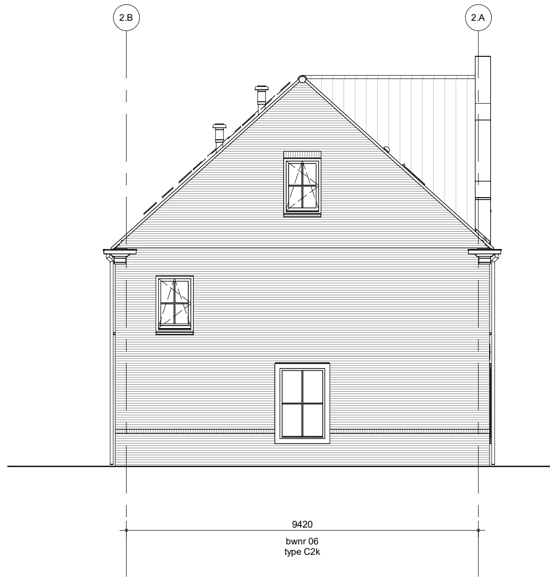
Linker zijgevel - Blok 02
