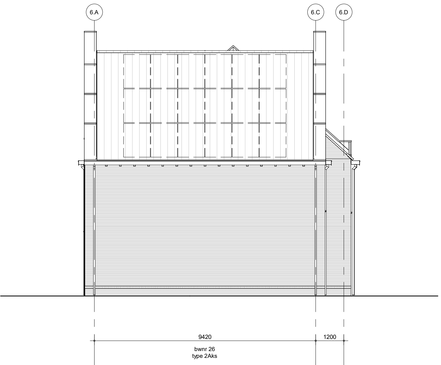
Rechterzijgevel - Blok 06
