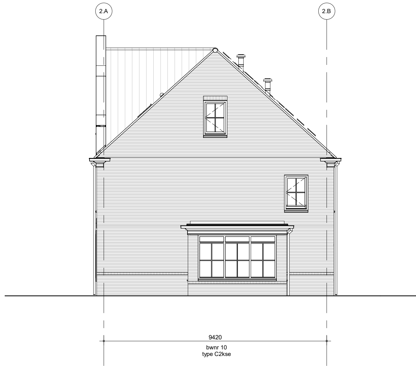
Rechter zijgevel - Blok 02
