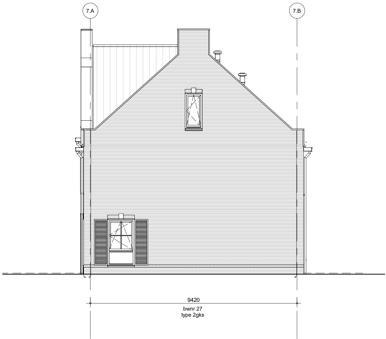
Rechter zijgevel- Blok 07
