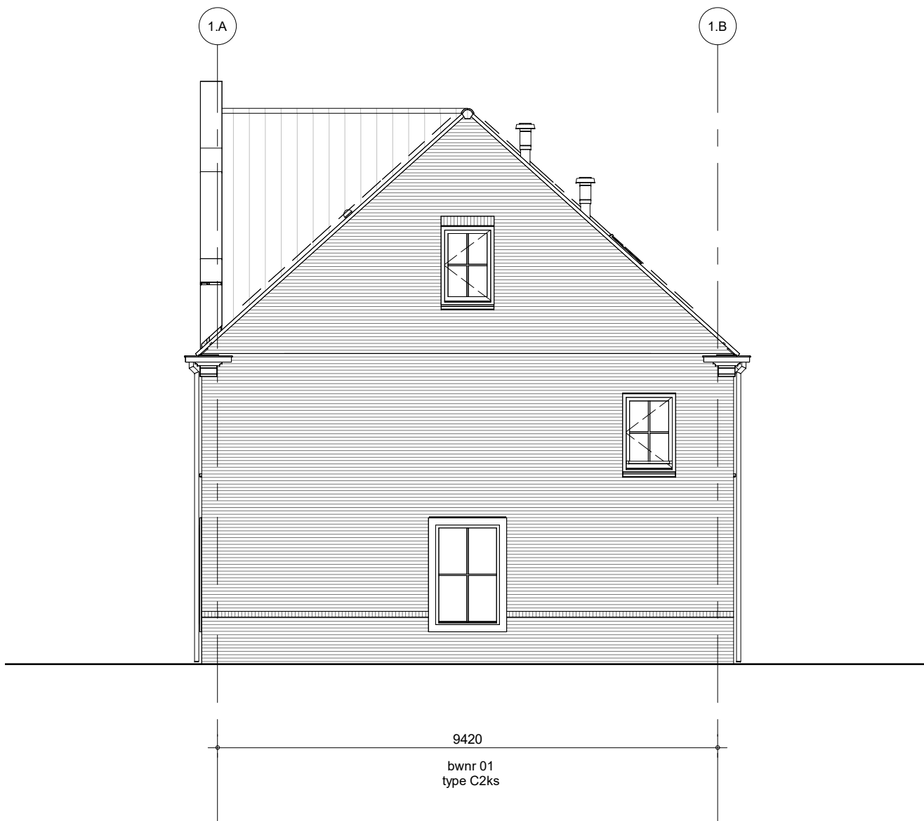
Rechter zijgevel - Blok 01
