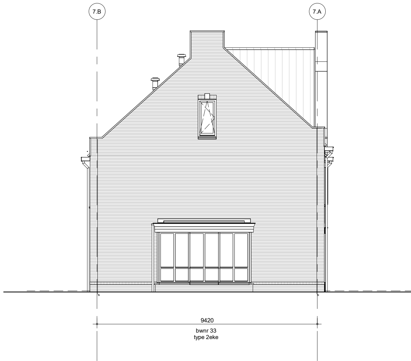
Linker zijgevel - Blok 07
