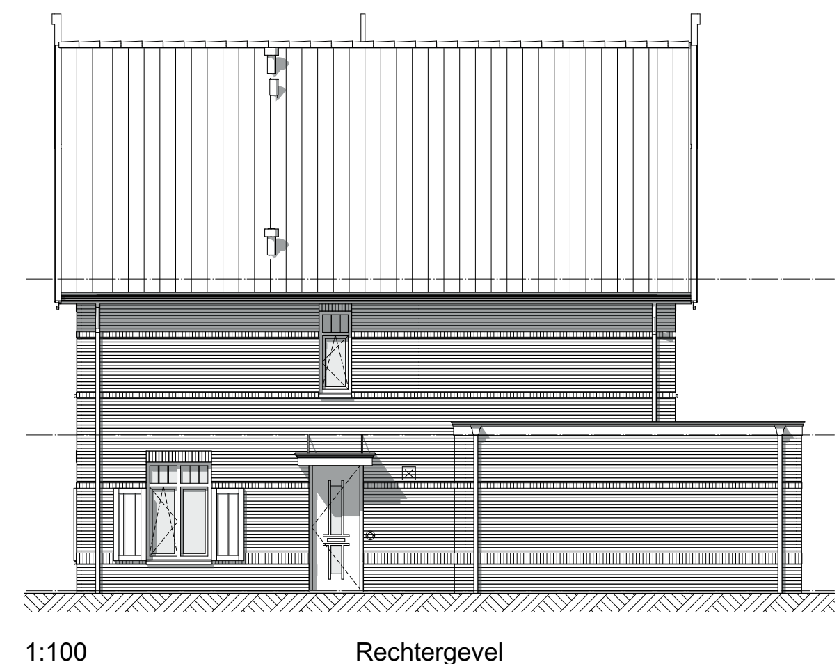
1:100 Rechtergevel
