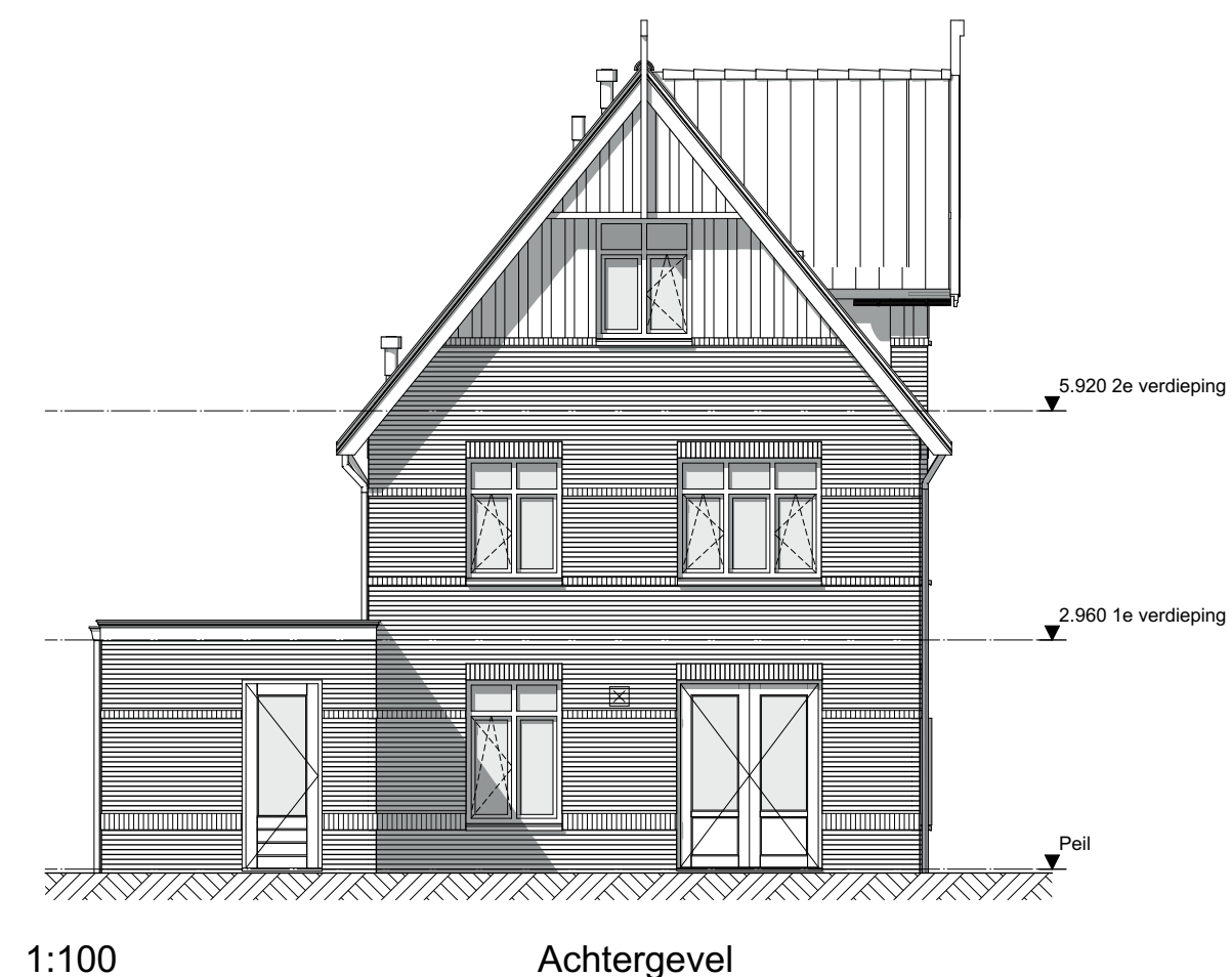
1:100 Achtergevel
