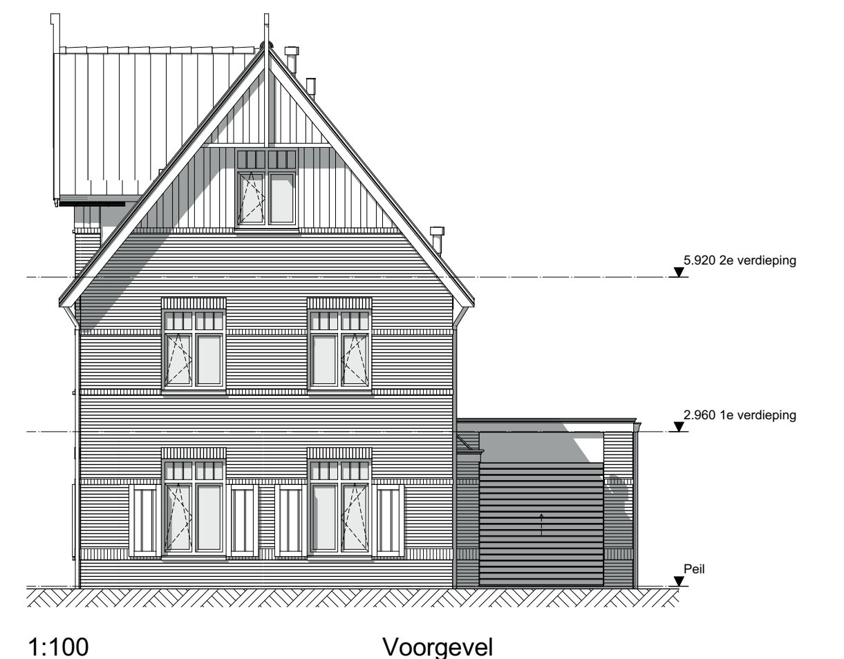
1:100 Voorgevel
