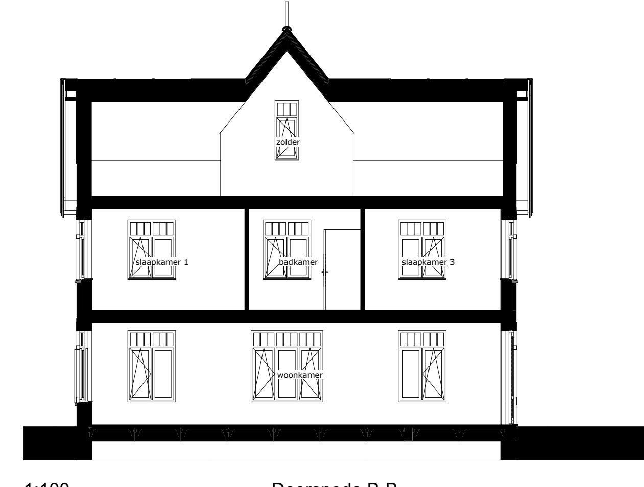
1:100 Doorsnede B-B
