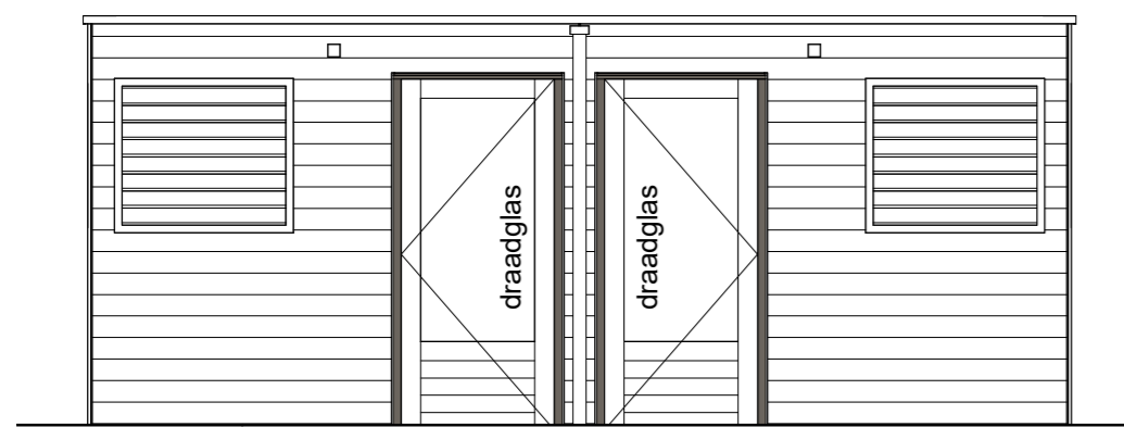
Gevel tuinzijde
