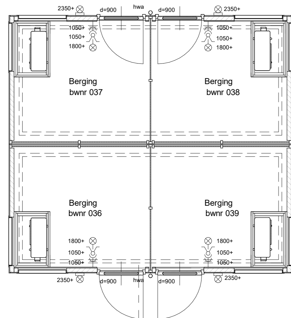
Plattegrond
