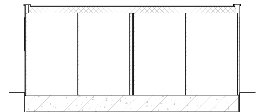
Doorsnede op palen
