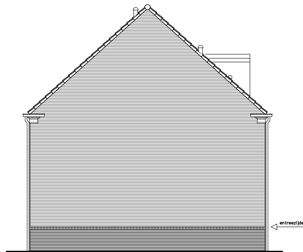
ZIJGEVEL Type C2k BWNR 42
