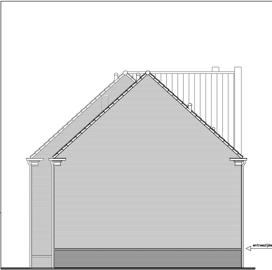
ZIJGEVEL Type C2k BWNR 101
