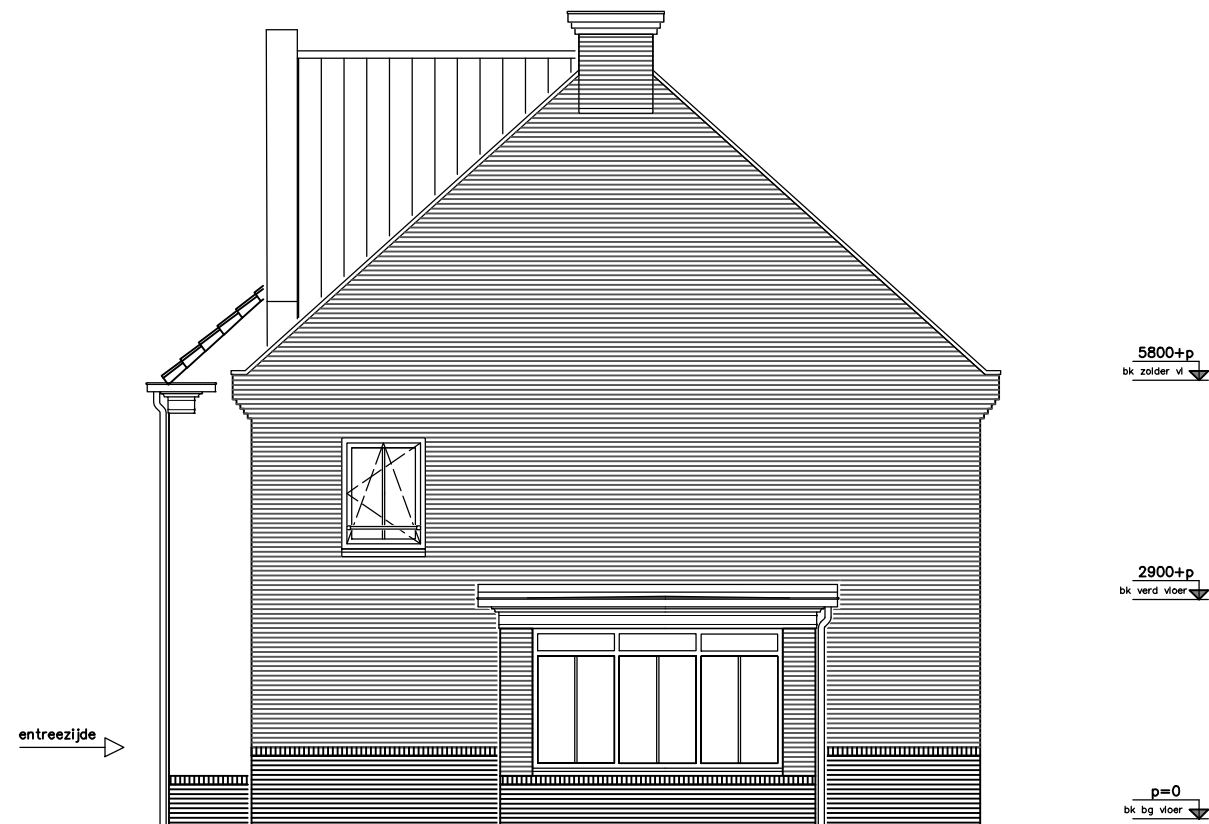
rechter zijgevel Type B4kkes bouwnr. 16
