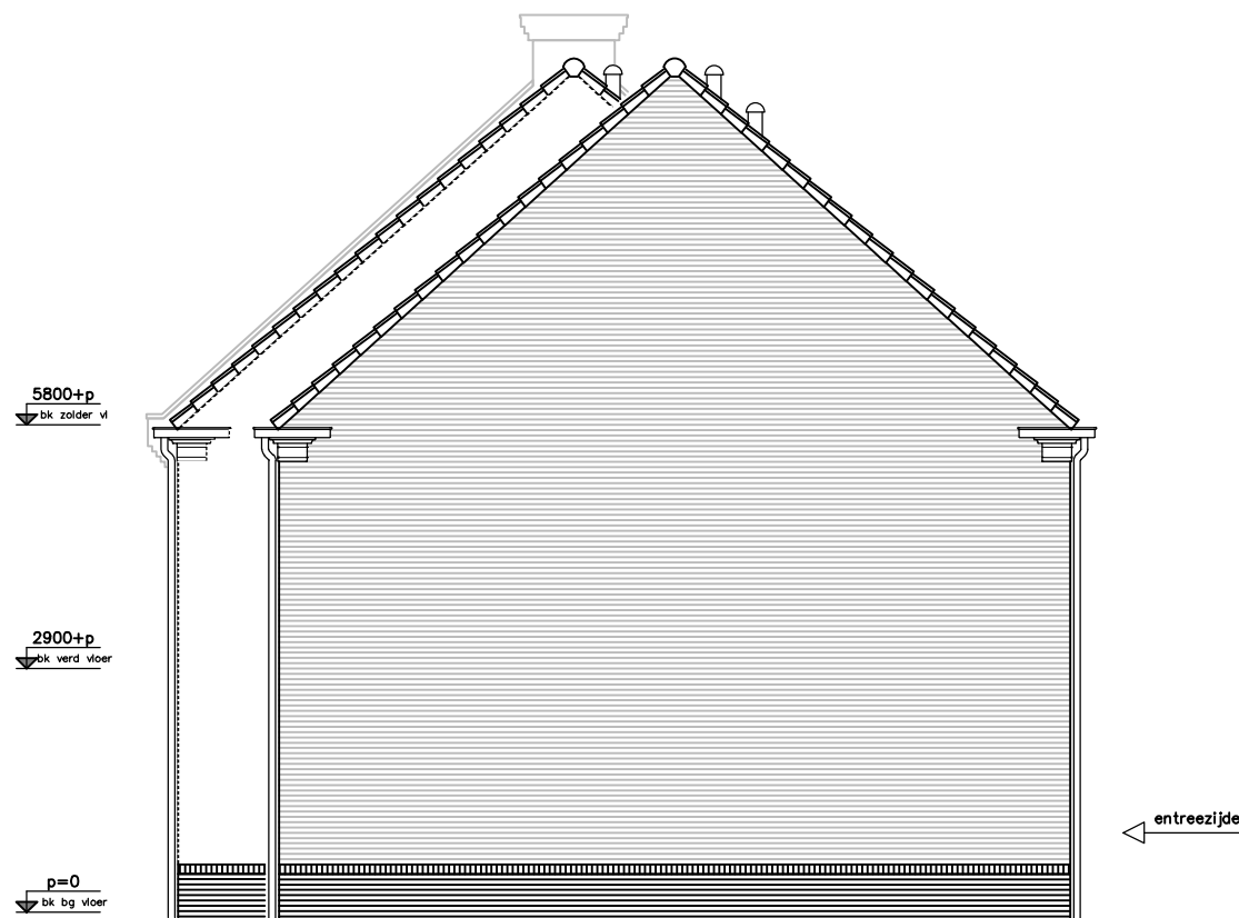
linker zijgevel Type B1k bouwnr. 9
