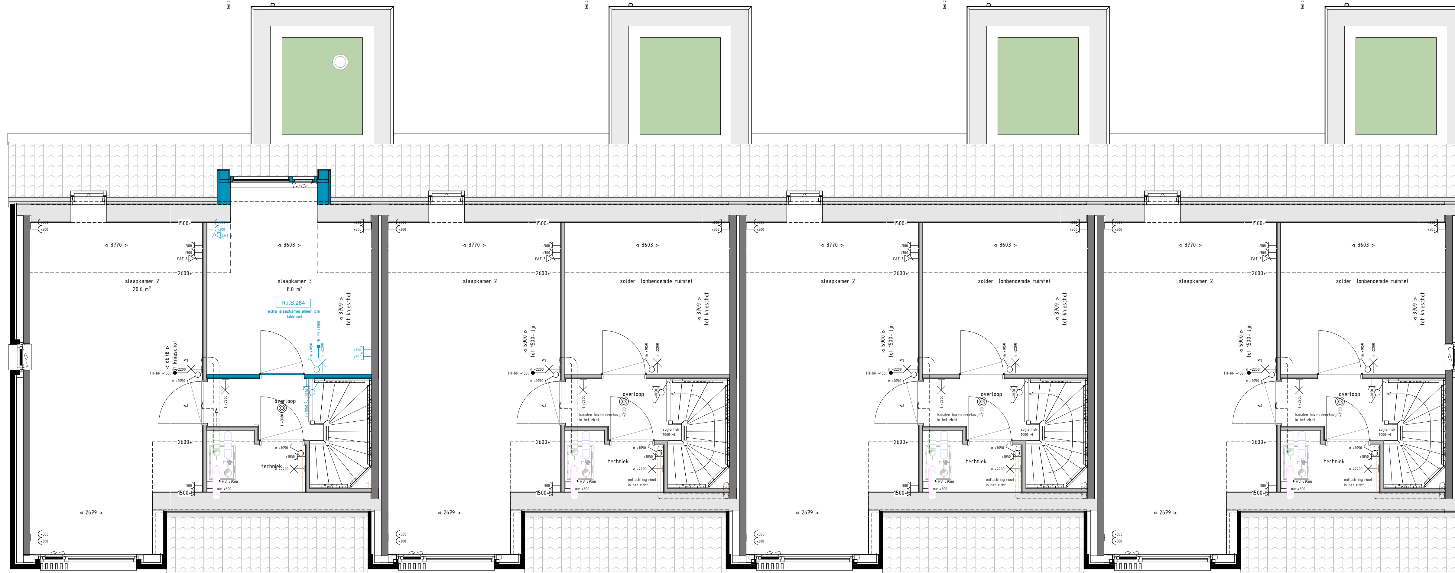
Eerste verdieping - extra slaapkamer en dakkapel
