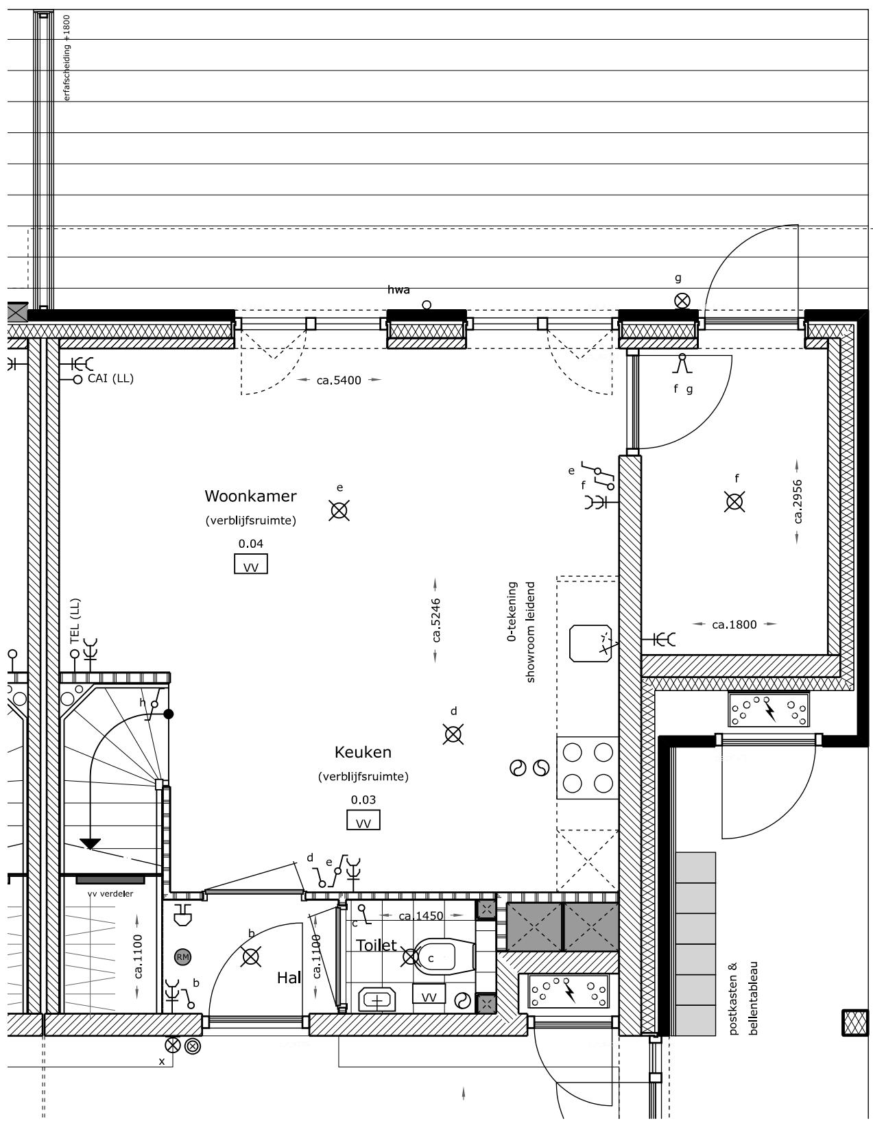
Begane grond
