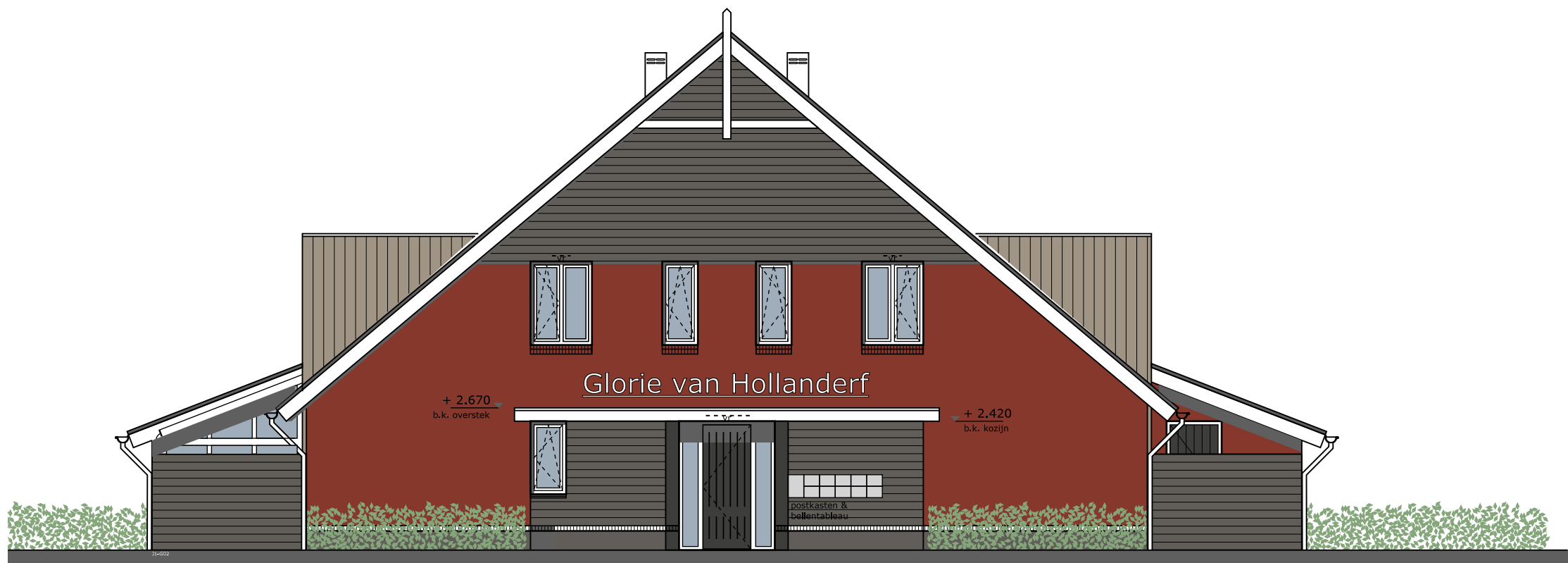
RECHTERZIJGEVEL
