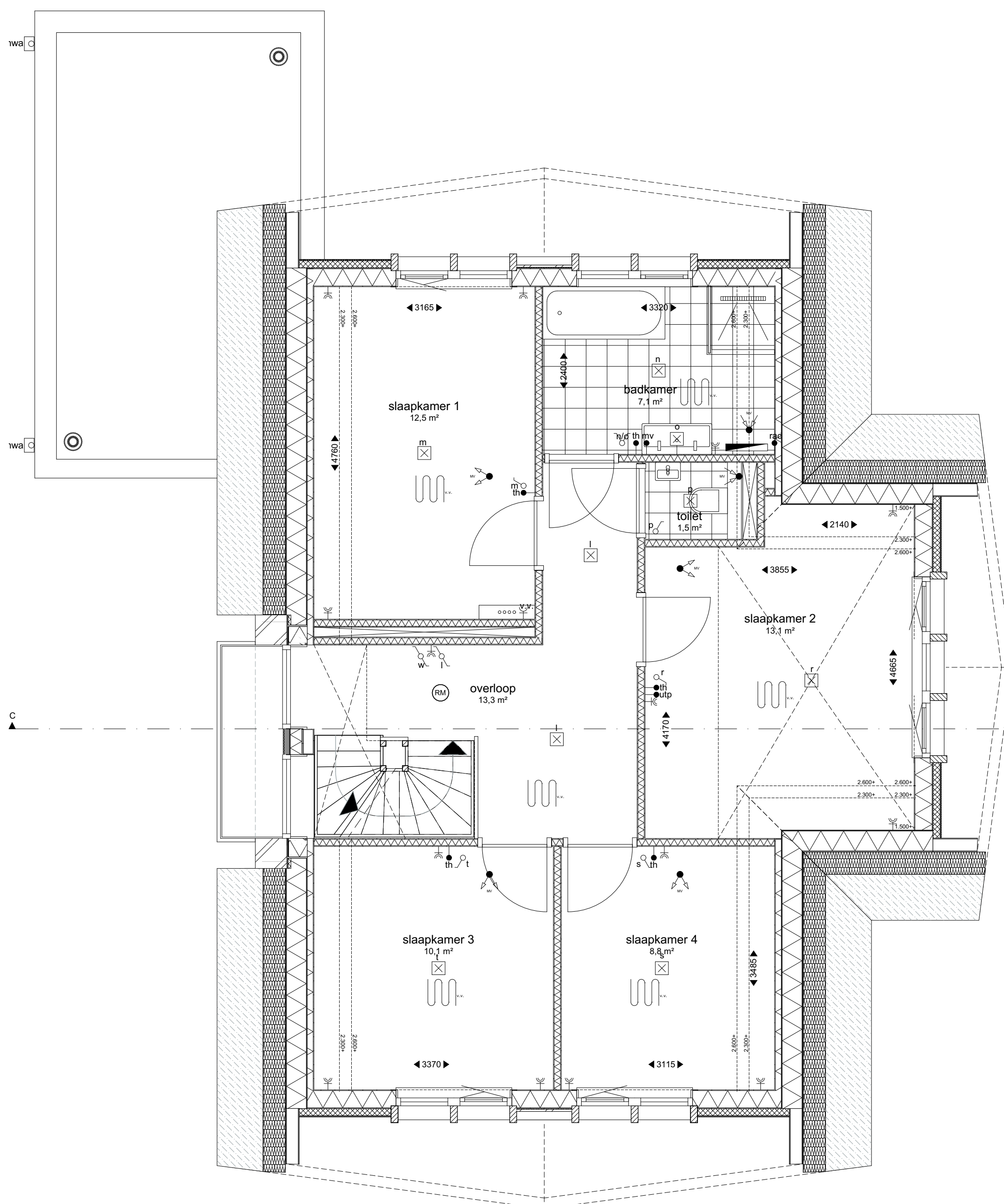
1:50 1e verdieping
