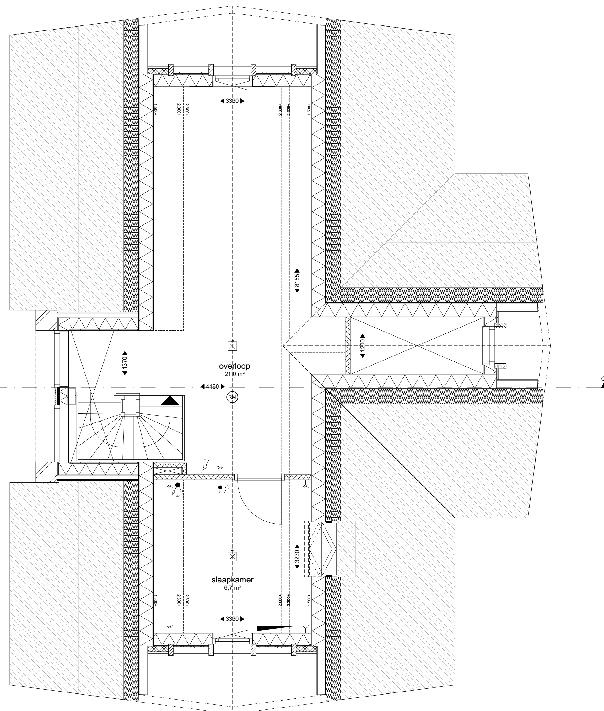
1:50 2e verdieping
