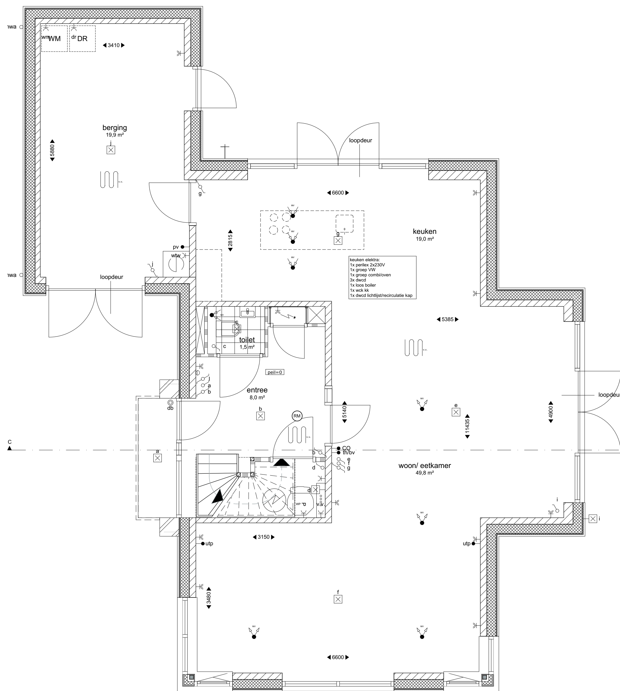
1:50 Begane grond
