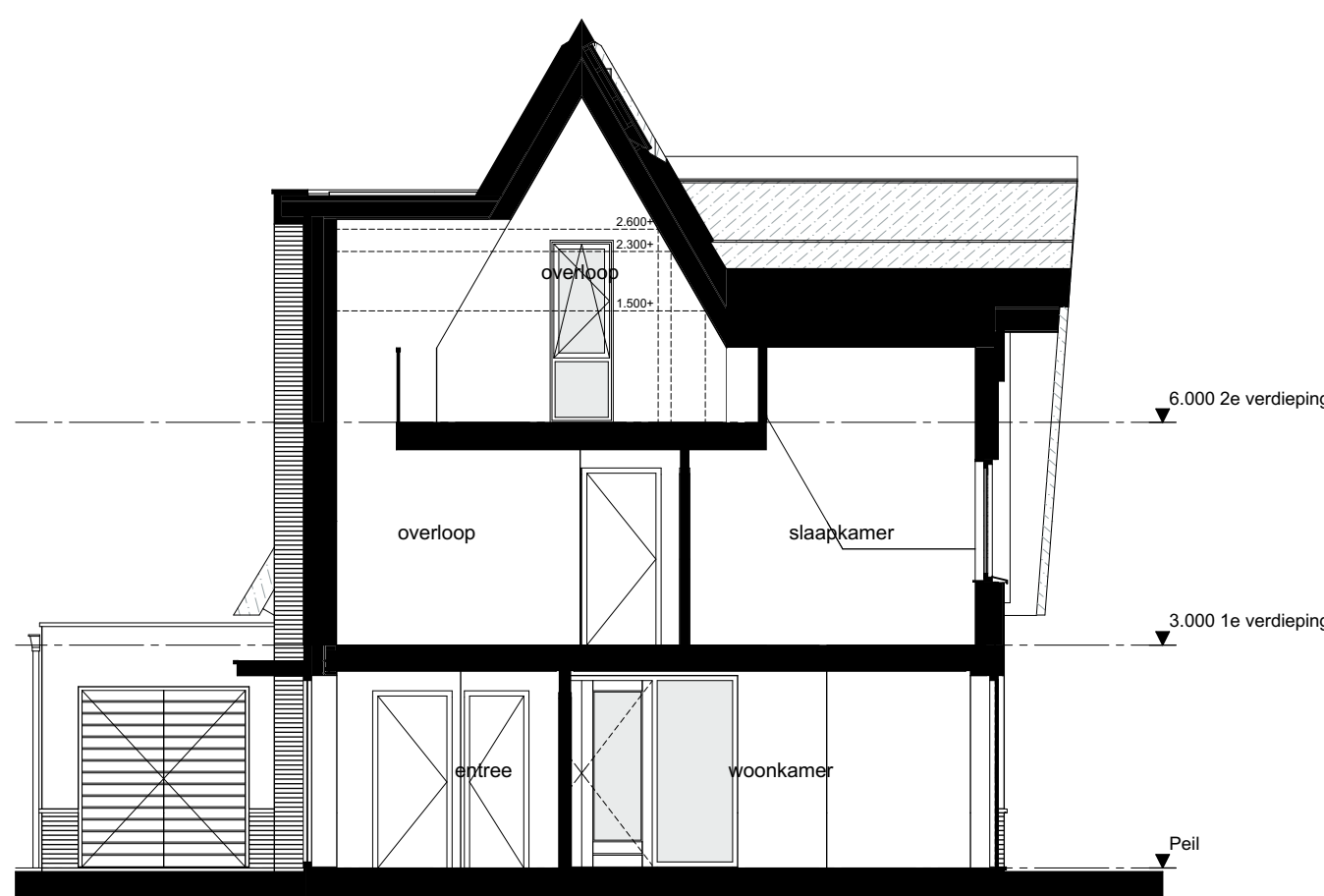
1:100 Doorsnede C-C
