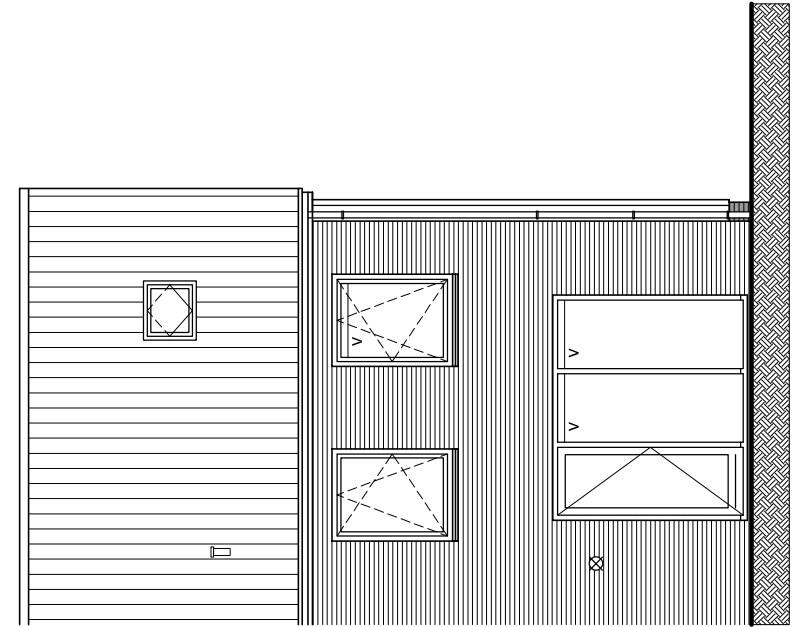
Achtergevel schaal 1:100 bouwnummer: 3
