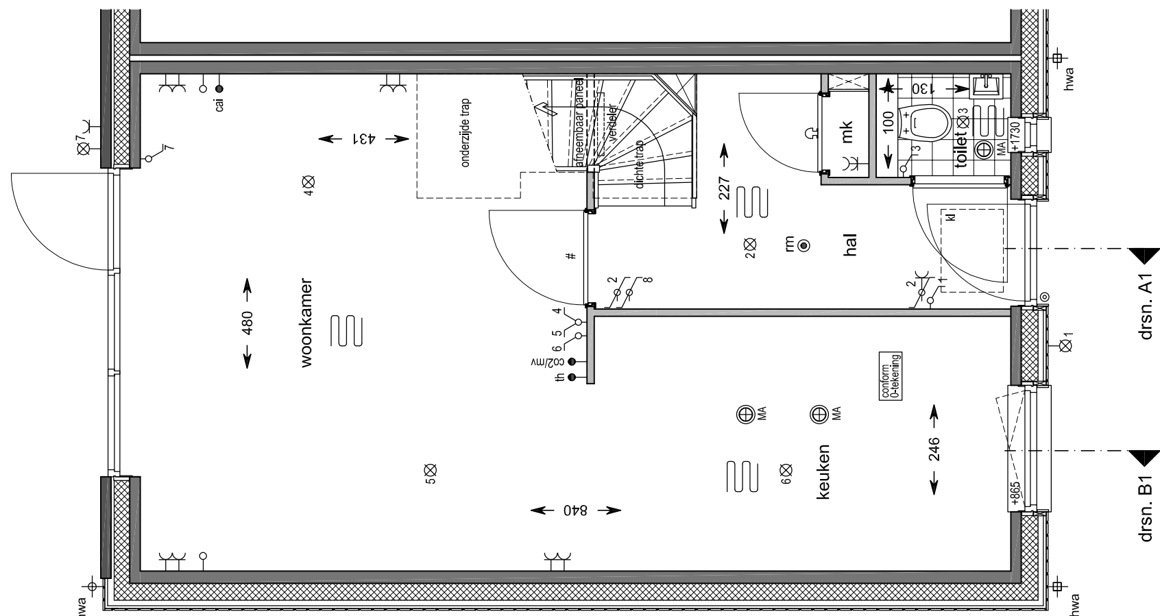
Begane grond schaal 1:50 bouwnummer: 33
