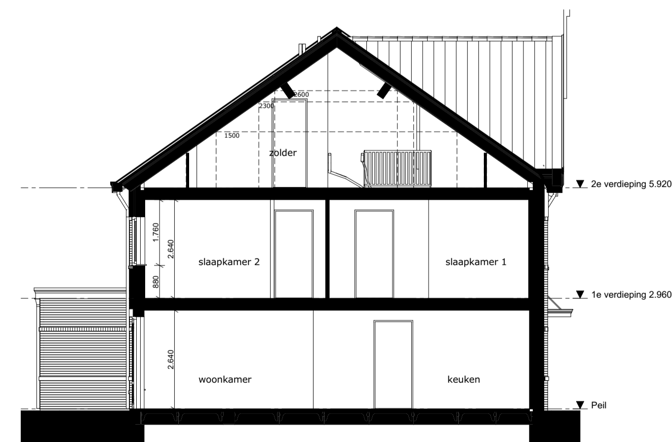
1:100 Doorsnede B-B
