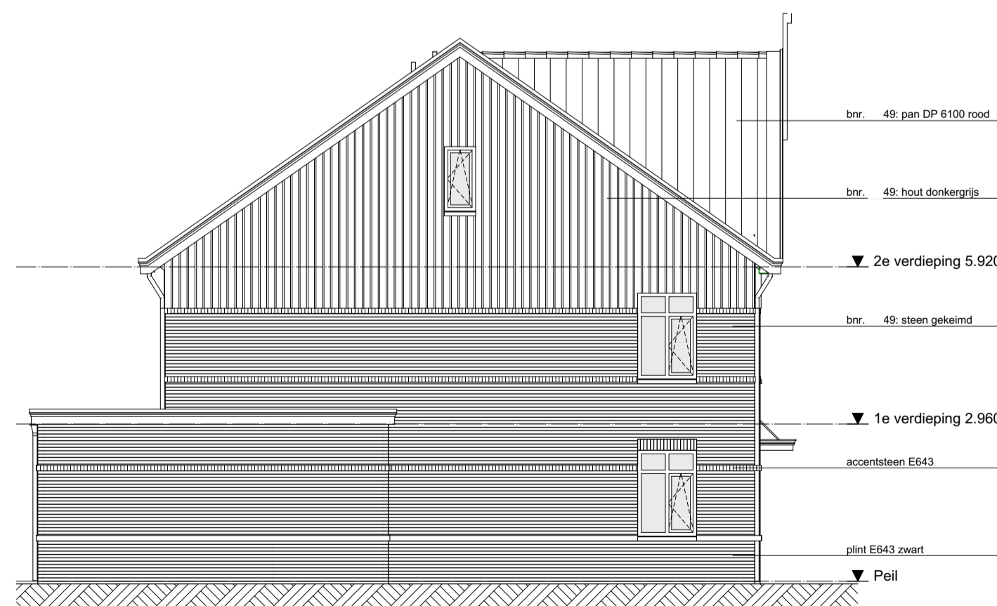
1:100 Linkergevel
