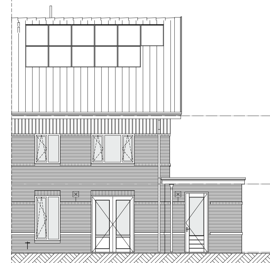
1:100 Achtergevel
