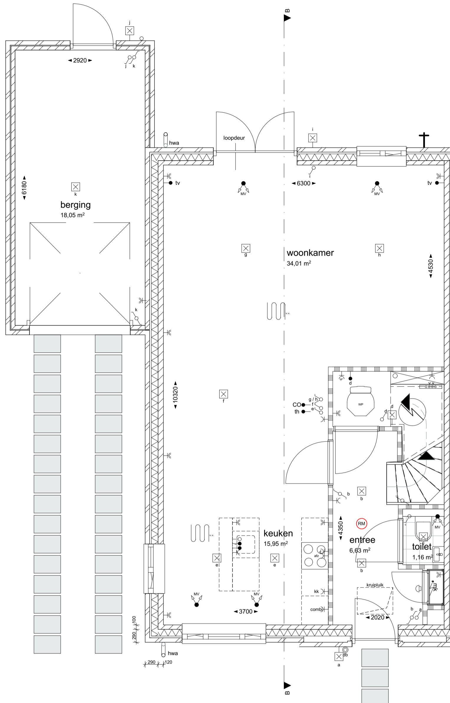
1:50 Begane grond
