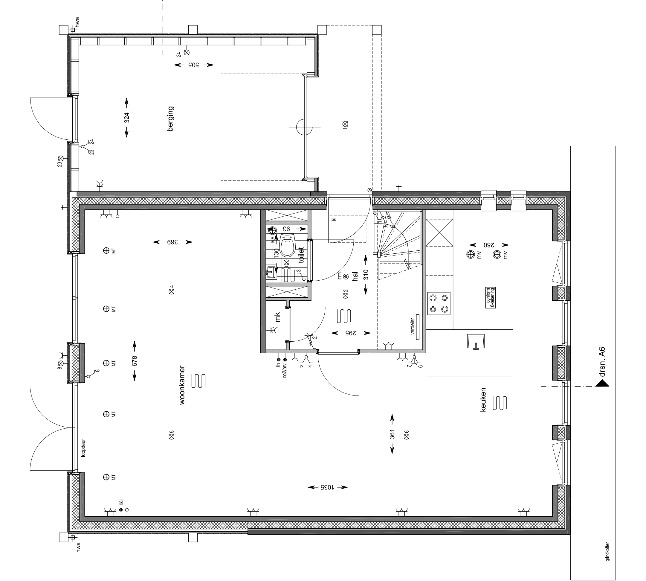
Begane grond schaal 1:50 bouwnummer : 73
