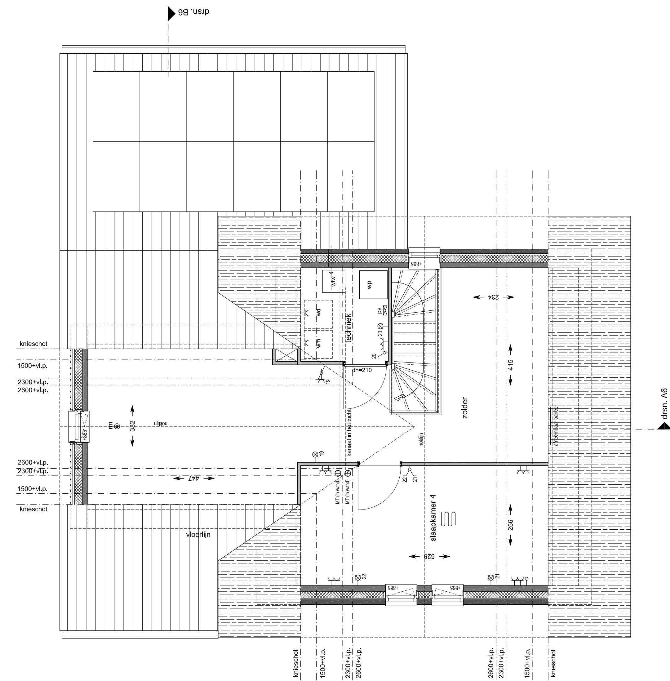
2e Verdieping schaal 1:50 bouwnummer : 73
