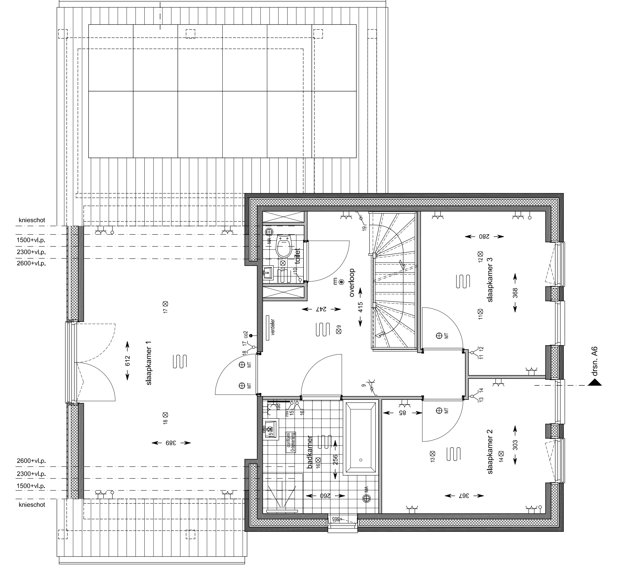
1e Verdieping schaal 1:50 bouwnummer : 73
