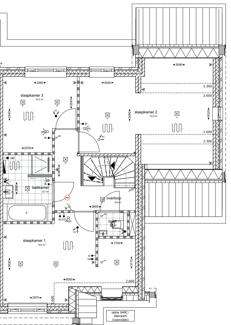
1:100 1e verdieping
