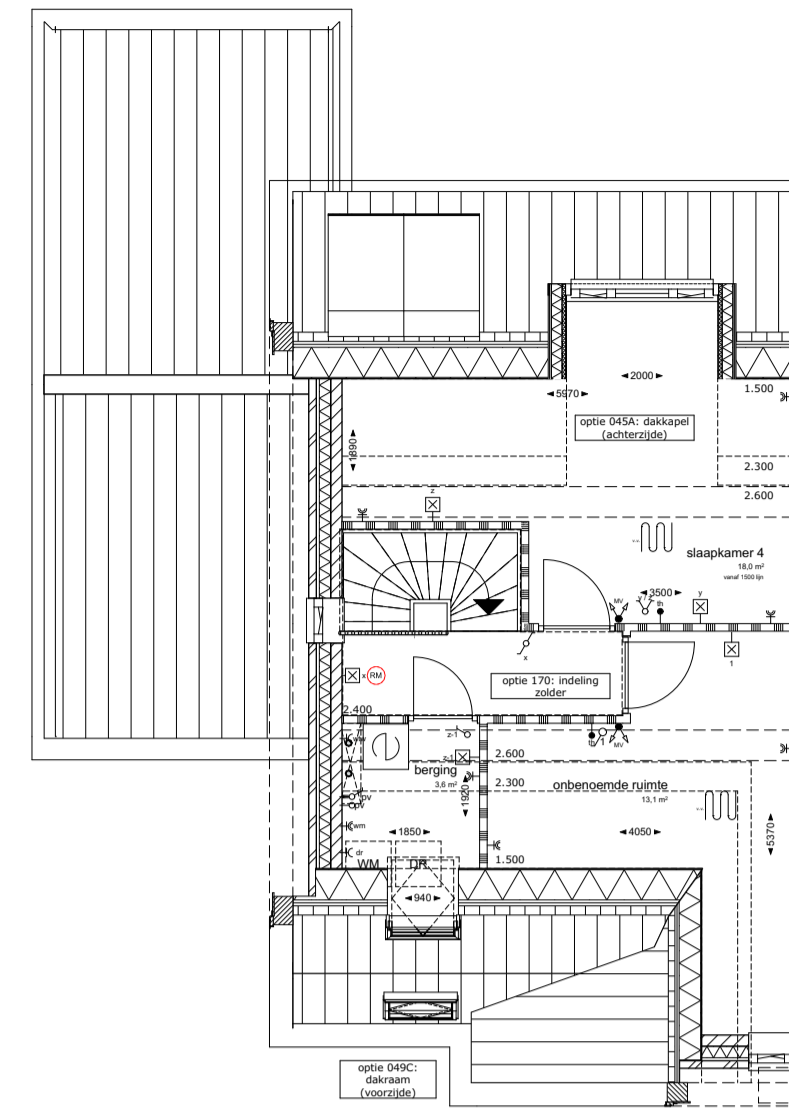
1:100 2e verdieping
