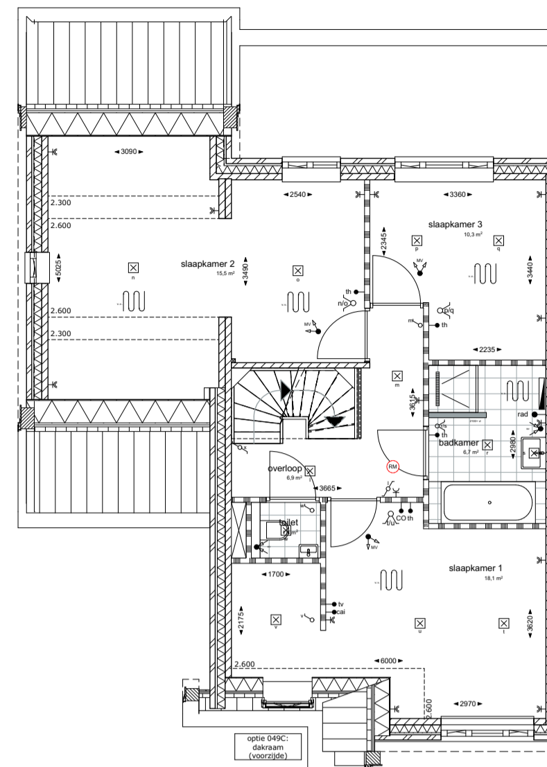
1:100 1e verdieping
