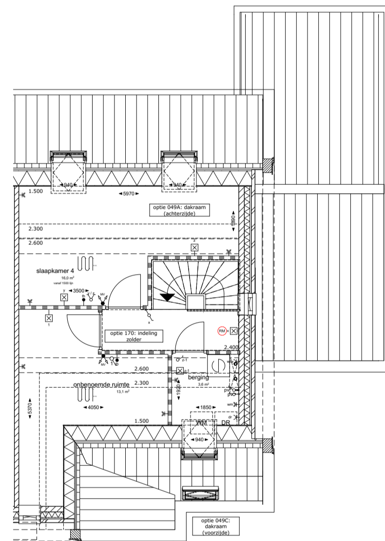
1:100 2e verdieping
