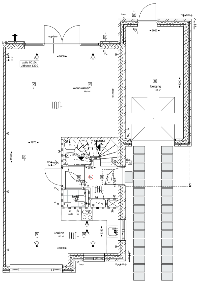
1:100 Begane grond
