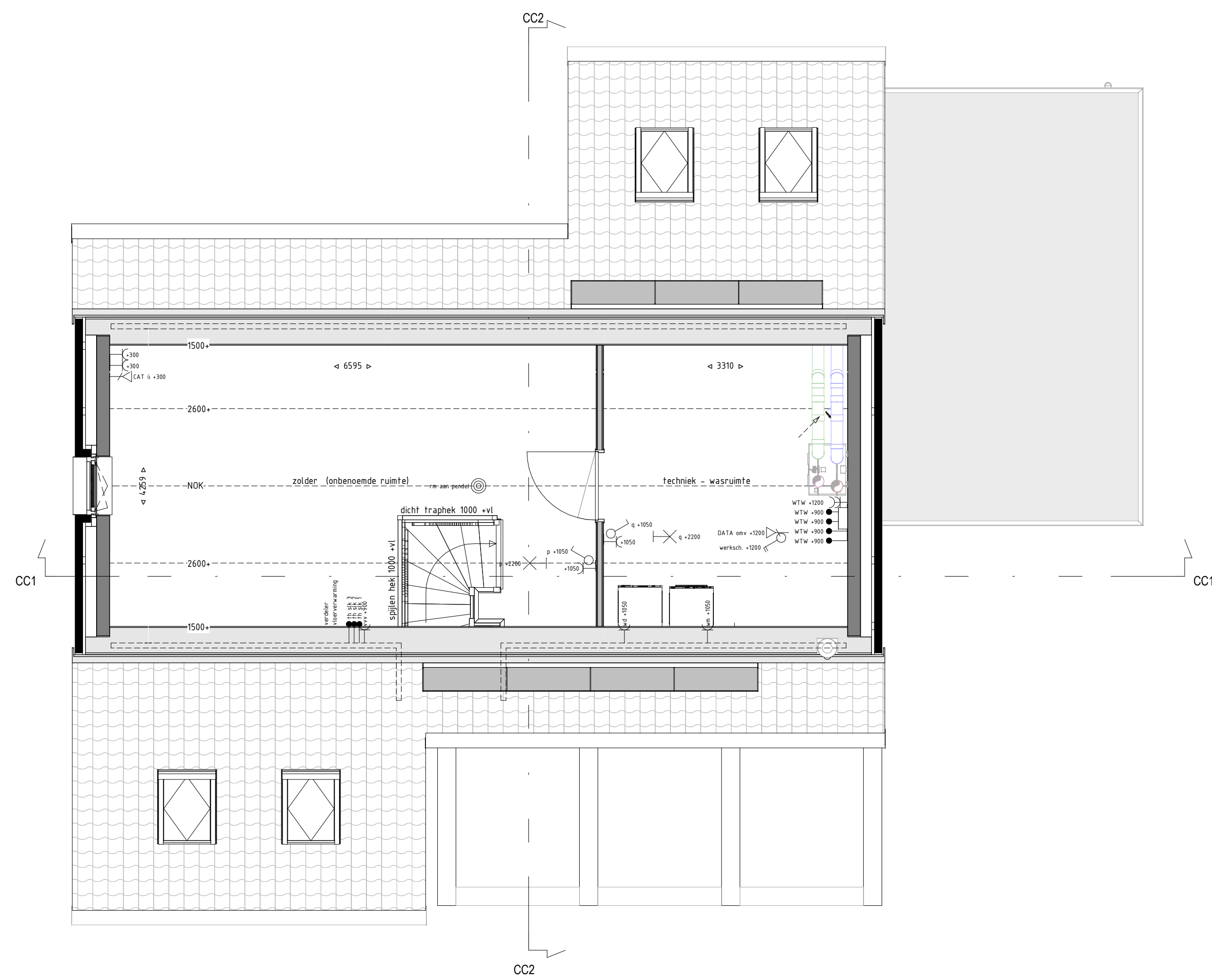
Tweede verdieping 1 : 50
