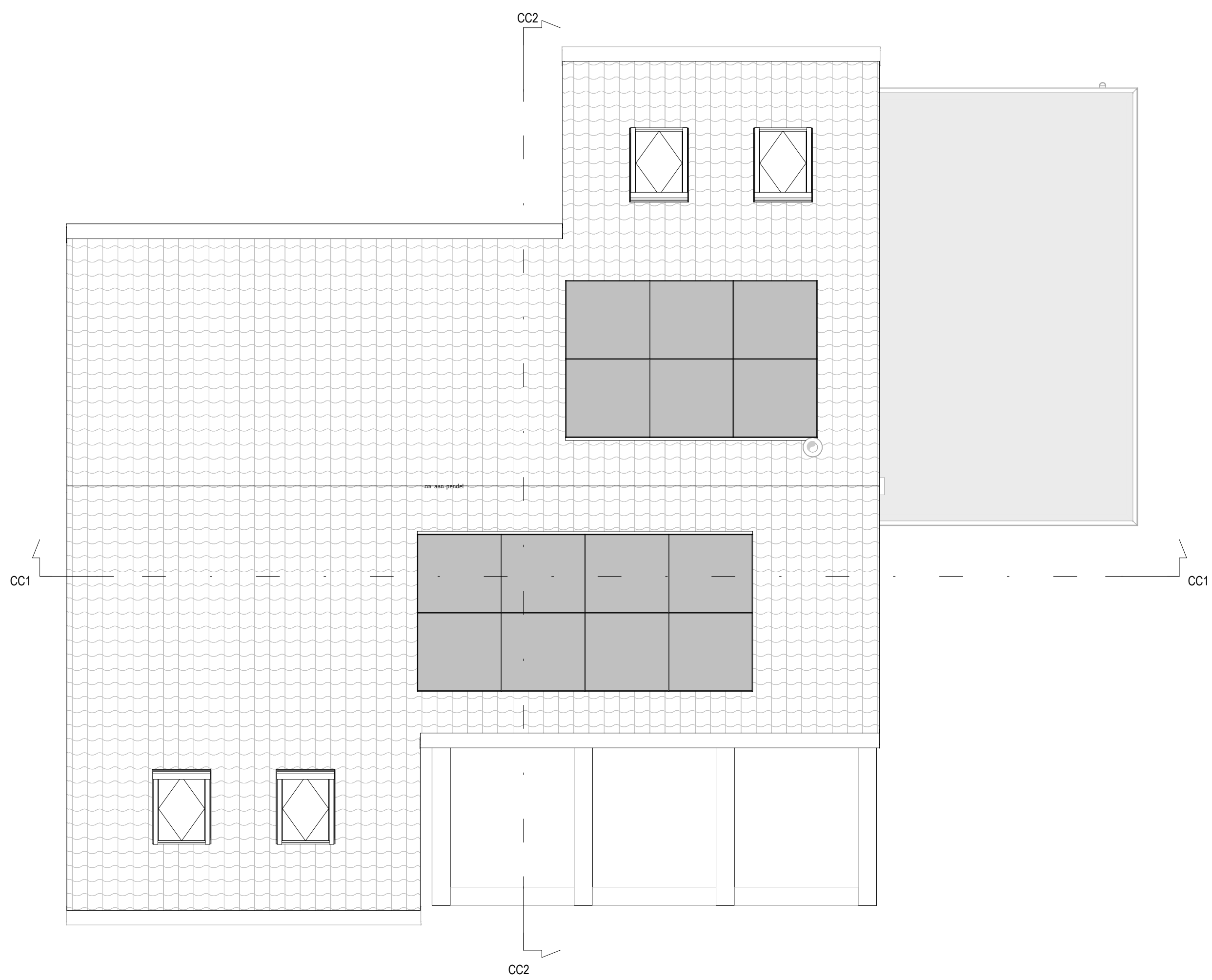
Dak 1 : 50
