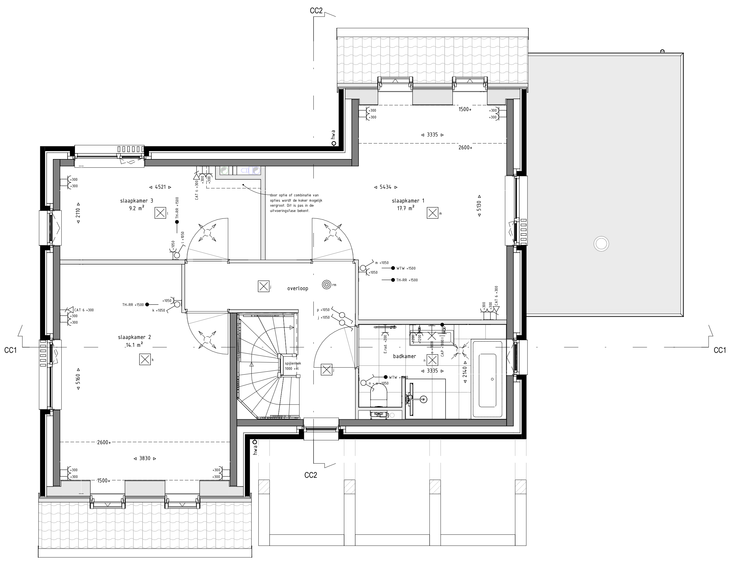
Eerste verdieping 1 : 50
