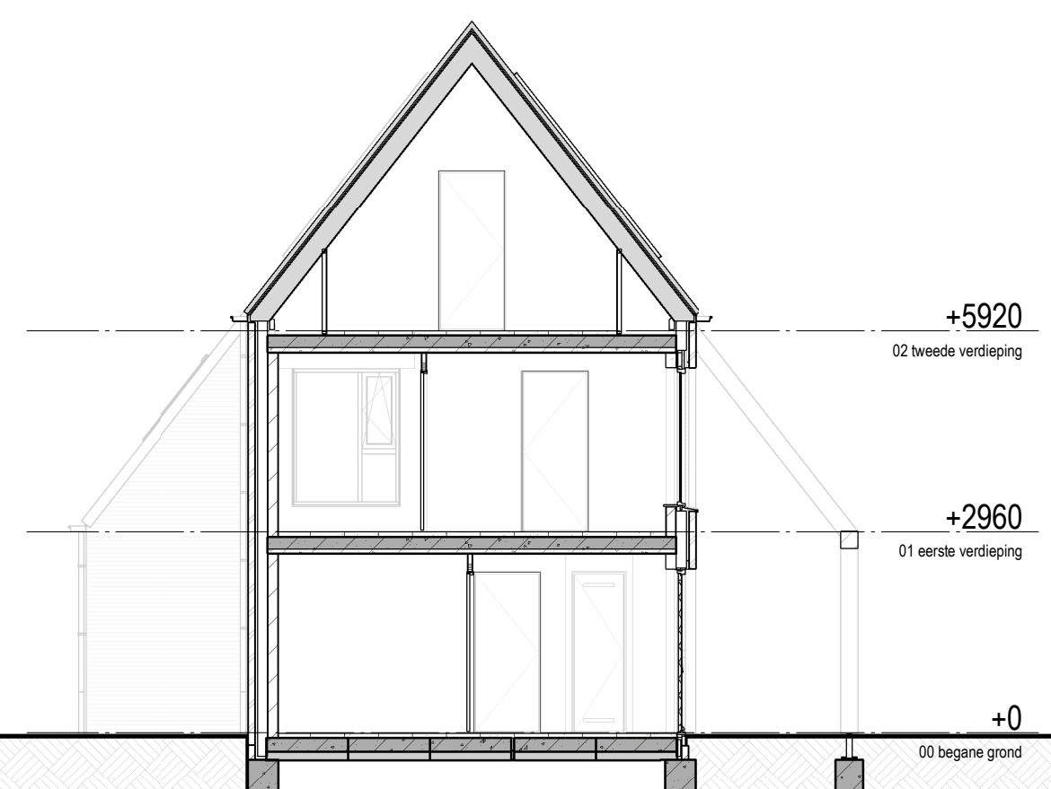
Doorsnede AA2 1 : 100
