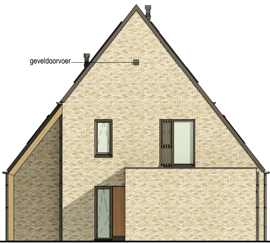
Rechter zijgevel 1 : 100
