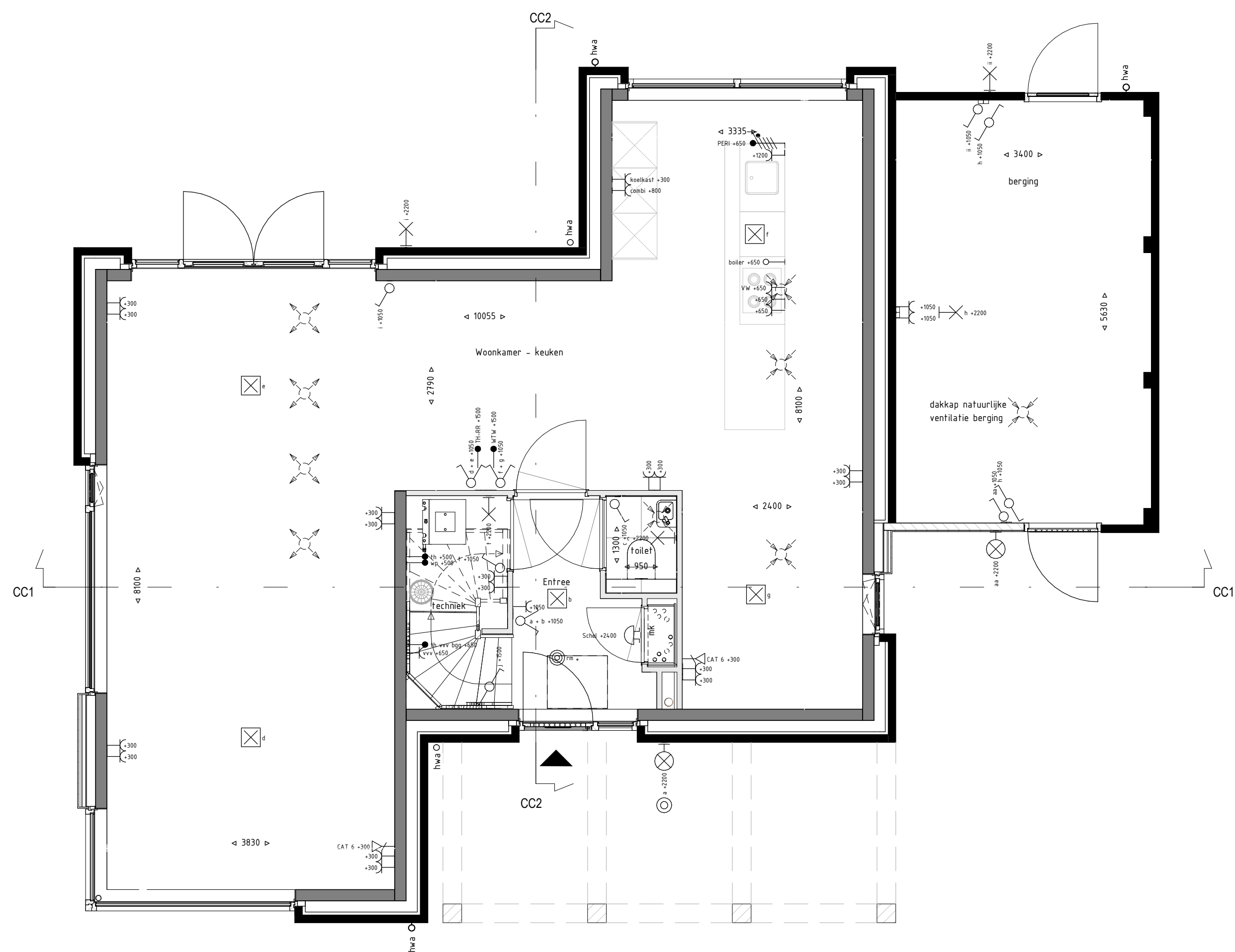
Begane grond 1 : 50
