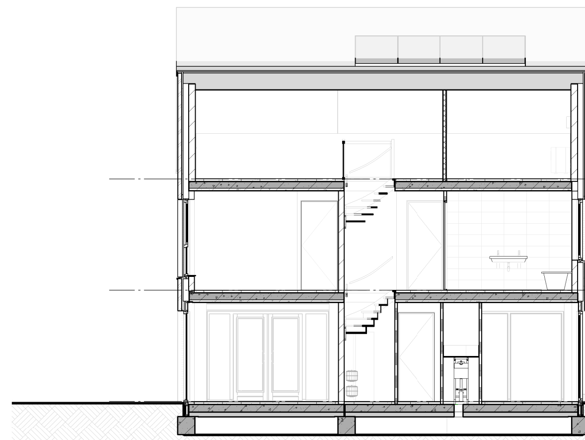
Doorsnede C1 1 : 100
