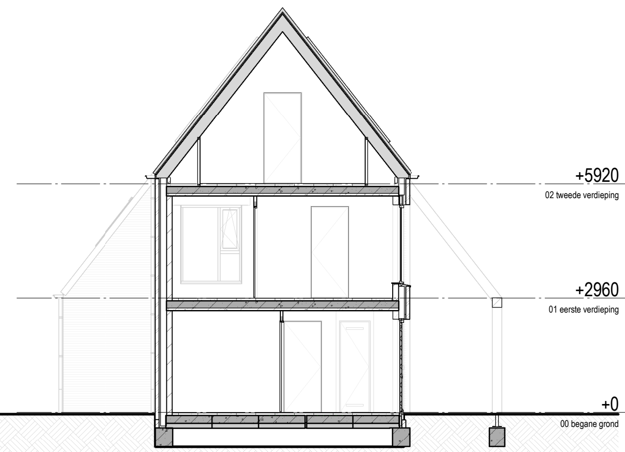
Doorsnede C2 1 : 100
