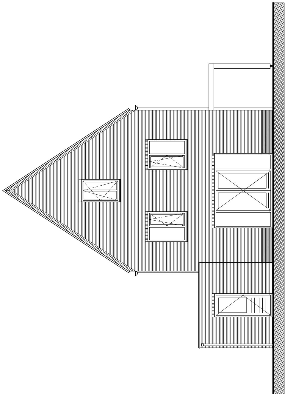
Achtergevel schaal 1:100 bouwnummer : 54
