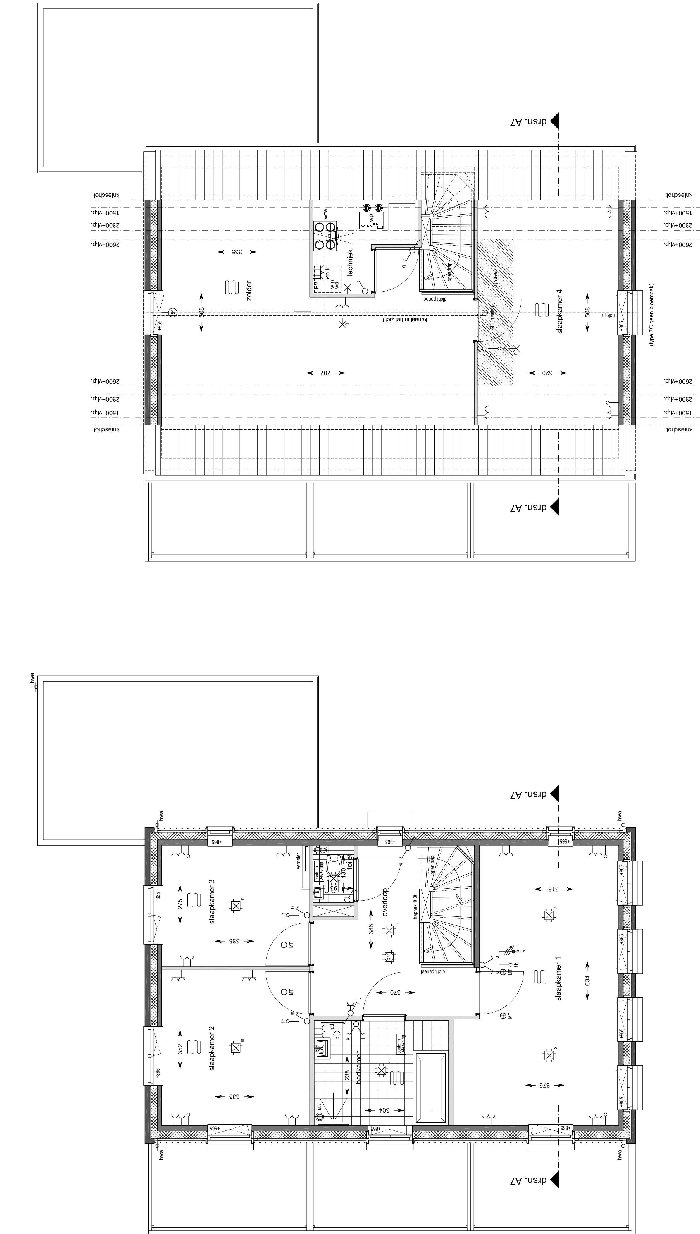
1e Verdieping schaal 1:50 bouwnummer : 54
