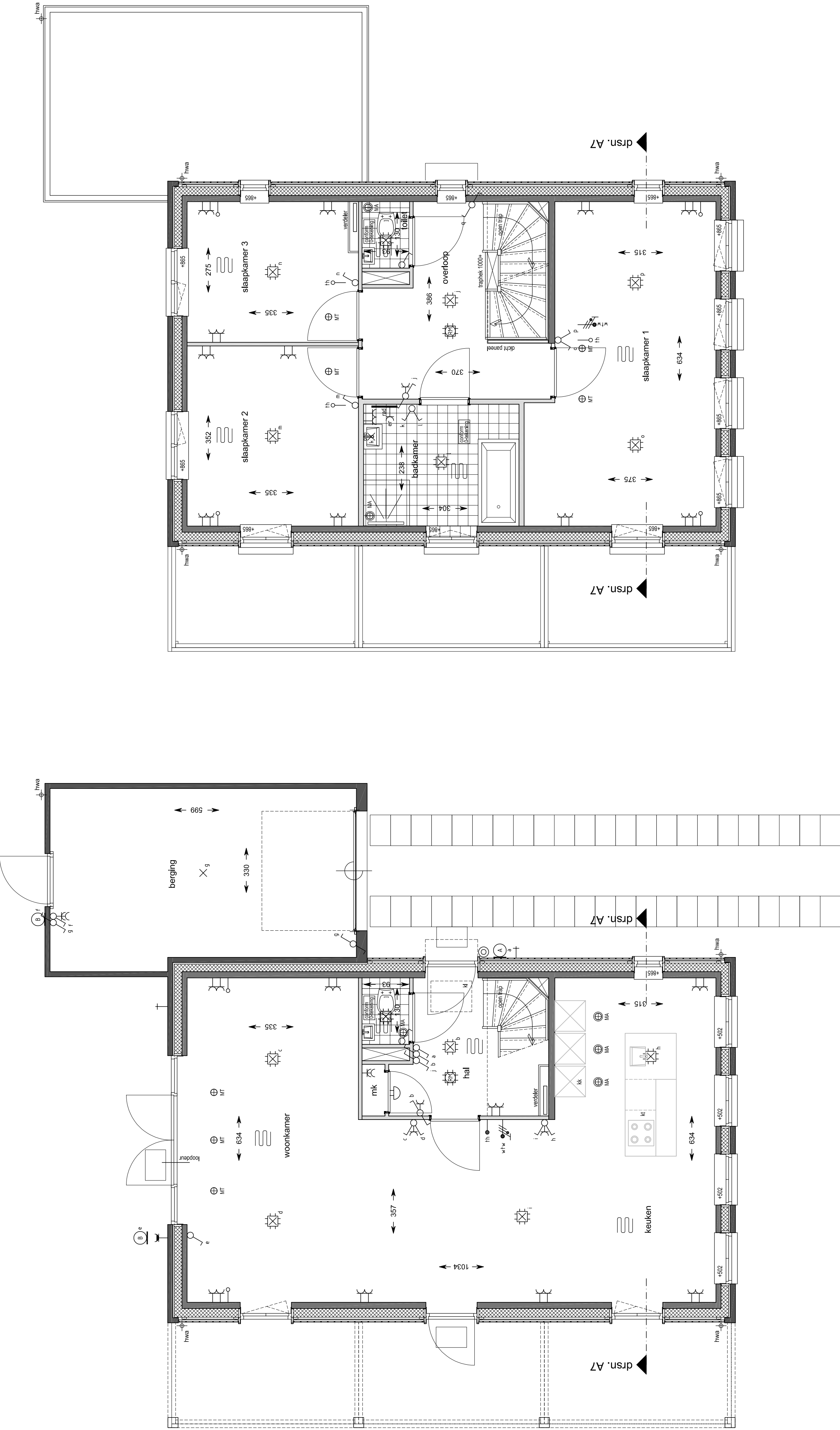
Begane grond schaal 1:50 bouwnummer : 54
