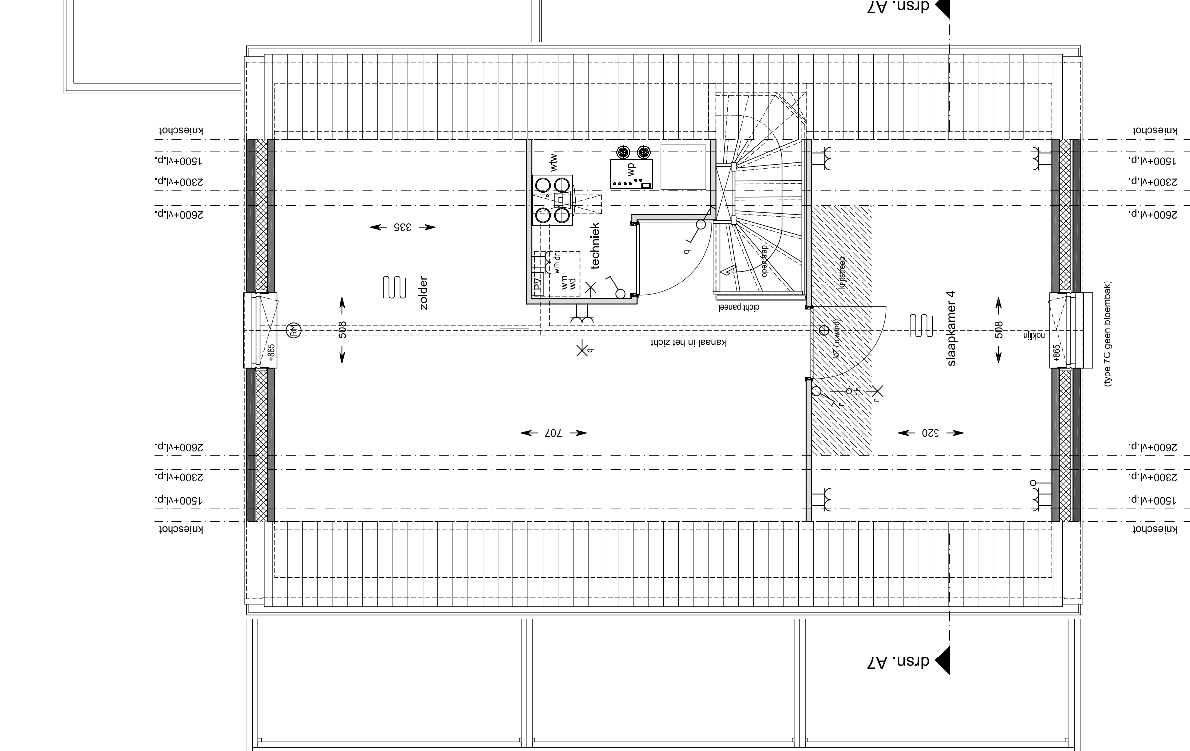
2e Verdieping schaal 1:50 bouwnummer : 54
