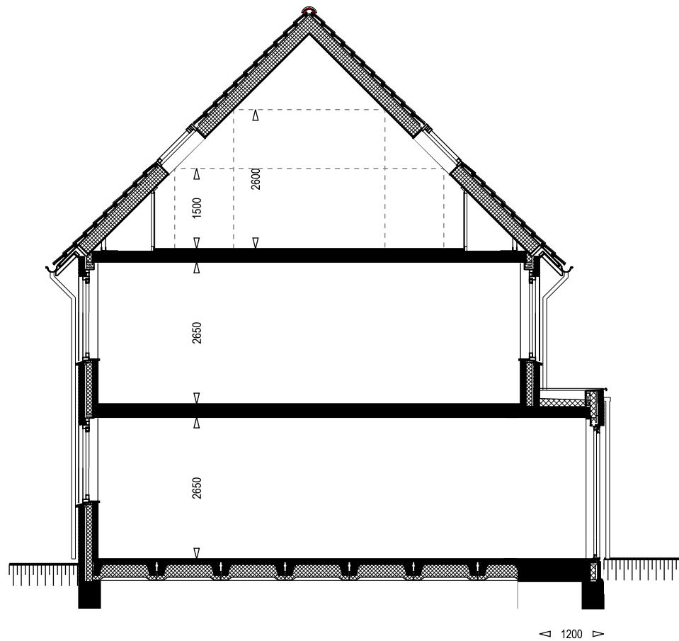
type A uitbouw 1200 mm optie dakraam voor optie dakraam achter
