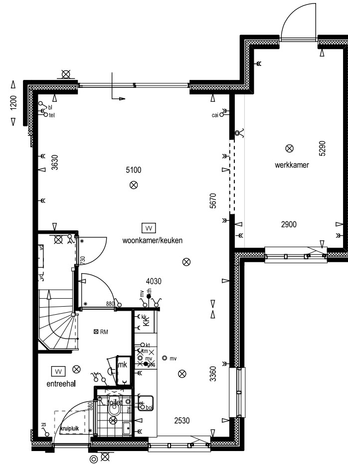
type A2/A3 optie uitbouw 1200 mm optie garage bij woonkamer i.c.m. uibouw
