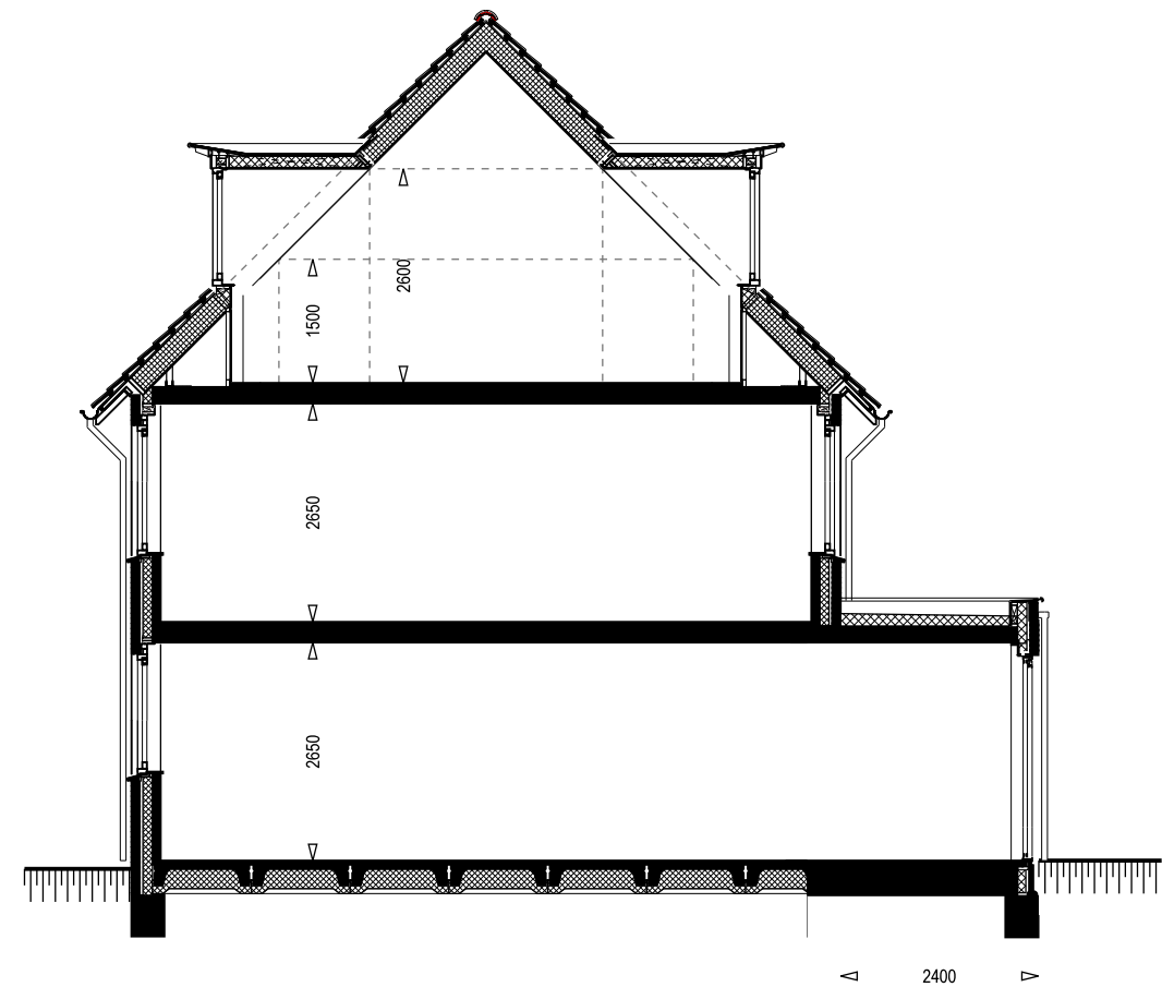
type A uitbouw 2400 mm optie dakkapel voor optie dakkapel achter
