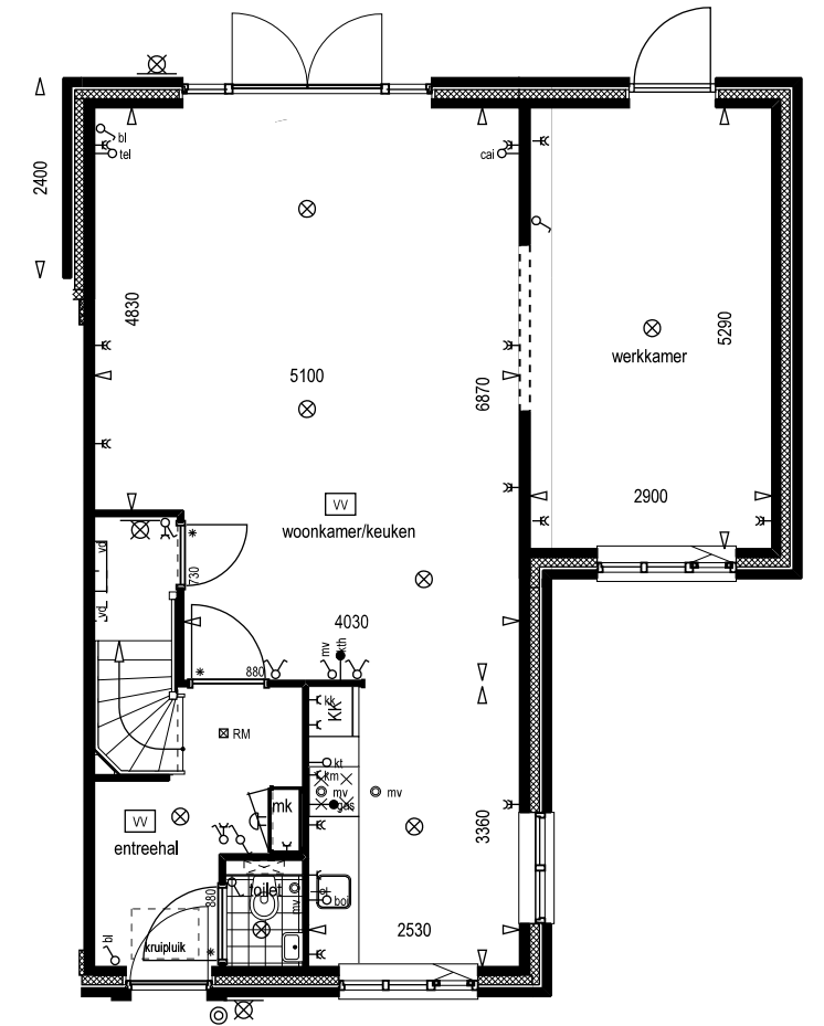
type A2/A3 optie uitbouw 2400 mm optie garage bij woonkamer i.c.m. uibouw optie openslaande deuren
