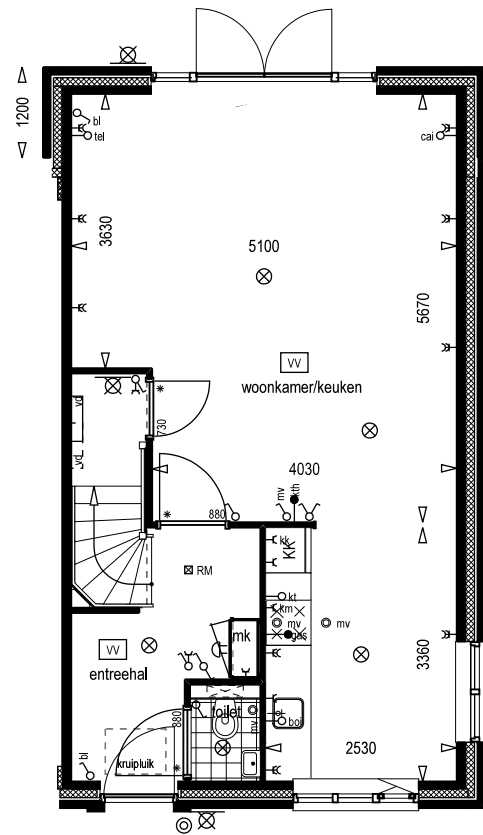
type A1 optie uitbouw 1200 mm optie openslaande deuren
