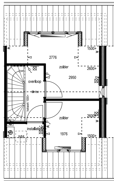
type A2 optie indeling zolder optie dakkapel voor optie dakkapel achter
