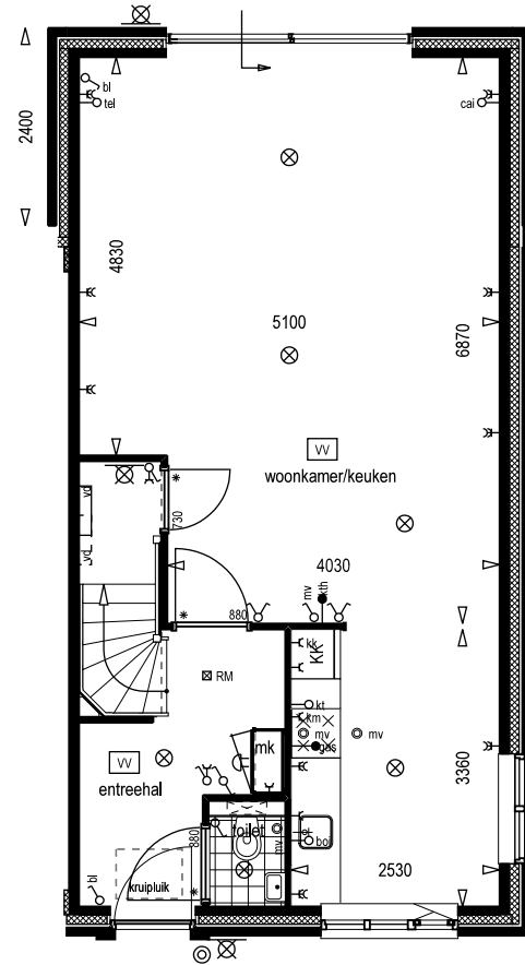
type A1 optie uitbouw 2400 mm
