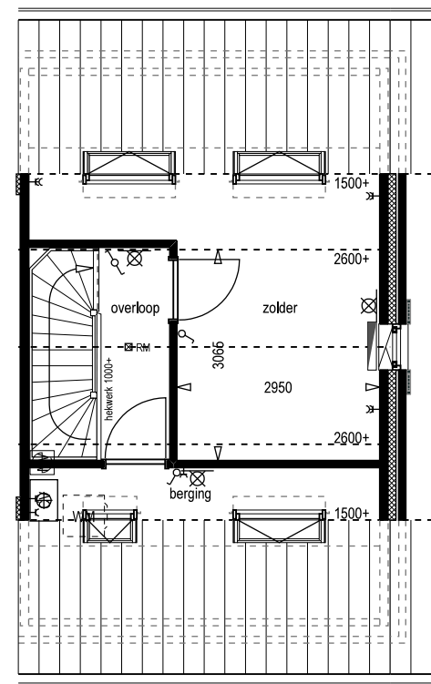
type A2 optie indeling zolder optie dakraam groot (3x) optie dakraam klein (1x)
