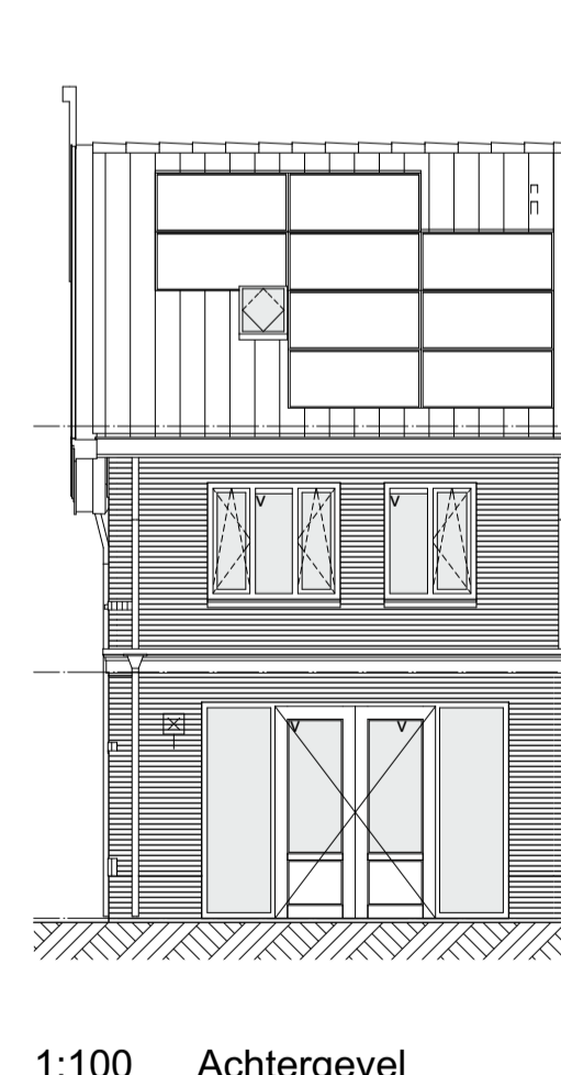
1:100 Achtergevel
