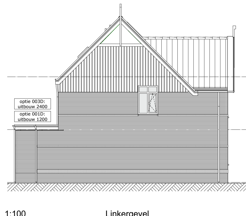
1:100 Linkergevel
