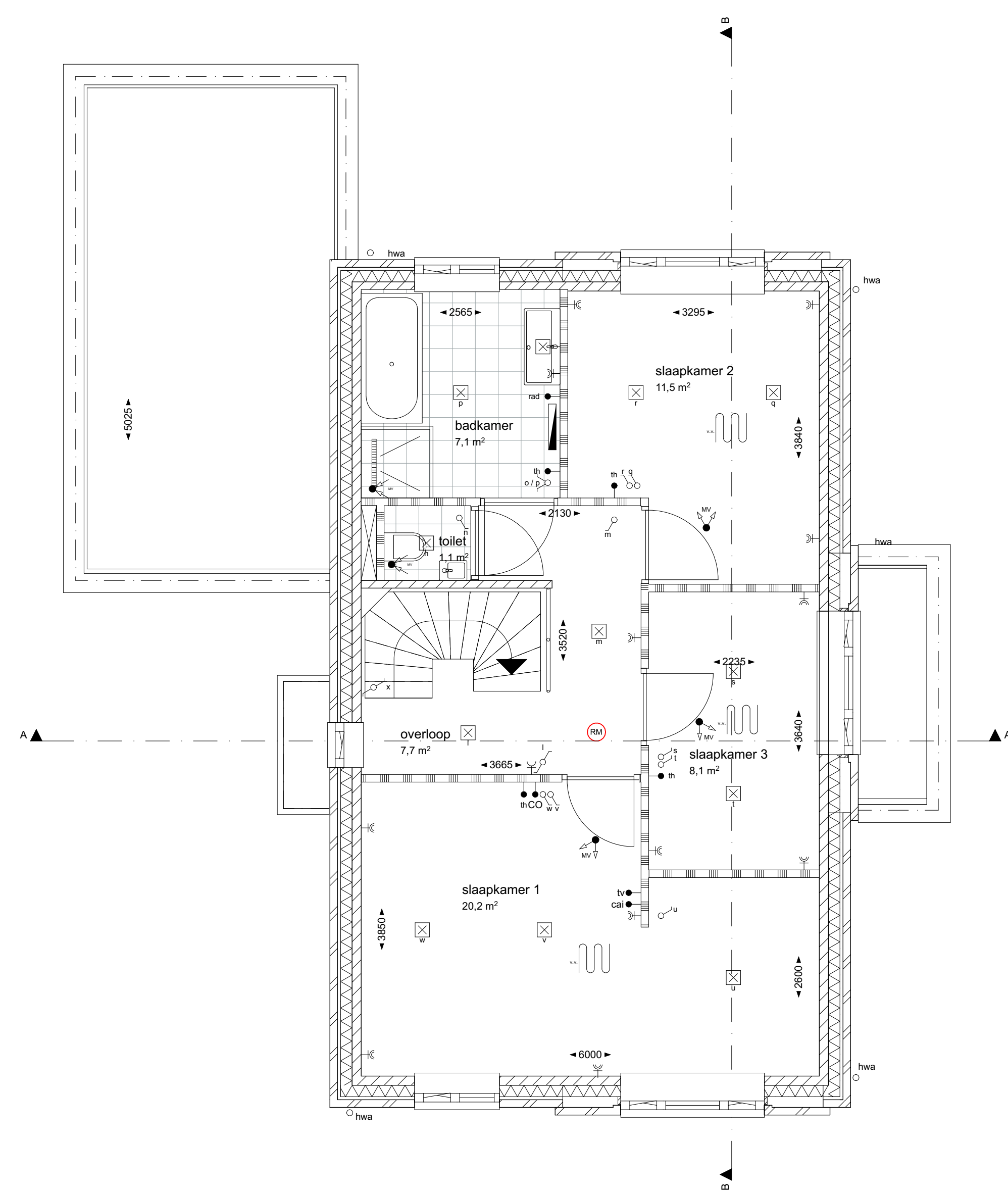
1:50 1e verdieping
