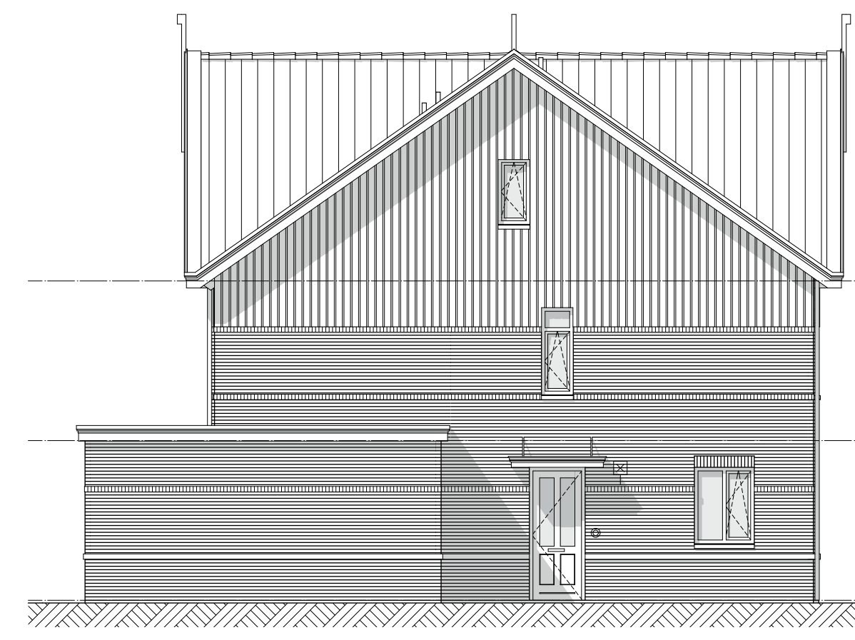
1:100 Linkergevel
