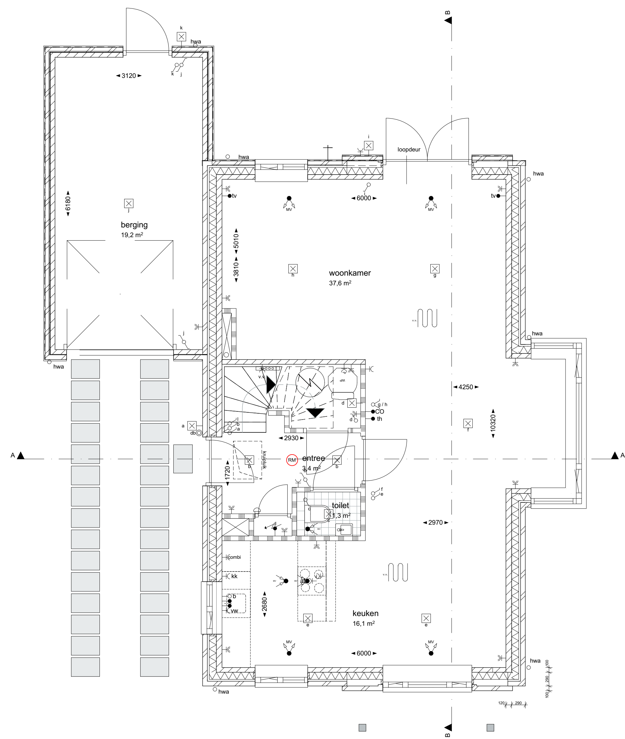
1:50 Begane grond
