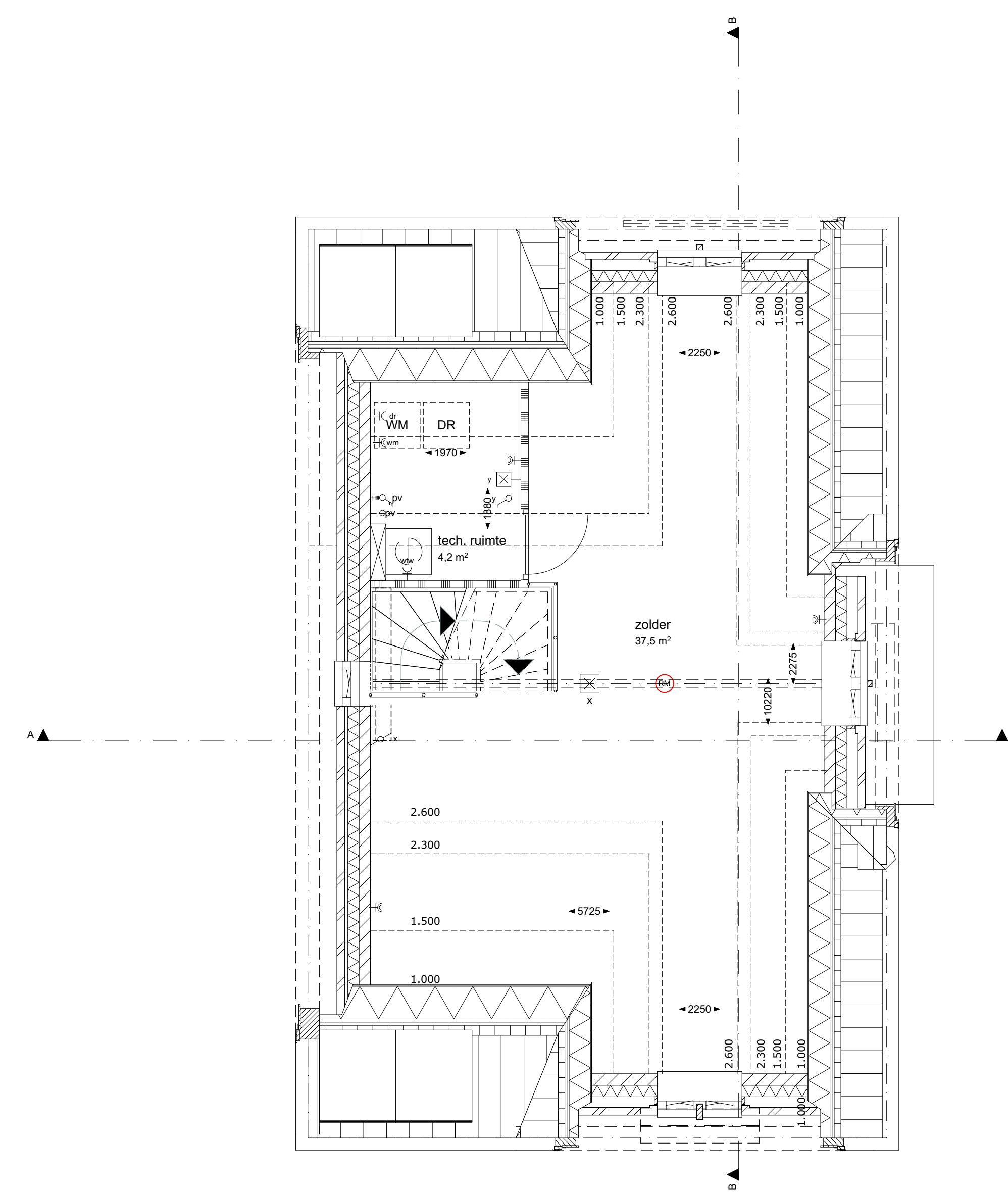
1:50 2e verdieping
