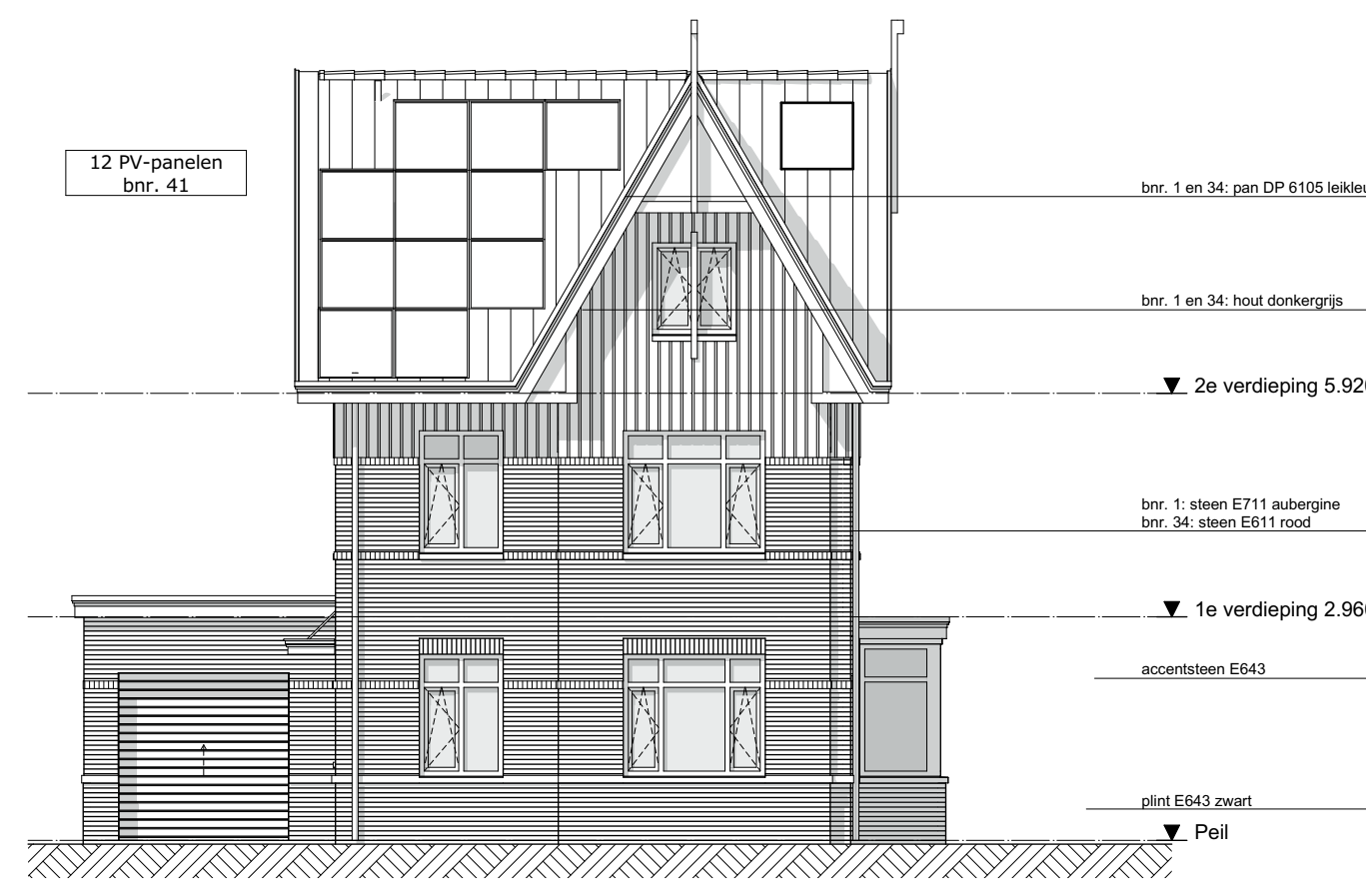
1:100 Voorgevel
