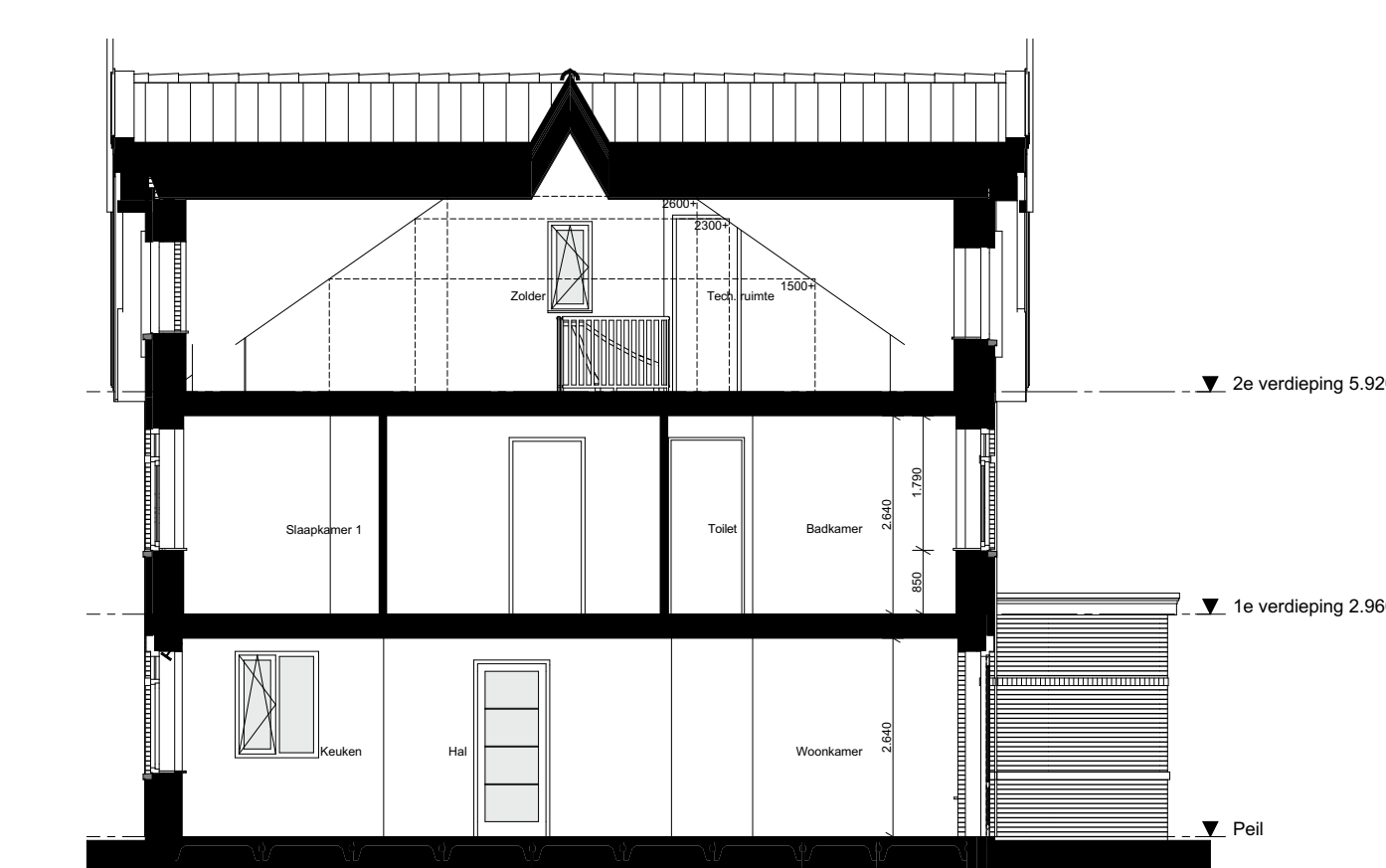
1:100 Doorsnede B-B
