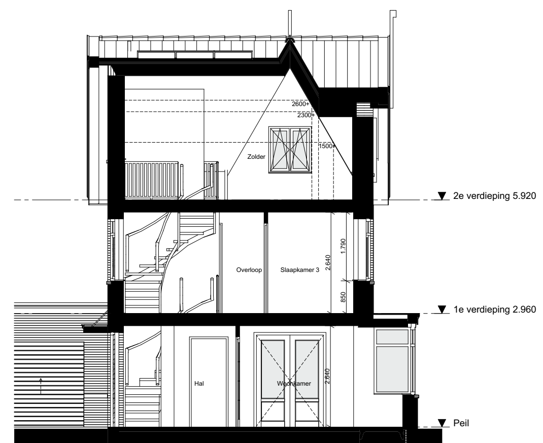
1:100 Doorsnede A-A
