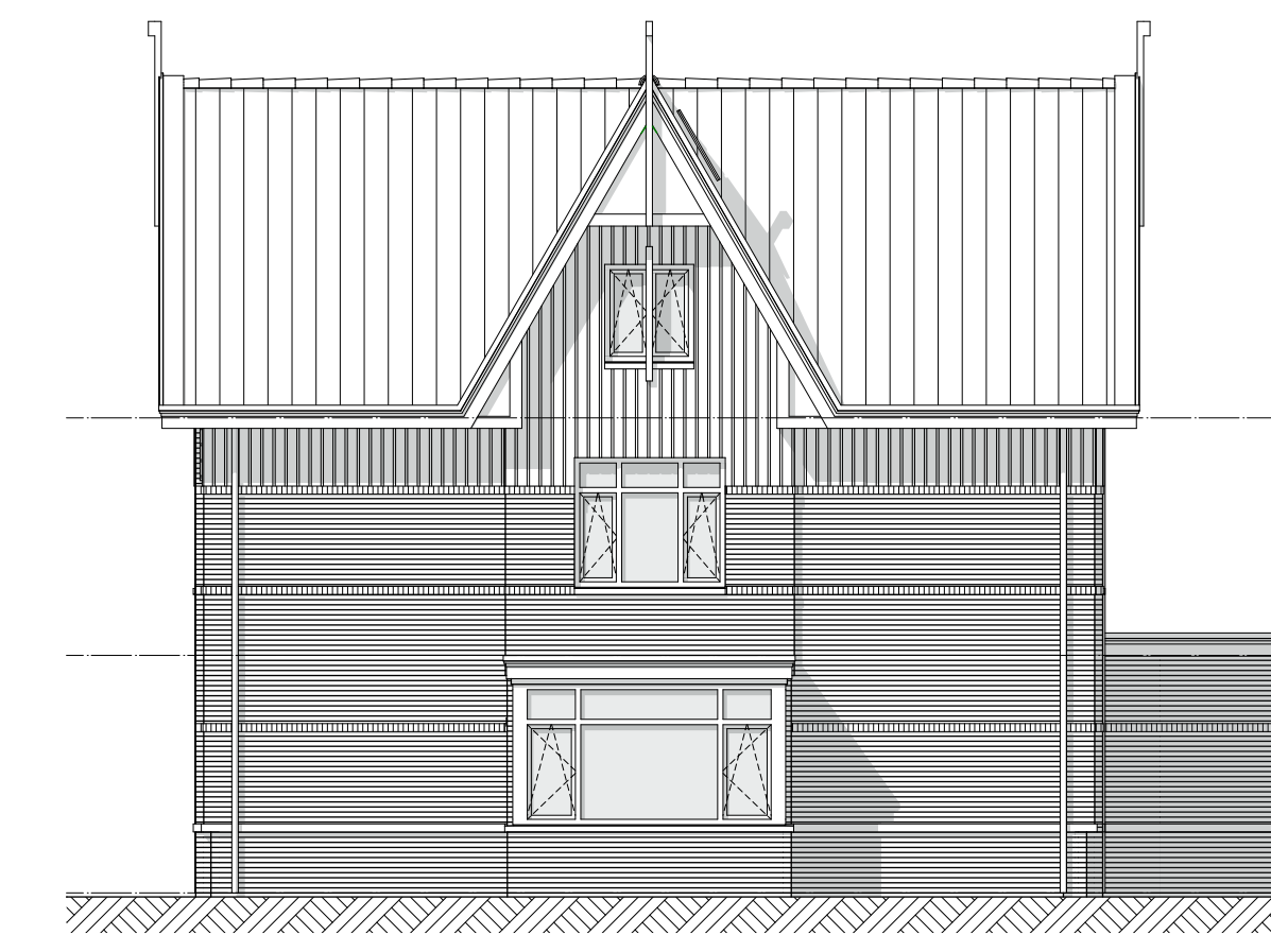
1:100 Rechtergevel
