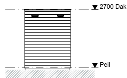
1:100 Zijgevel
