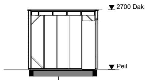
1:100 Doorsnede A-A
