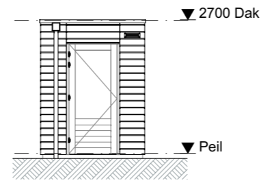
1:100 Voorgevel
