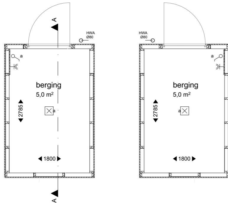
1:50 Begane grond
