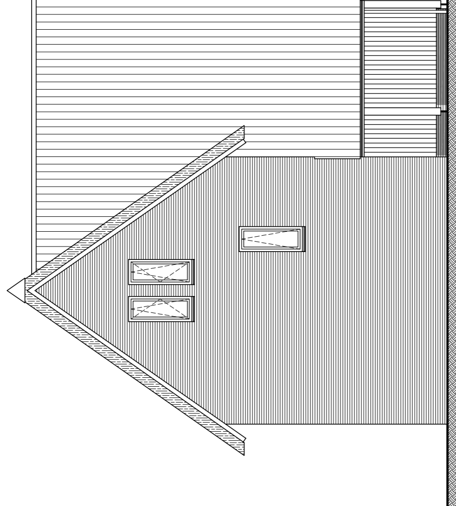
Rechterzijgevel schaal 1:100 bouwnummer : 66
