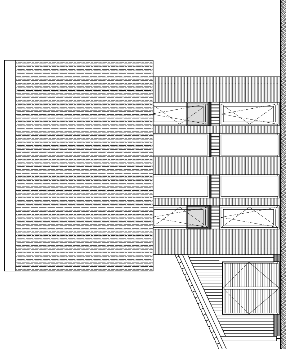
Voorgevel schaal 1:100 bouwnummer : 66
