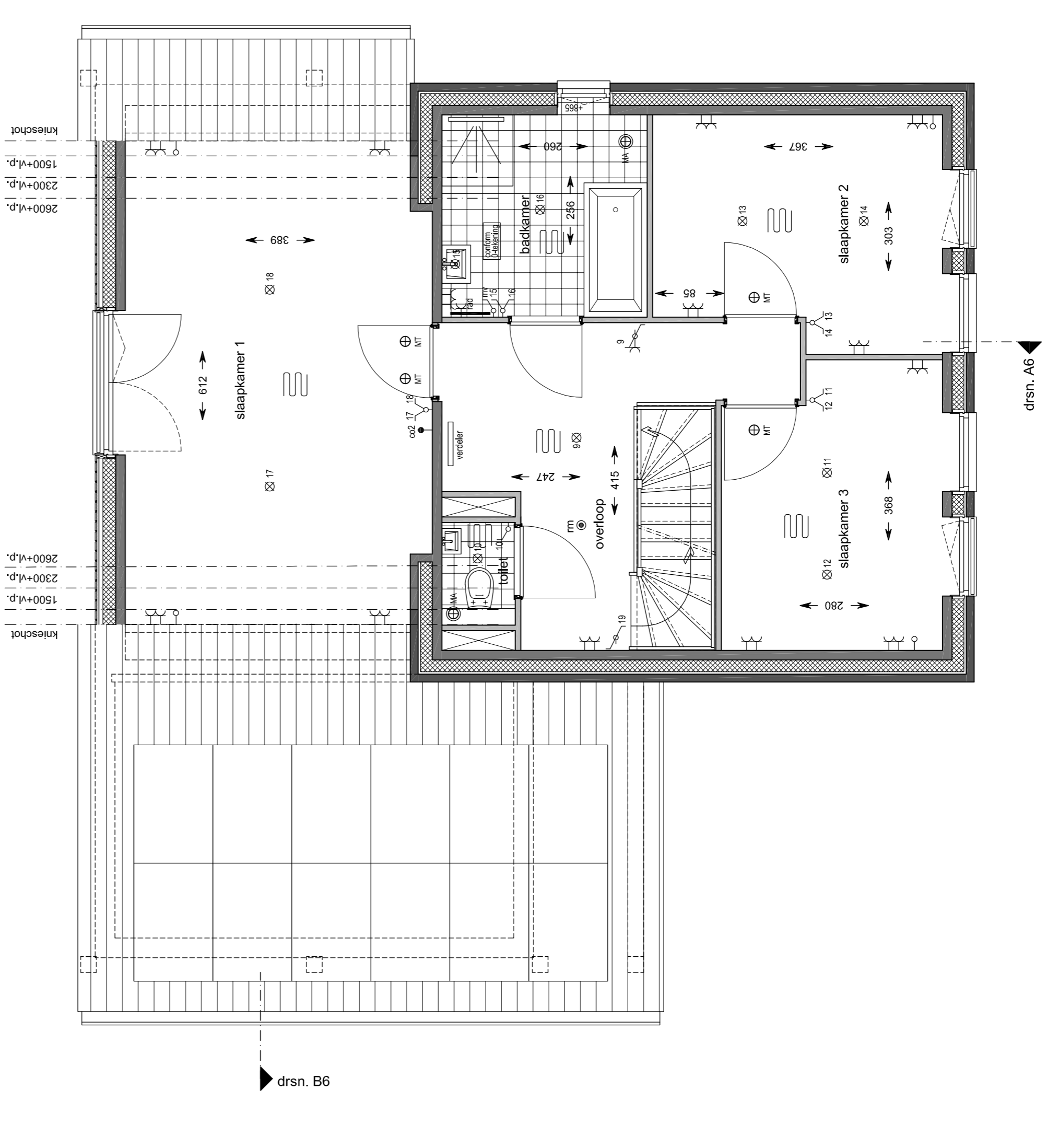
1e Verdieping schaal 1:50 bouwnummer : 66
