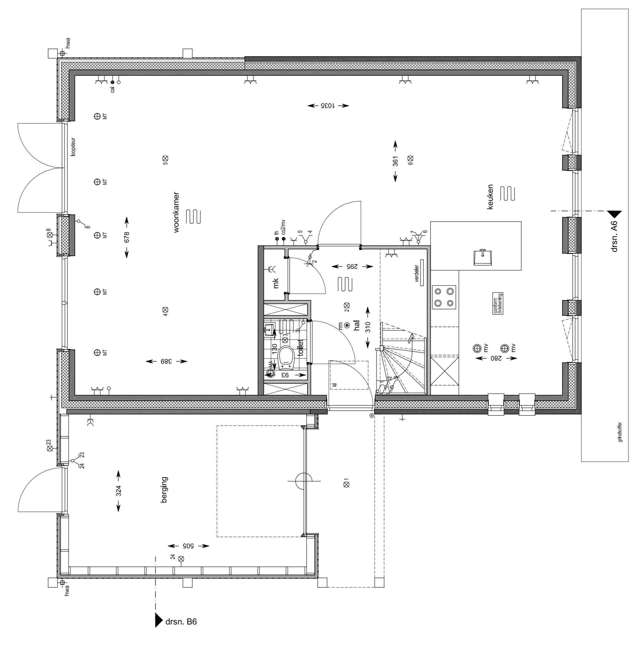
Begane grond schaal 1:50 bouwnummer : 66
