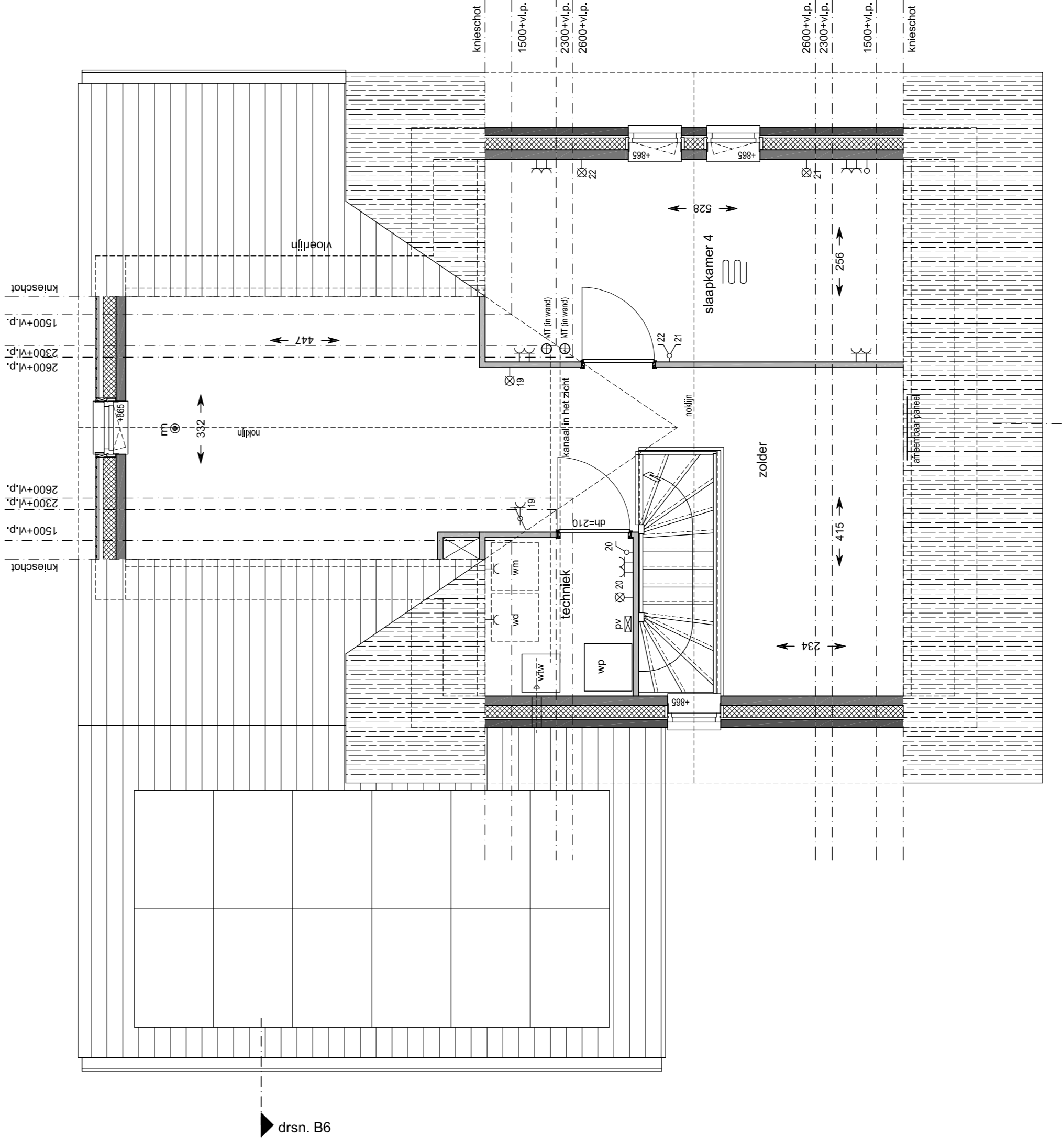
2e Verdieping schaal 1:50 bouwnummer : 66
