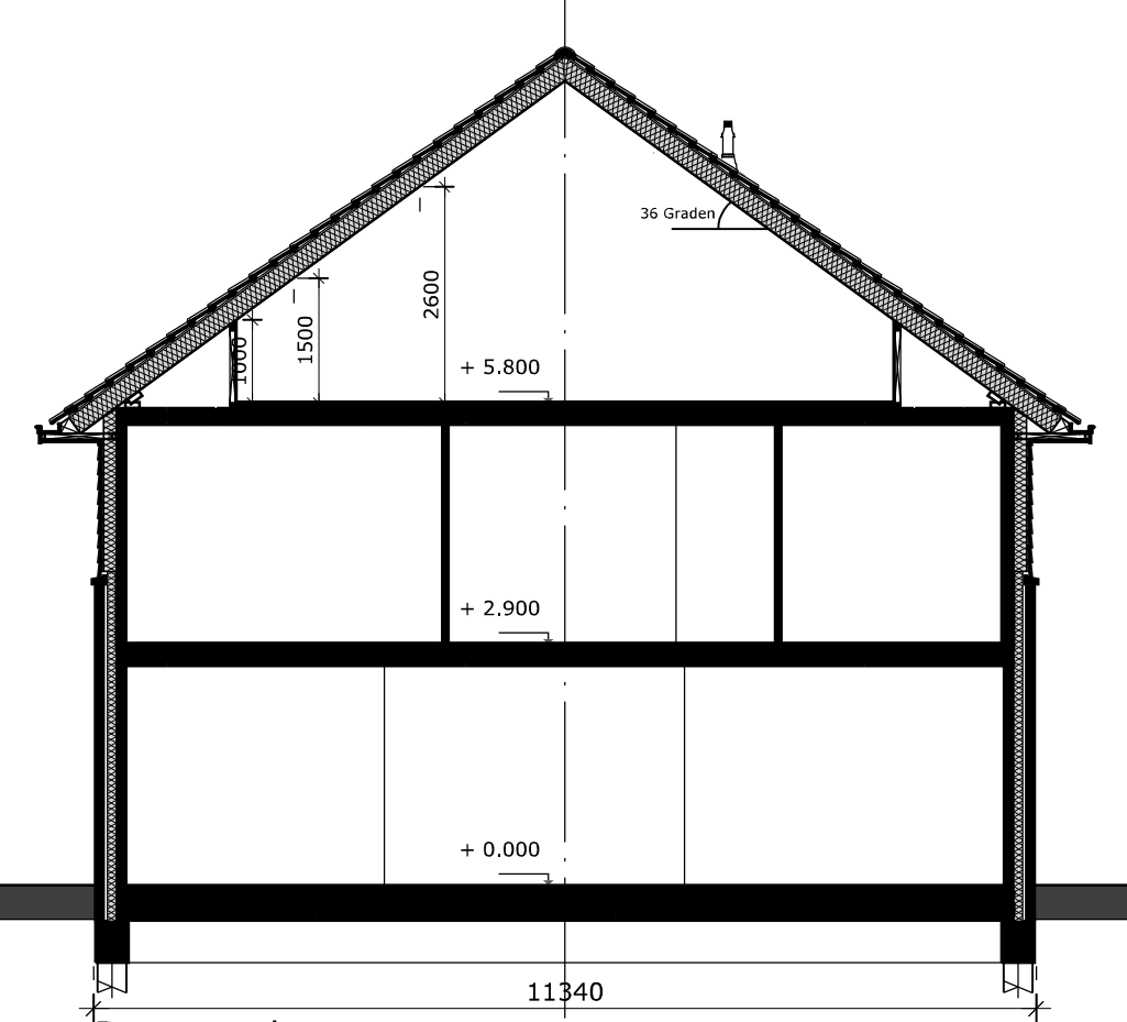
Doorsnede Principe doorsnede
