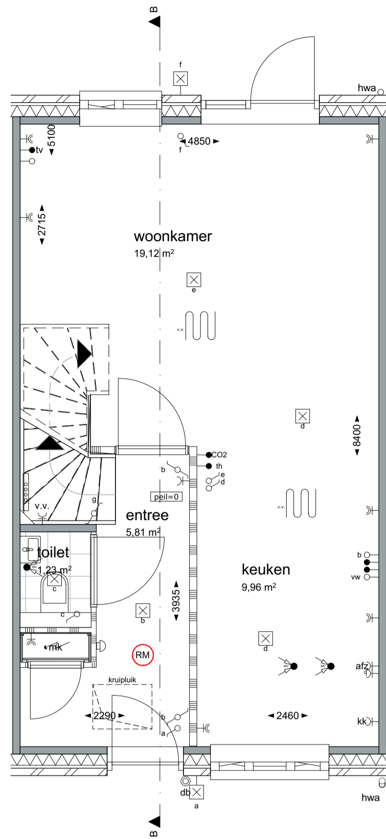
1:50 Begane grond
