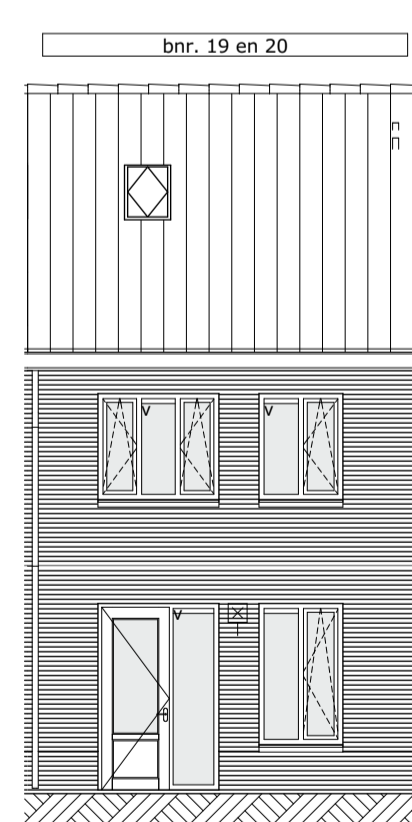
1:100 Achtergevel
