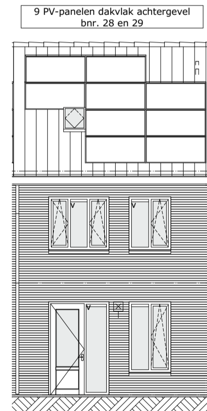
1:100 Achtergevel
