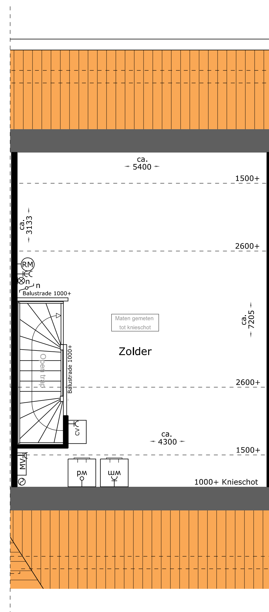
2e Verdieping
