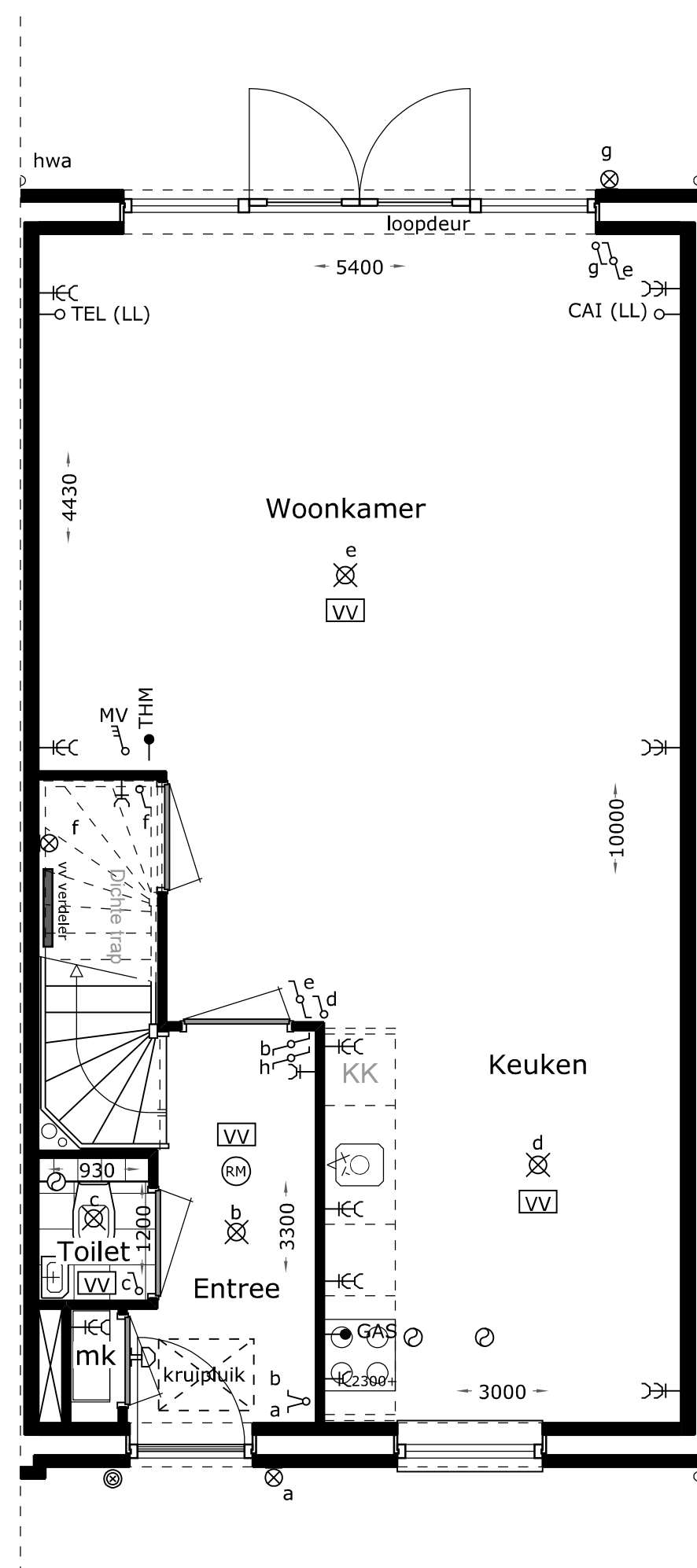
Begane grond
