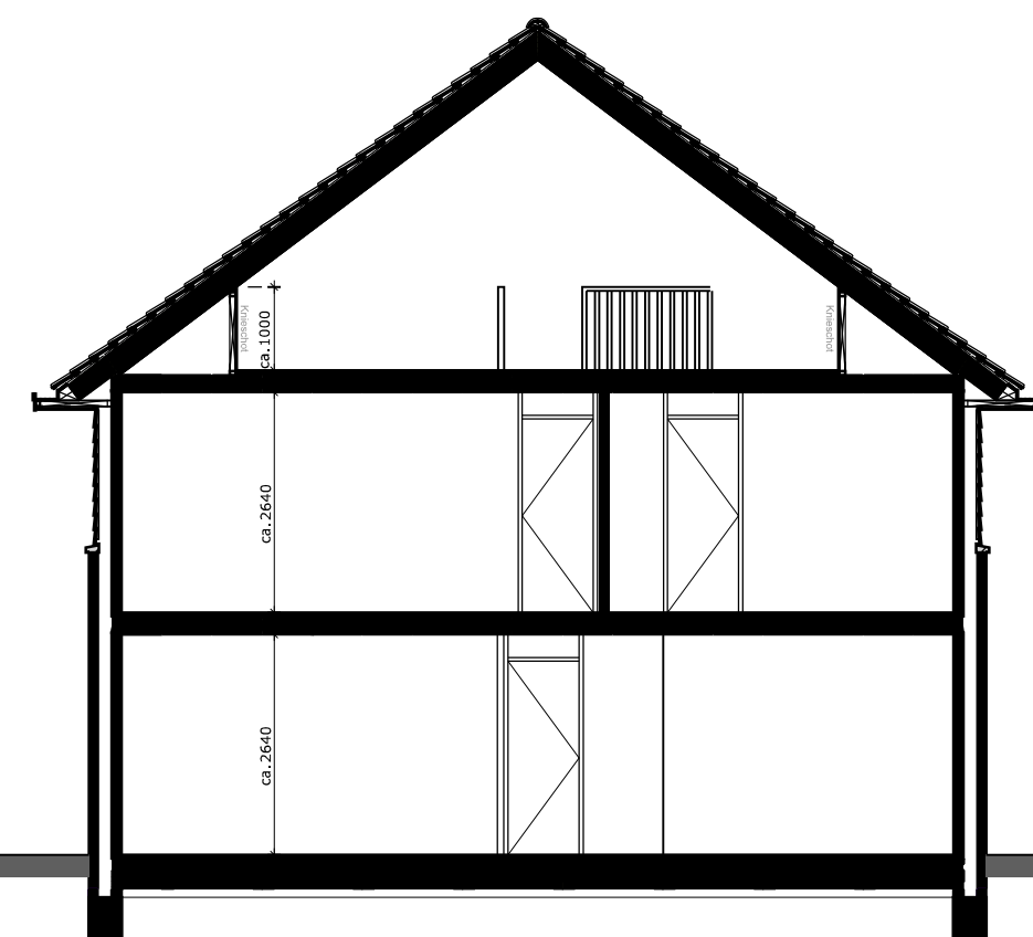
Principe doorsnede
