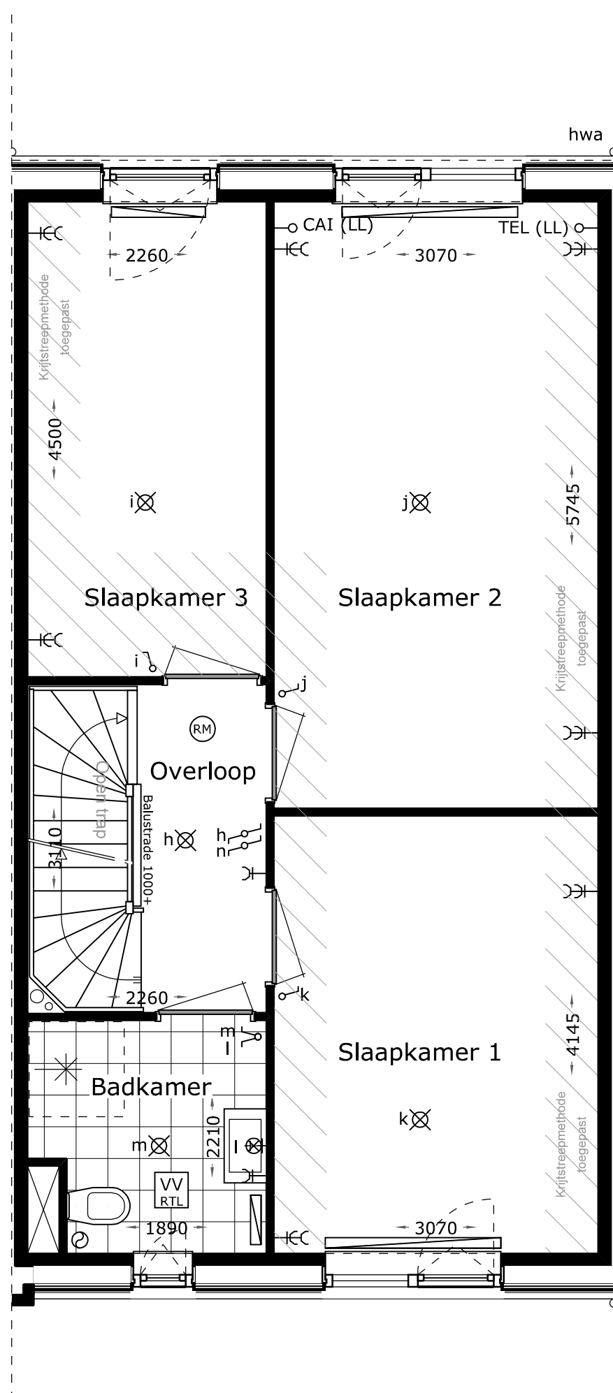
1e Verdieping
