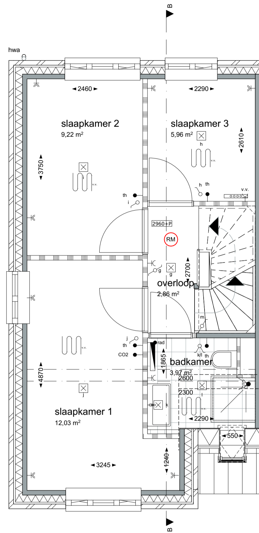
1:50 1e verdieping
