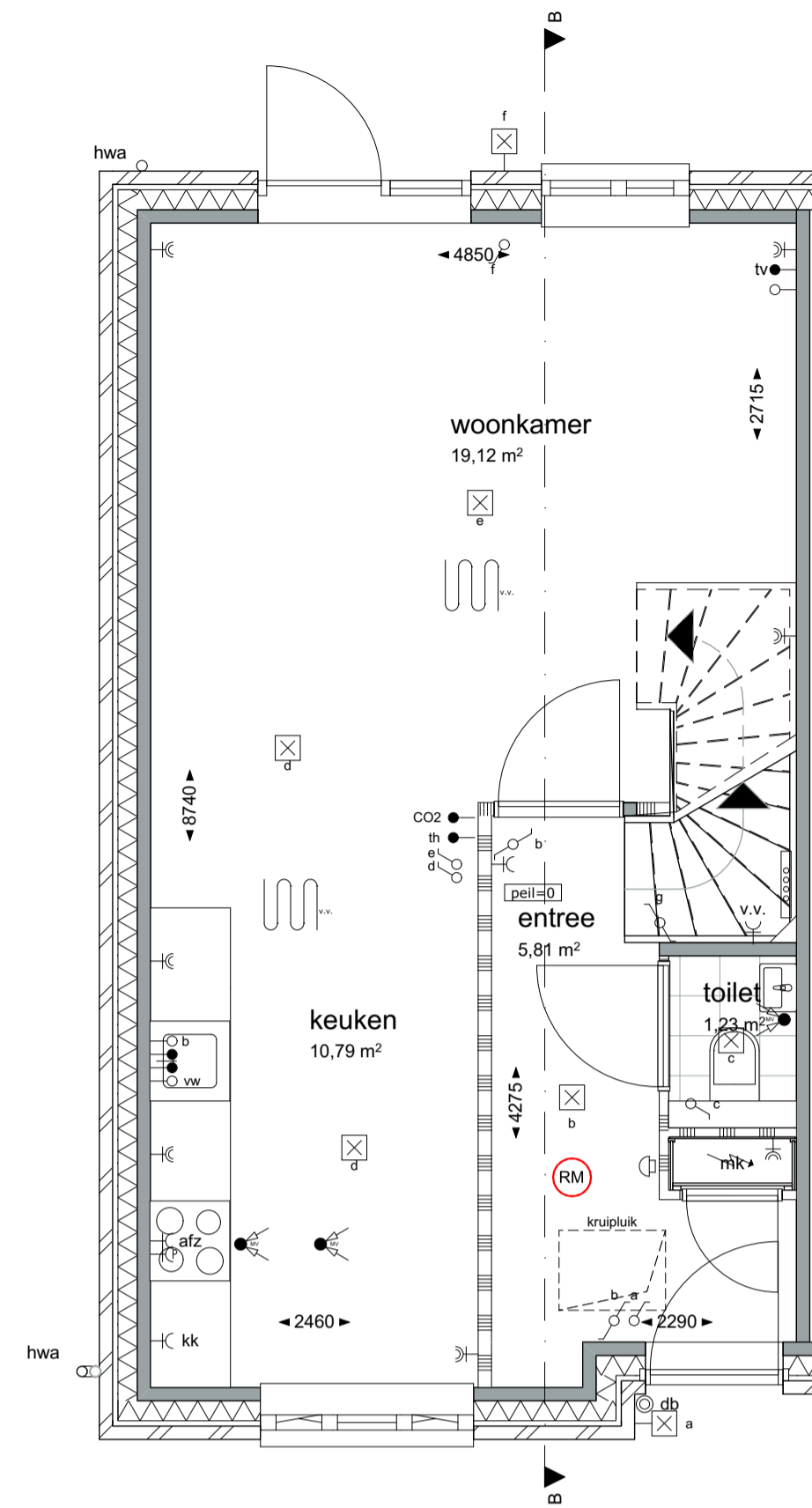
1:50 Begane grond
