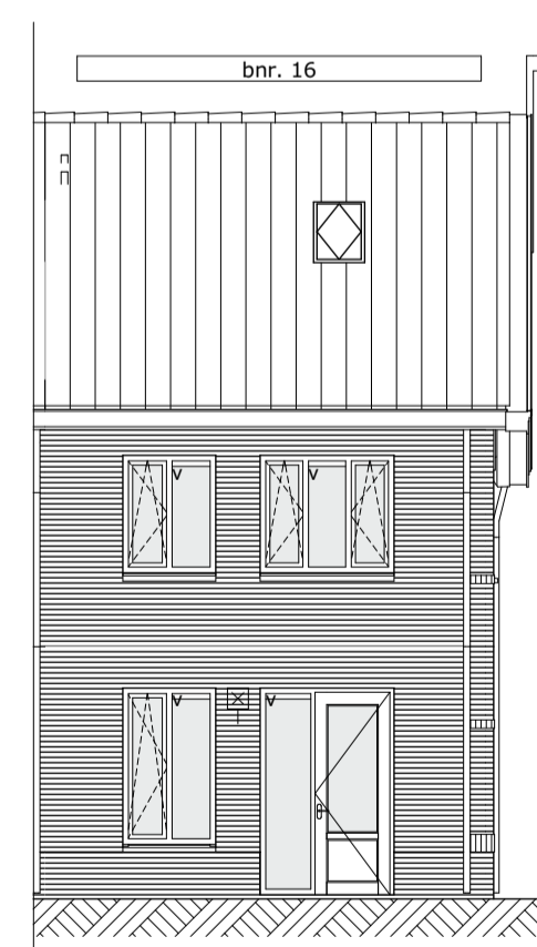
1:100 Achtergevel
