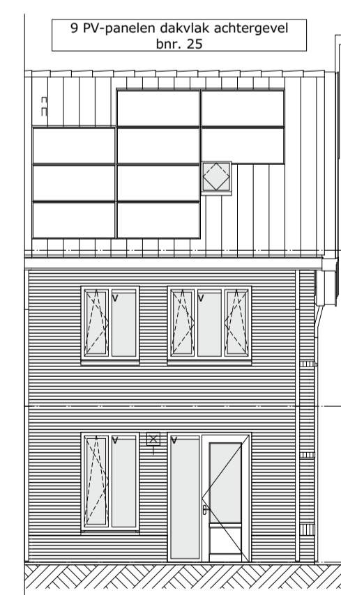
1:100 Achtergevel
