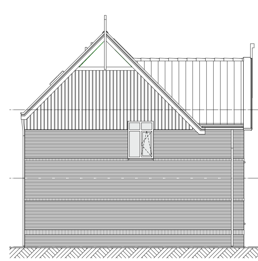
1:100 Linkergevel
