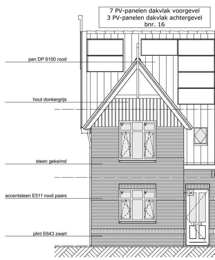
1:100 Voorgevel
