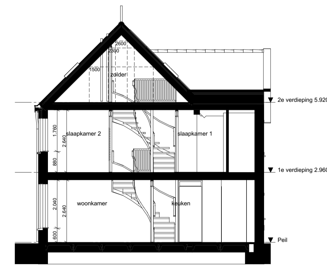
1:100 Doorsnede B-B A1E
