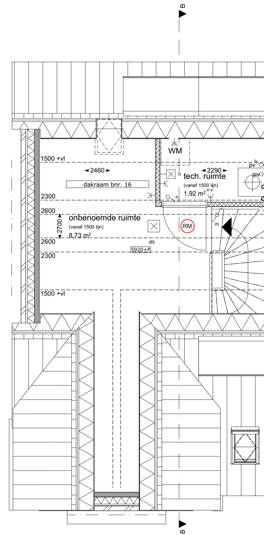
1:50 2e verdieping
