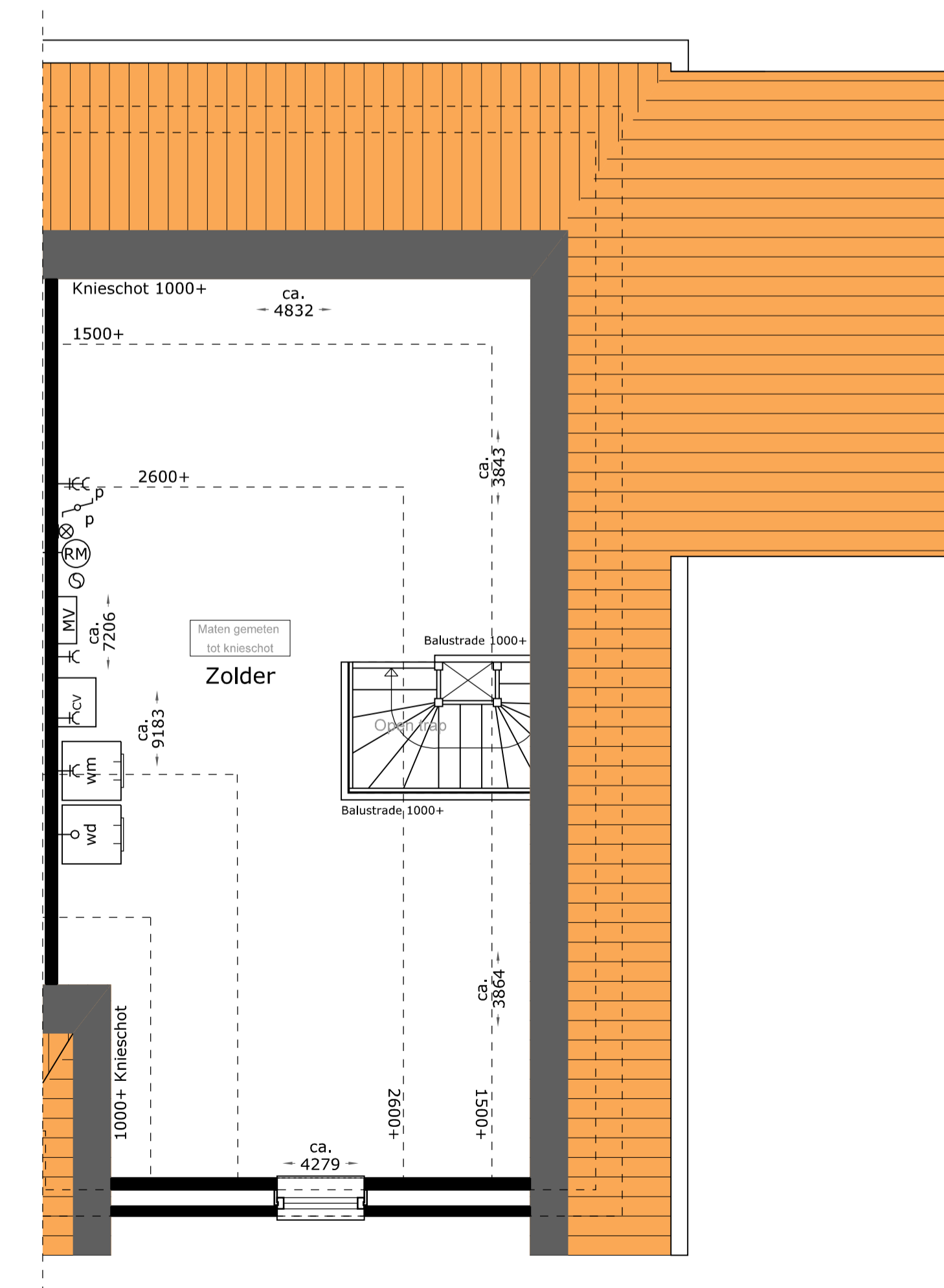
2e Verdieping
