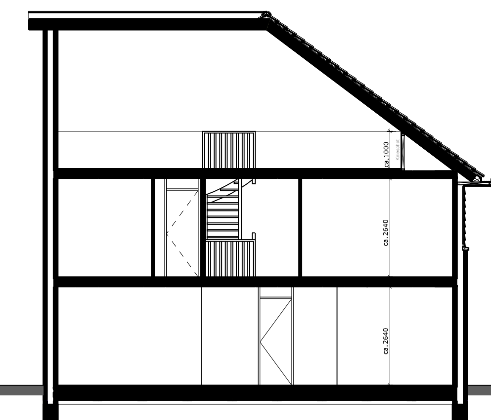
Principe doorsnede
