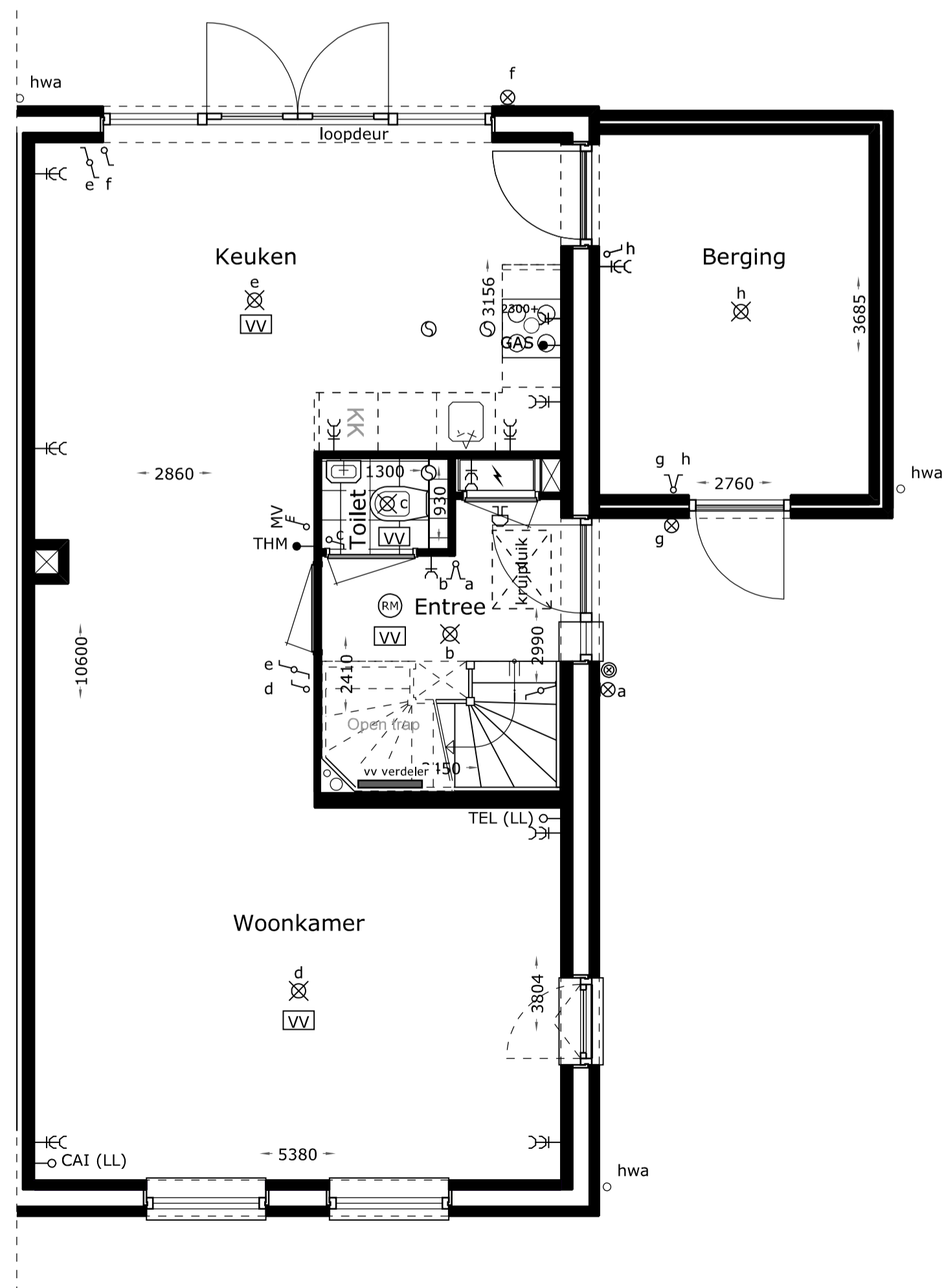
Begane grond
