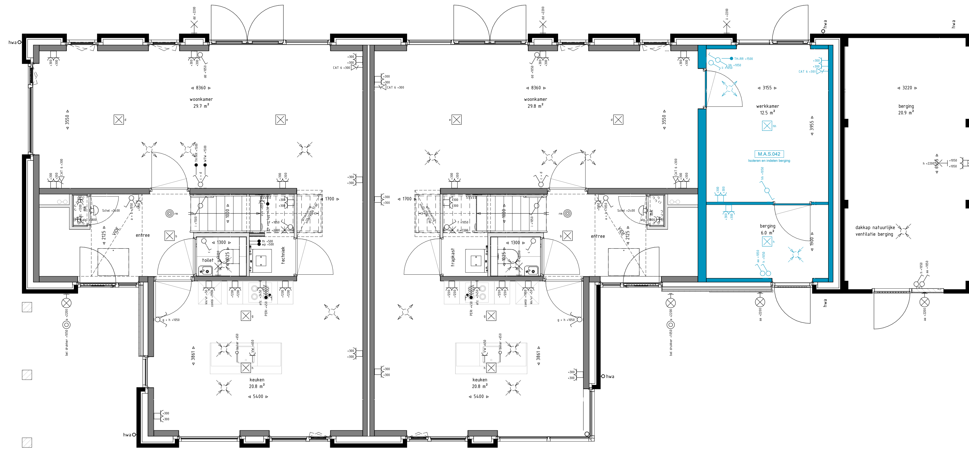
Begane grond - geïsoleerde berging indeling 1:50
