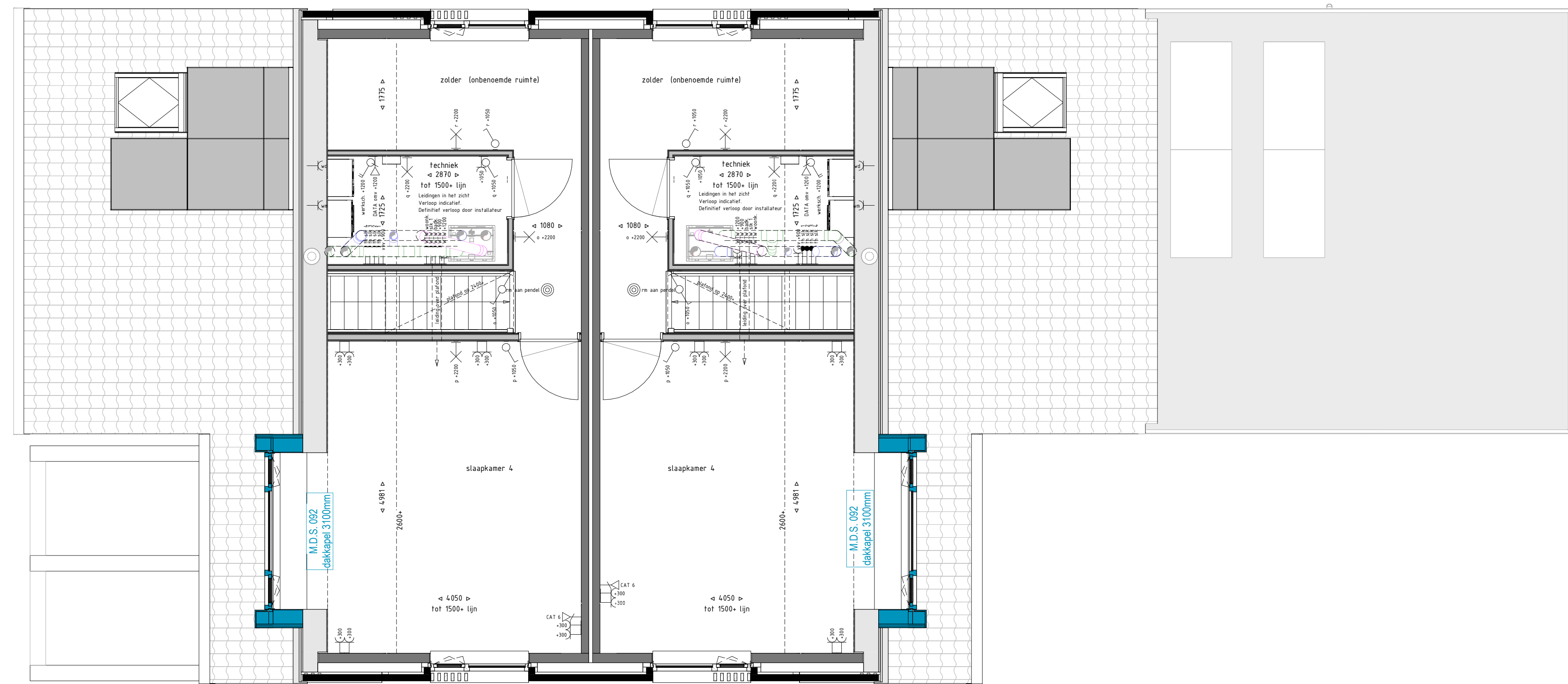
Tweede verdieping - dakkapel 1:50
