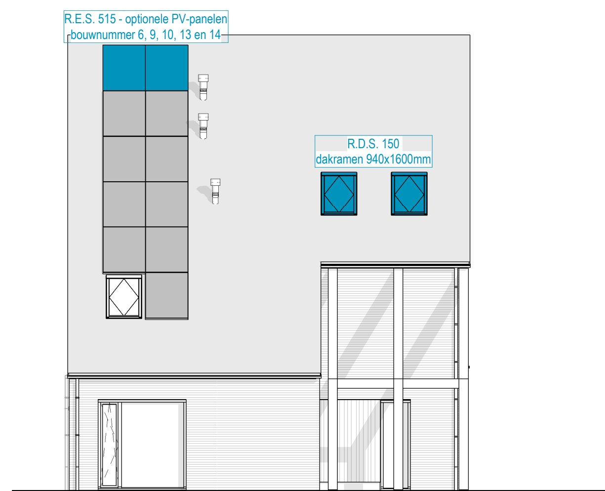
Linker zijgevel - PV panelen en dakraam 1:100
