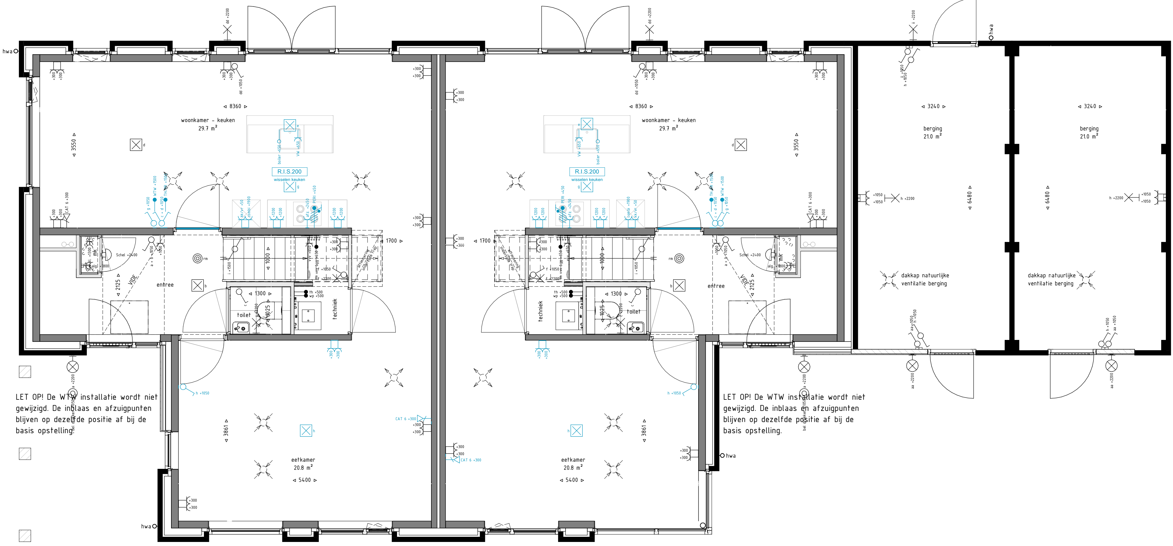
Begane grond - keuken 1:50
