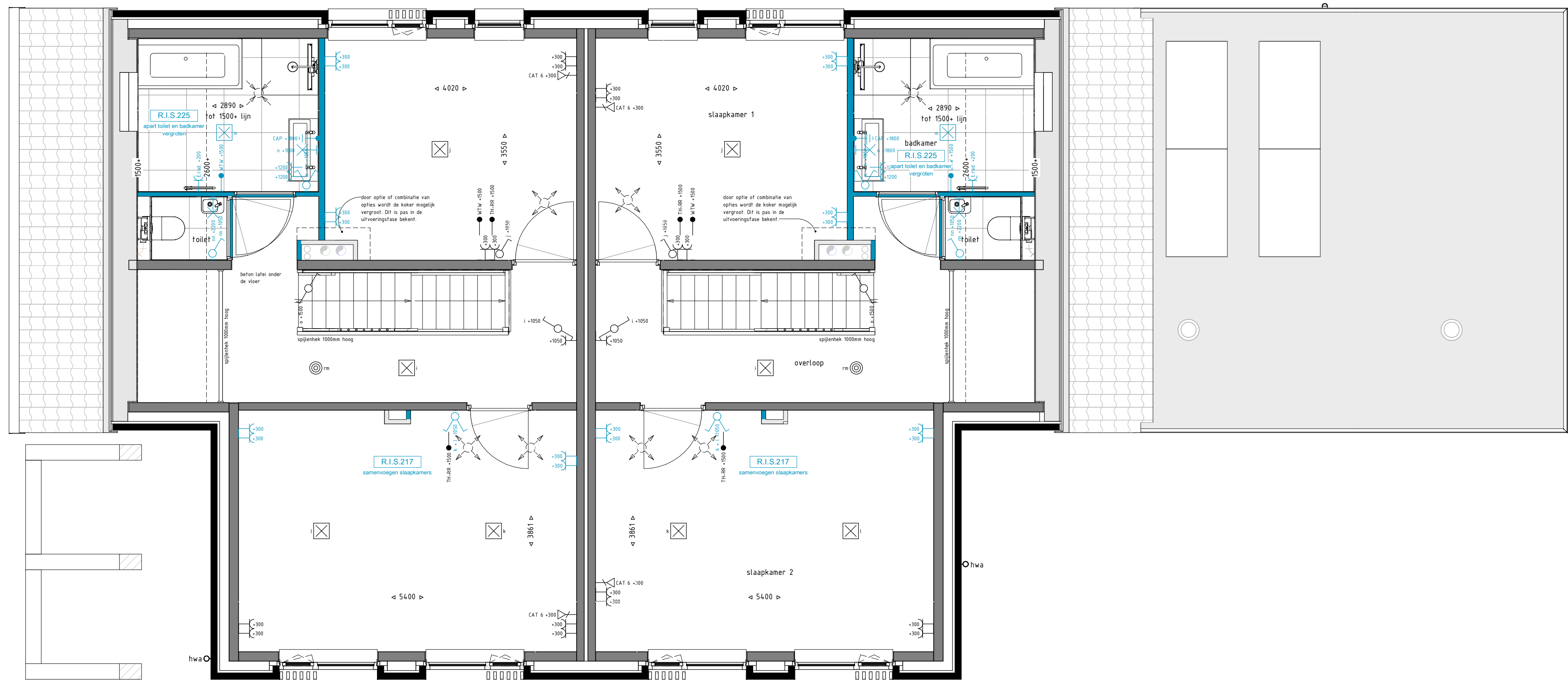
Eerste verdieping - toilet + badkamer apart en slaapkamers samenvoegen 1:50
