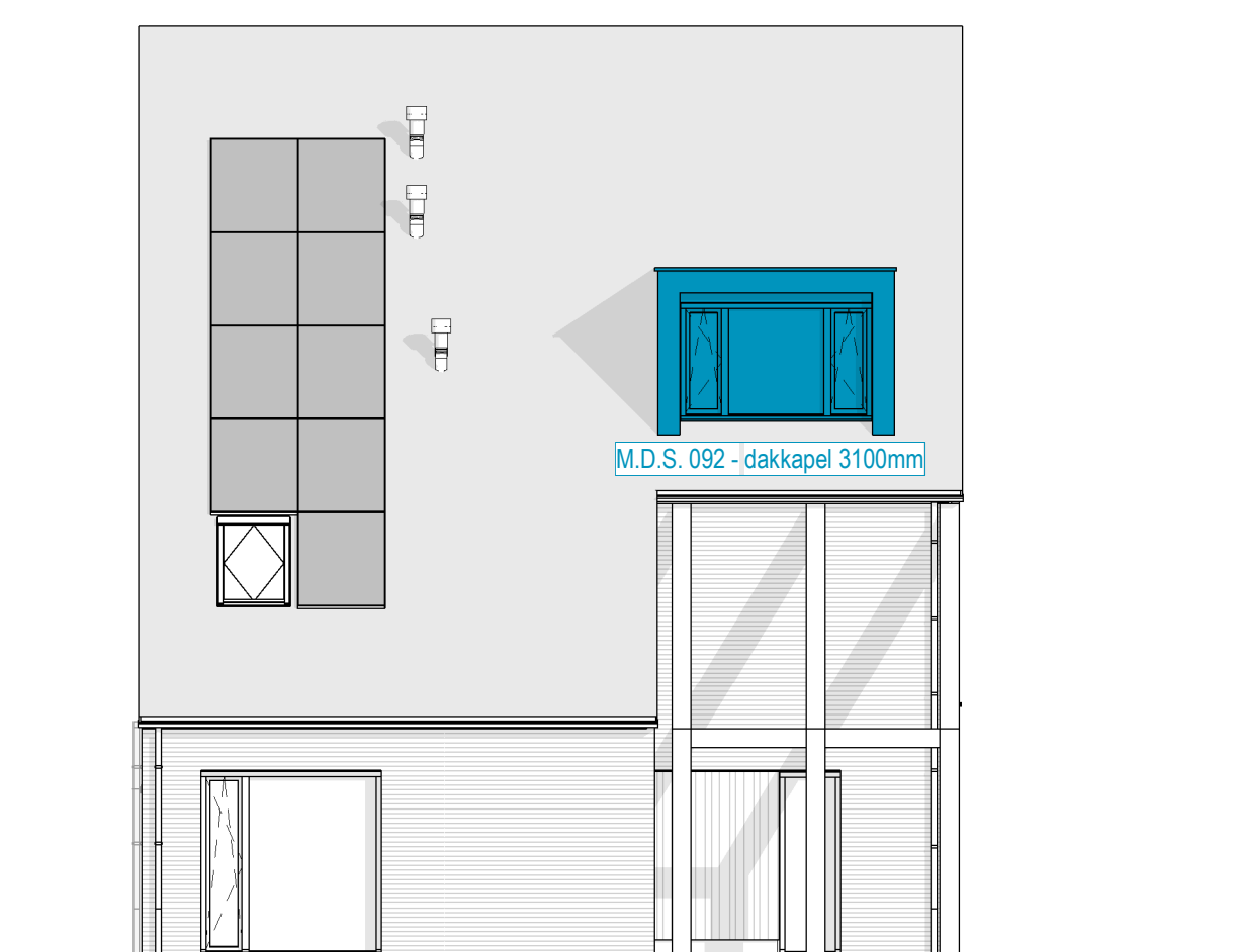
Linker zijgevel - dakkapel 1:100
