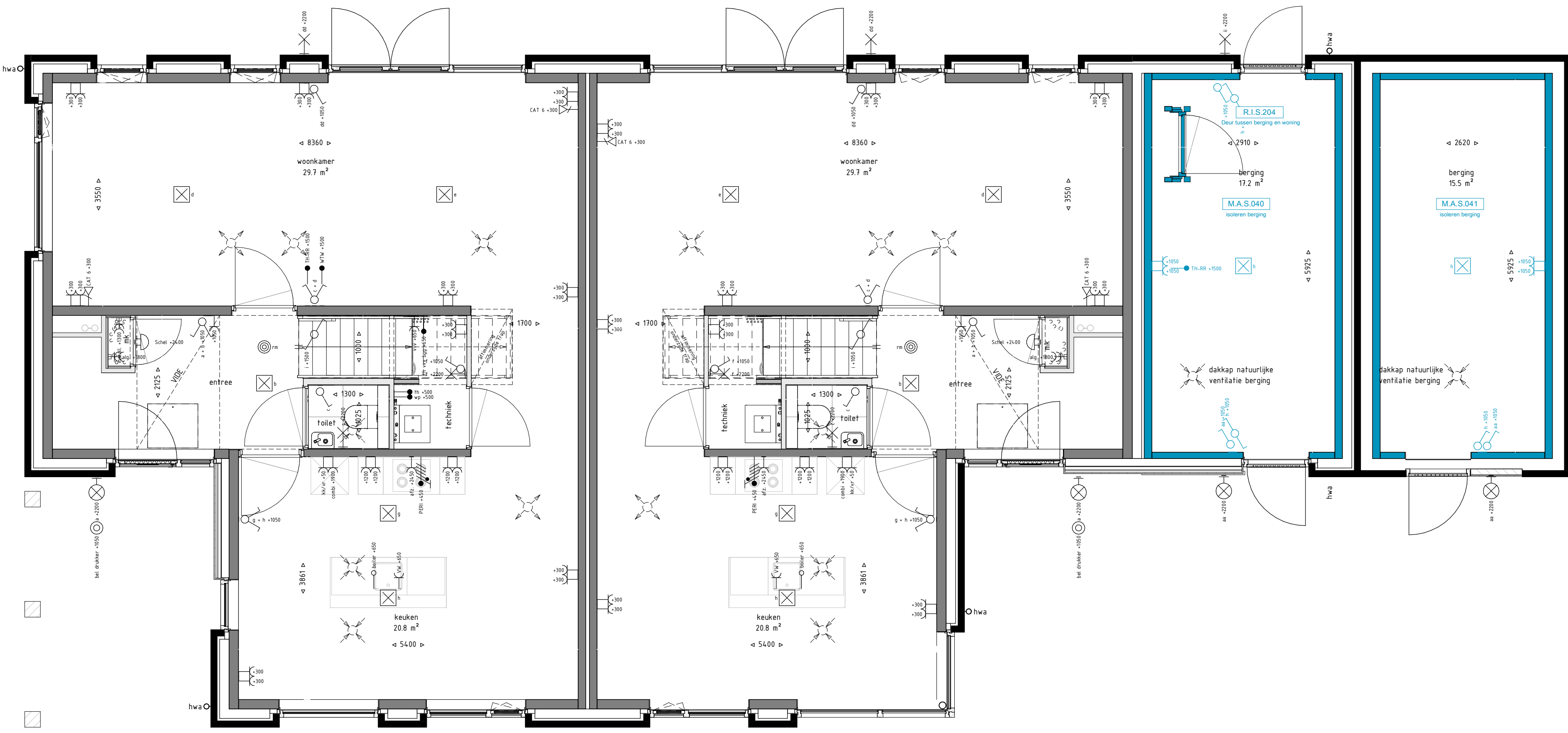
Begane grond - geïsoleerde berging 1:50
