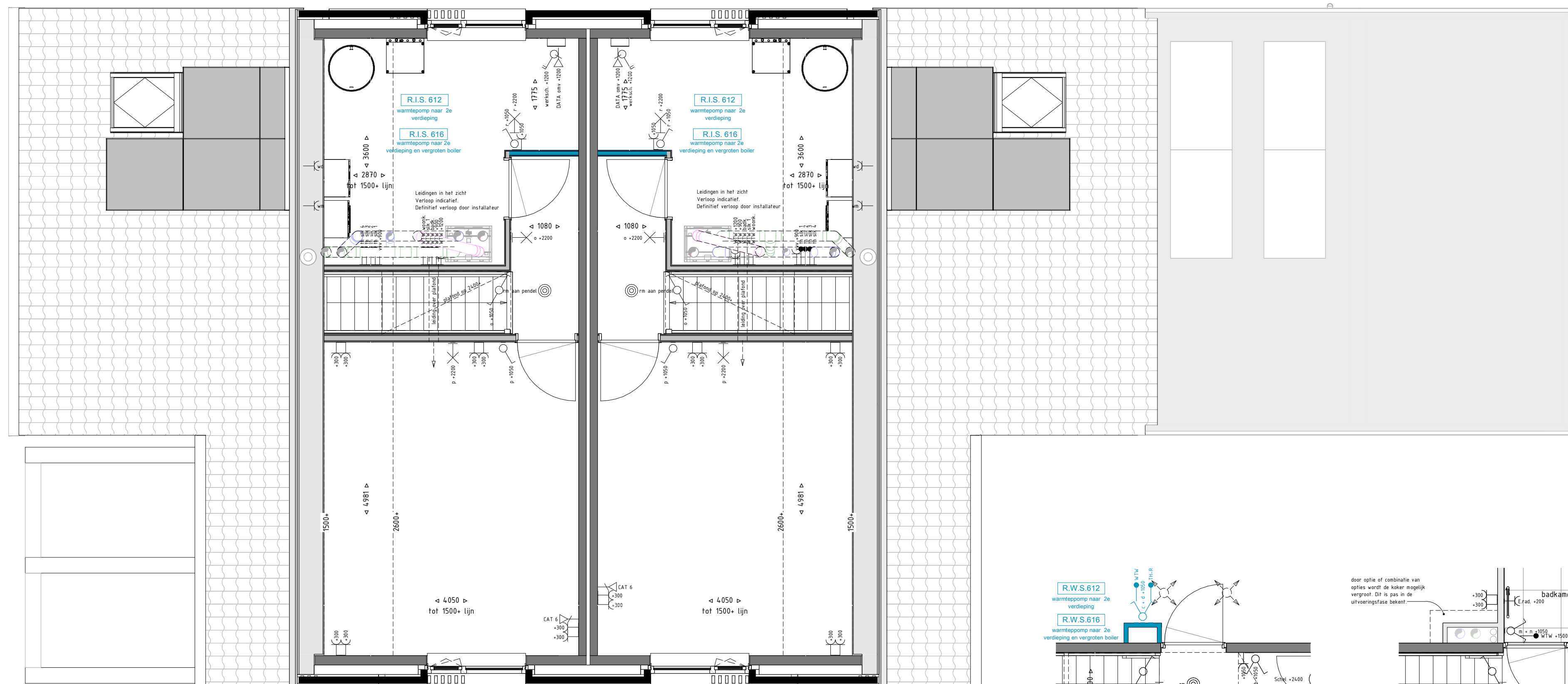
Tweede verdieping - boiler 1:50
