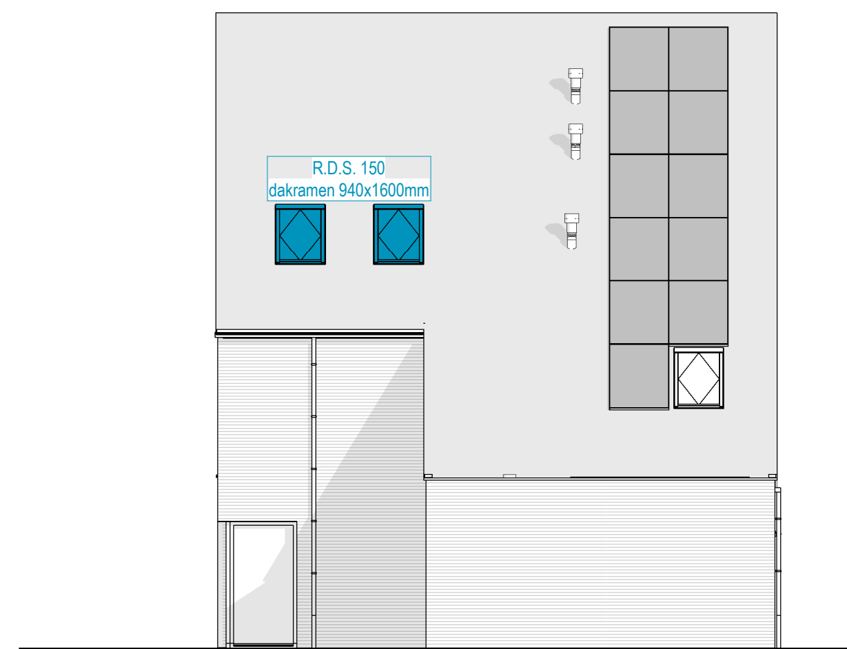
Rechter zijgevel - dakraam 1:100
