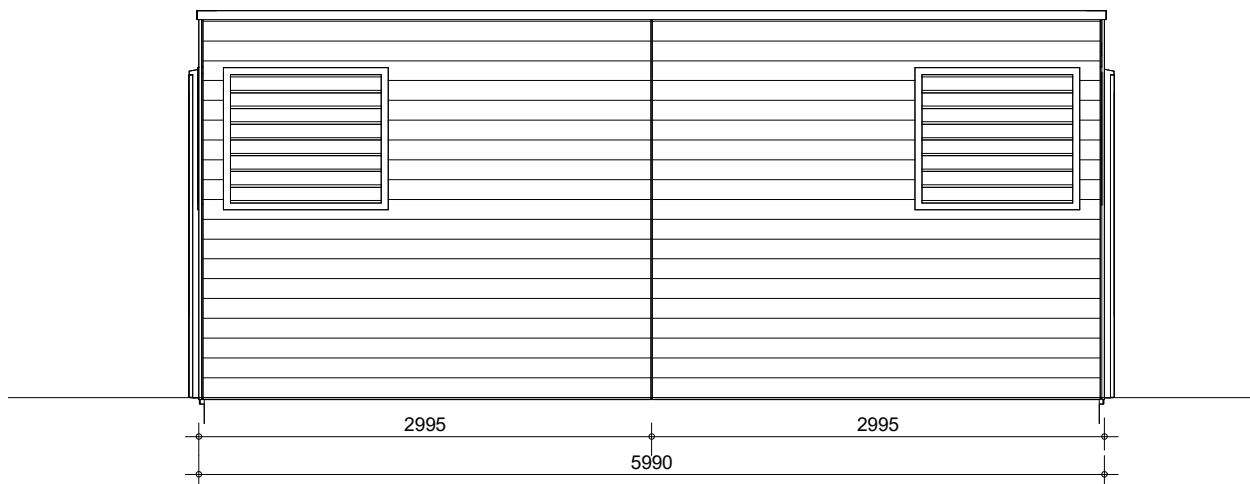
Gevel achterzijde
