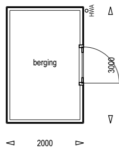
plattegrond enkele berging
