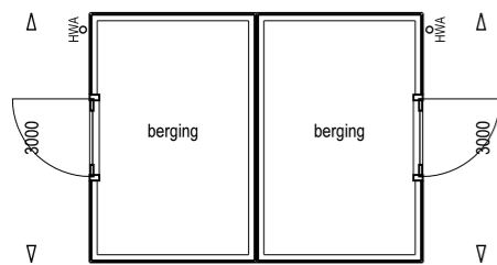
plattegrond dubbele berging
