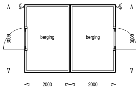
plattegrond dubbele berging
