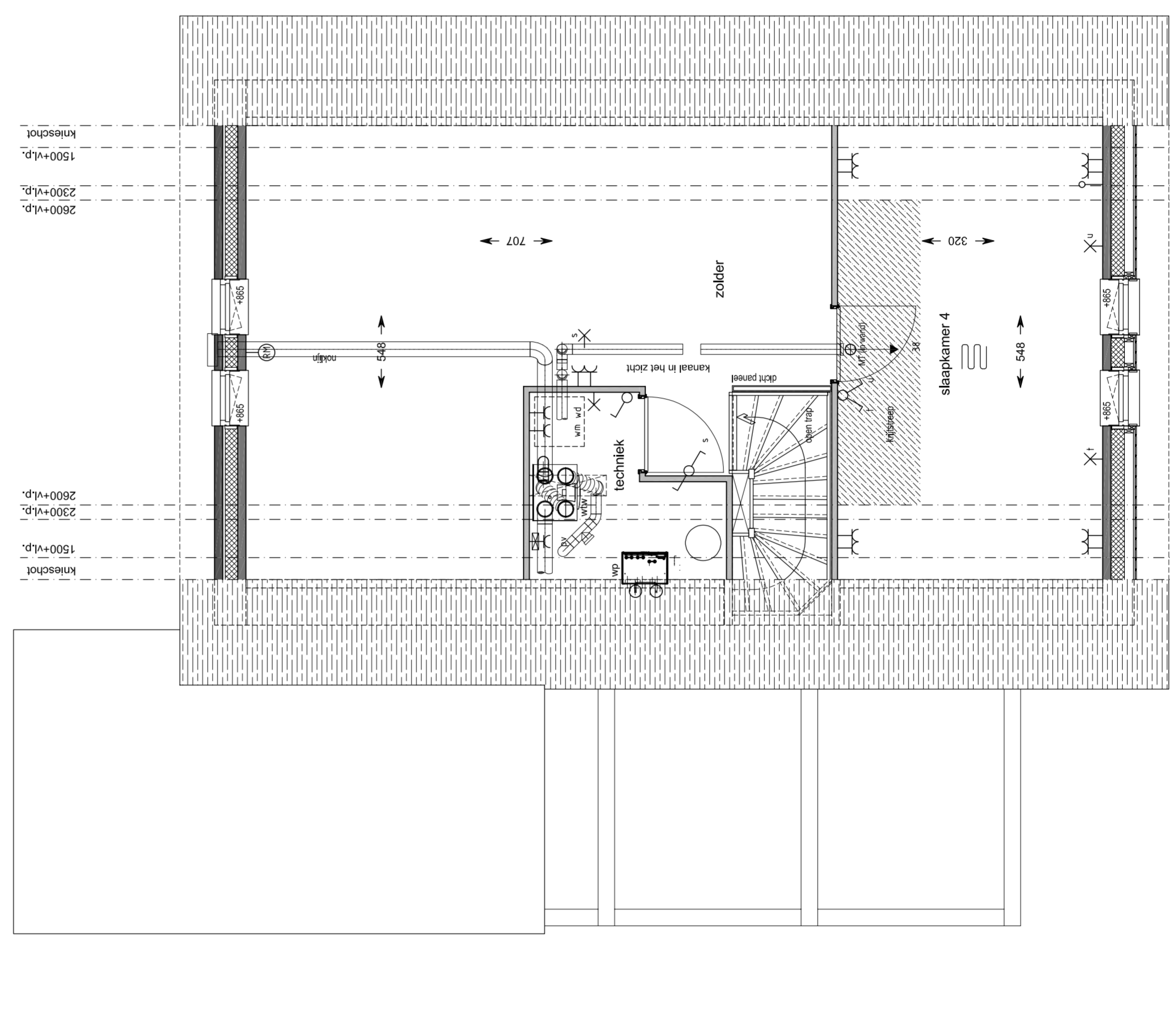
2e Verdieping schaal 1:50 bouwnummer : 27
