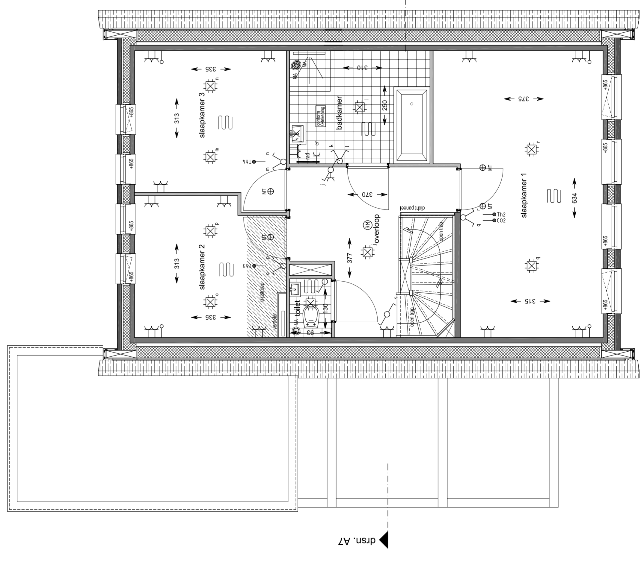
1e Verdieping schaal 1:50 bouwnummer : 27
