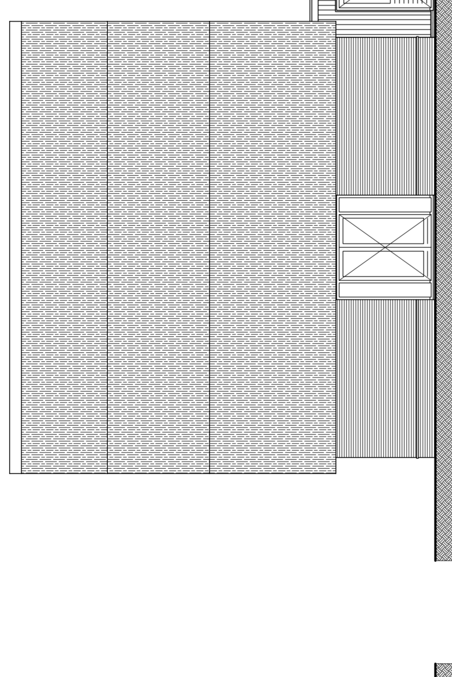
Rechterzijgevel schaal 1:100 bouwnummer : 27
