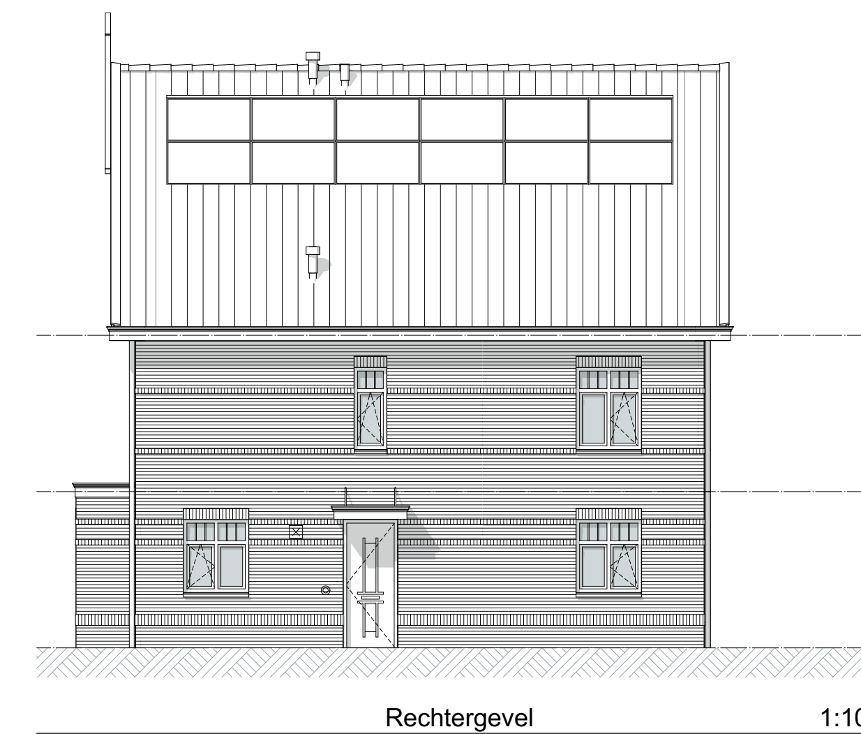
Rechtergevel 1:100
