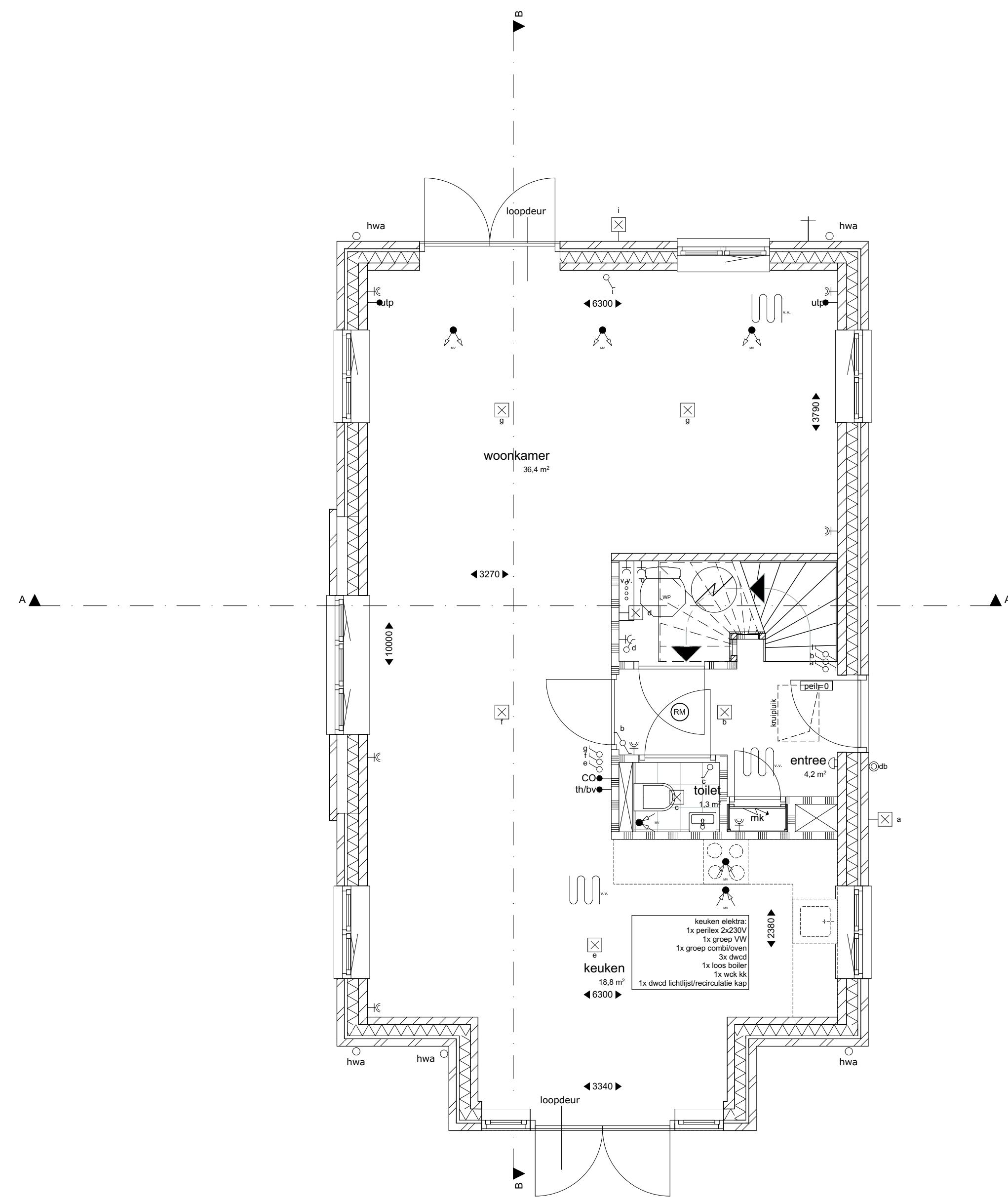
1:50 Begane grond
