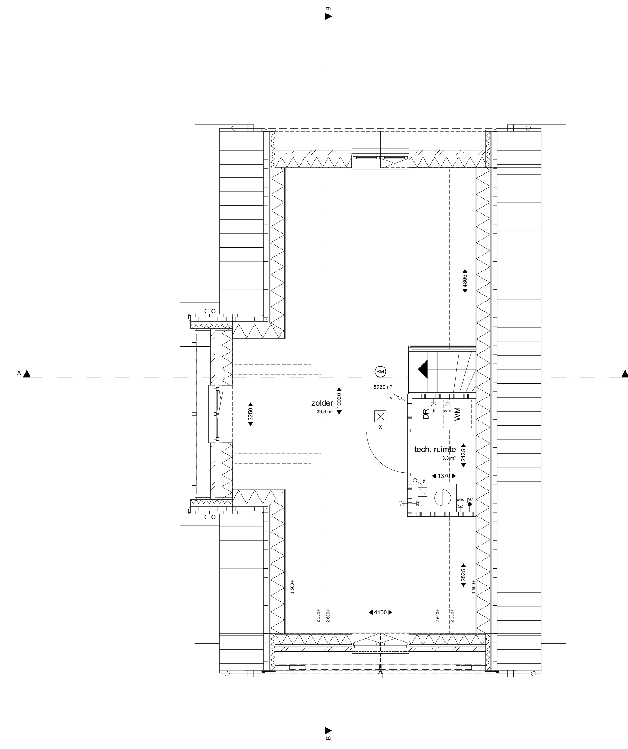
1:50 2e verdieping
