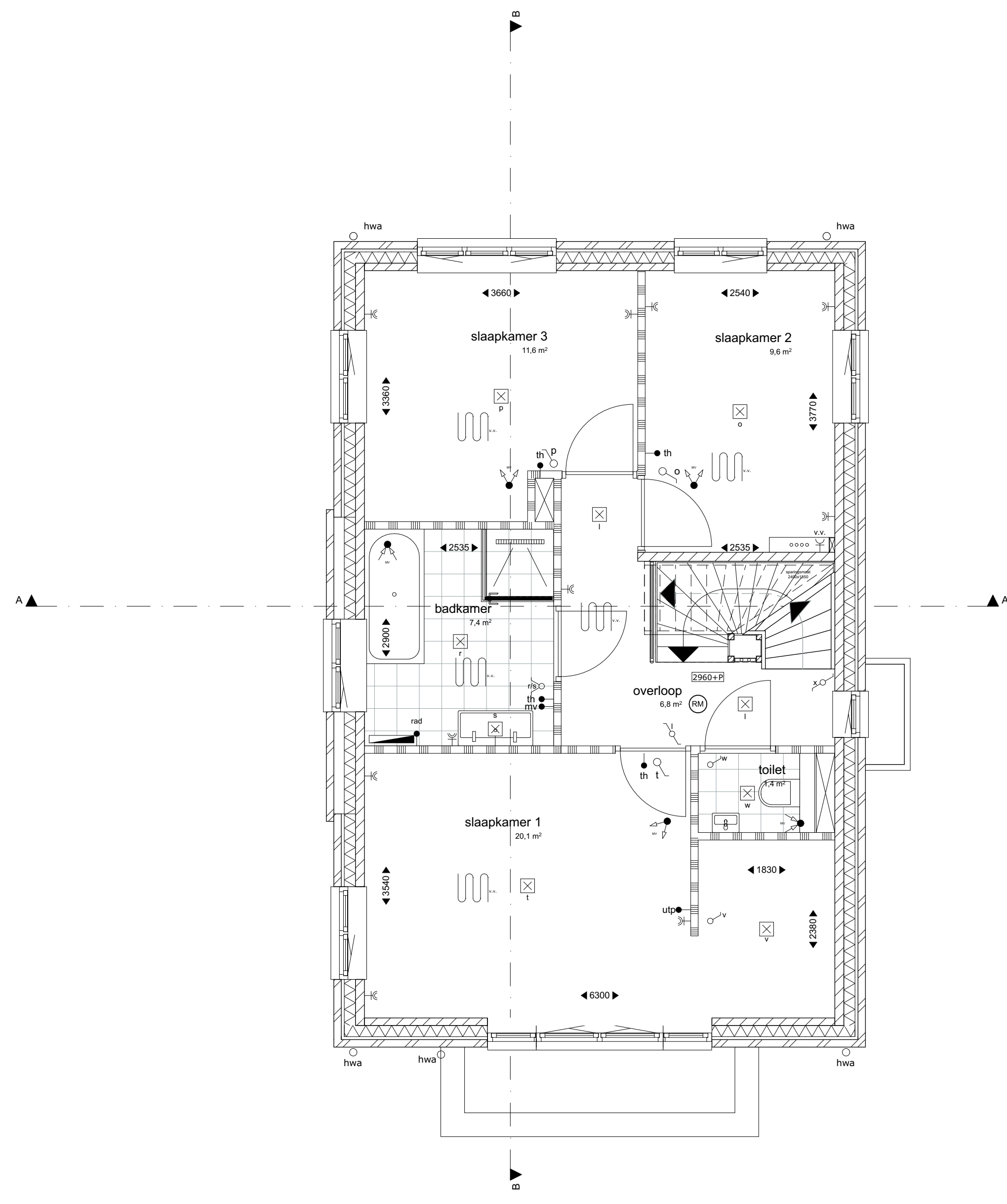
1:50 1e verdieping
