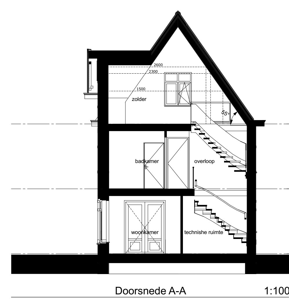
Doorsnede A-A 1:100
