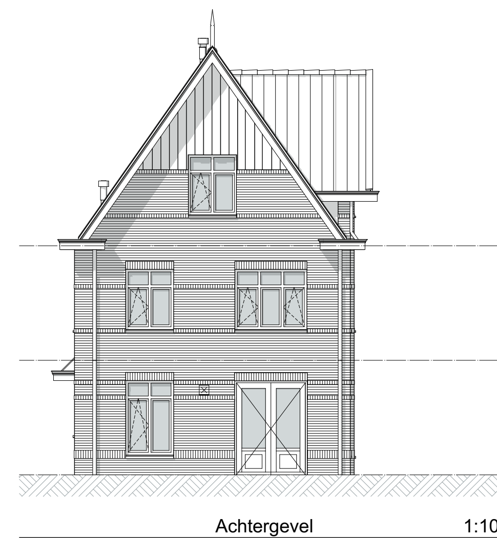
Achtergevel 1:100
