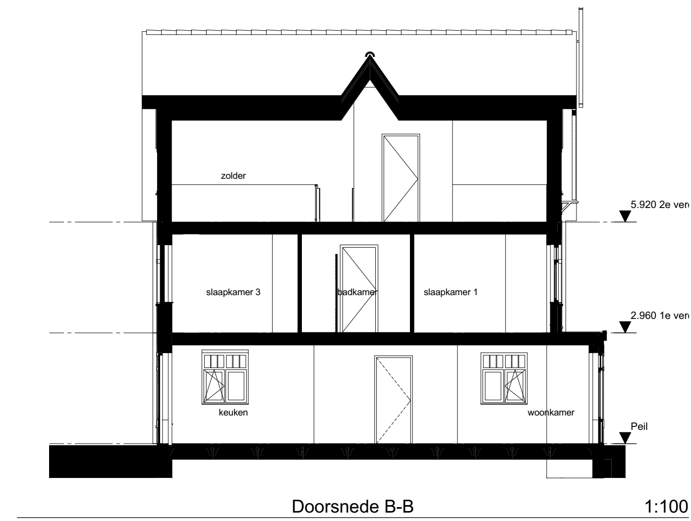
Doorsnede B-B 1:100
