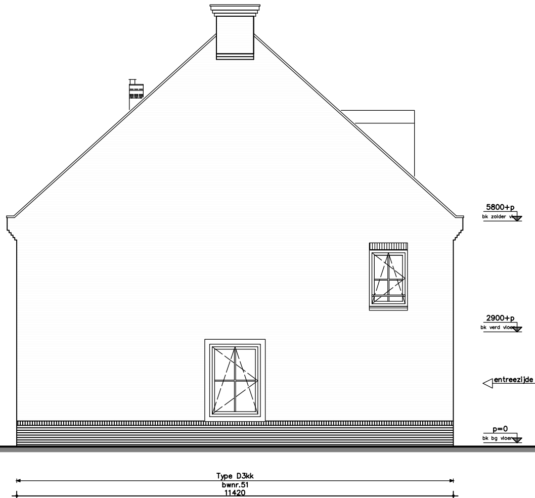
linkerzijgevel
