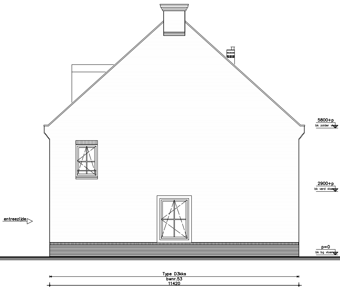
rechterzijgevel
