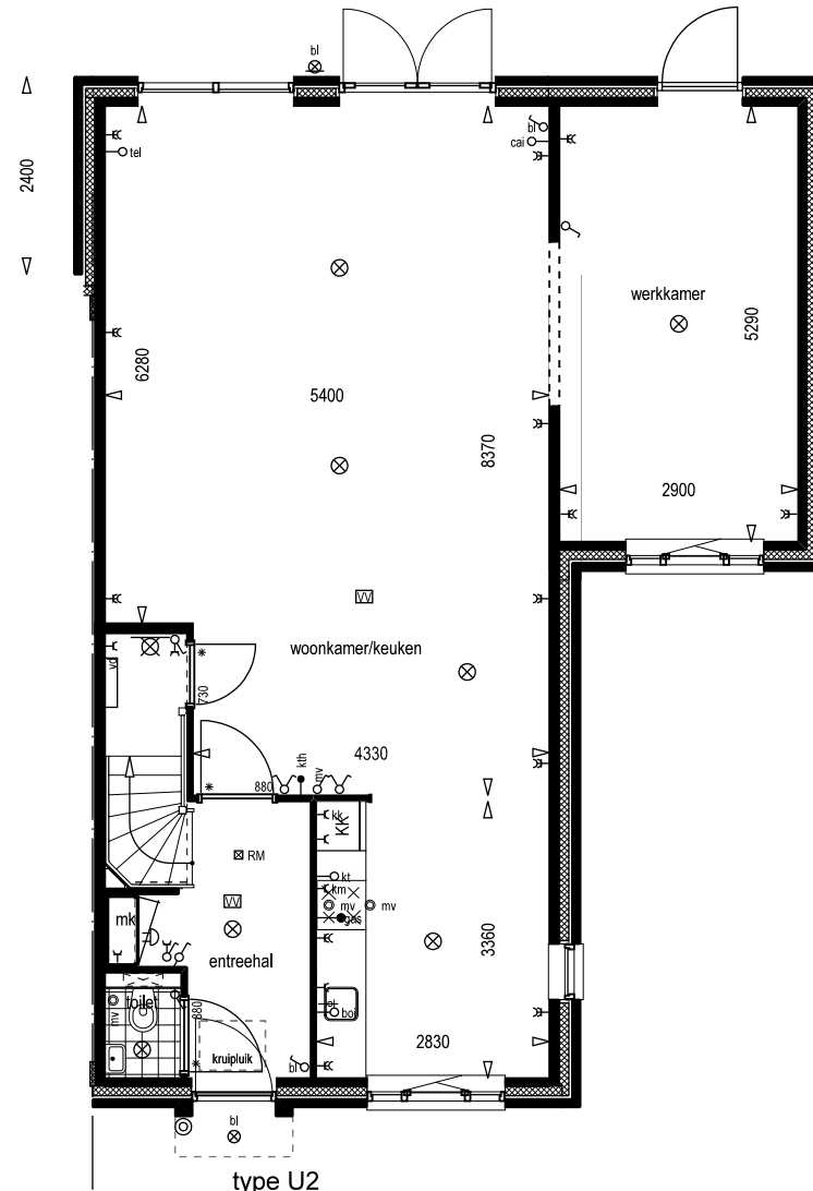
type U2 optie uitbouw 2400 mm optie garage bij woonkamer i.c.m. uitbouw
