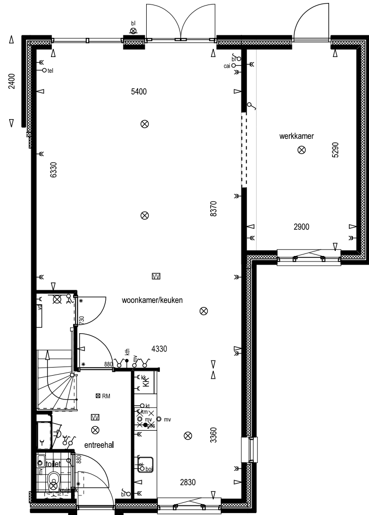
type U1 optie uitbouw 2400 mm optie garage bij woonkamer i.c.m. uitbouw
