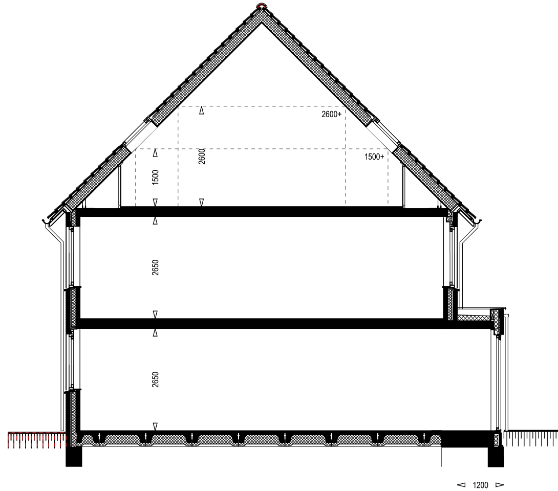
type U1 uitbouw 1200 mm optie dakraam voor optie dakraam achter
