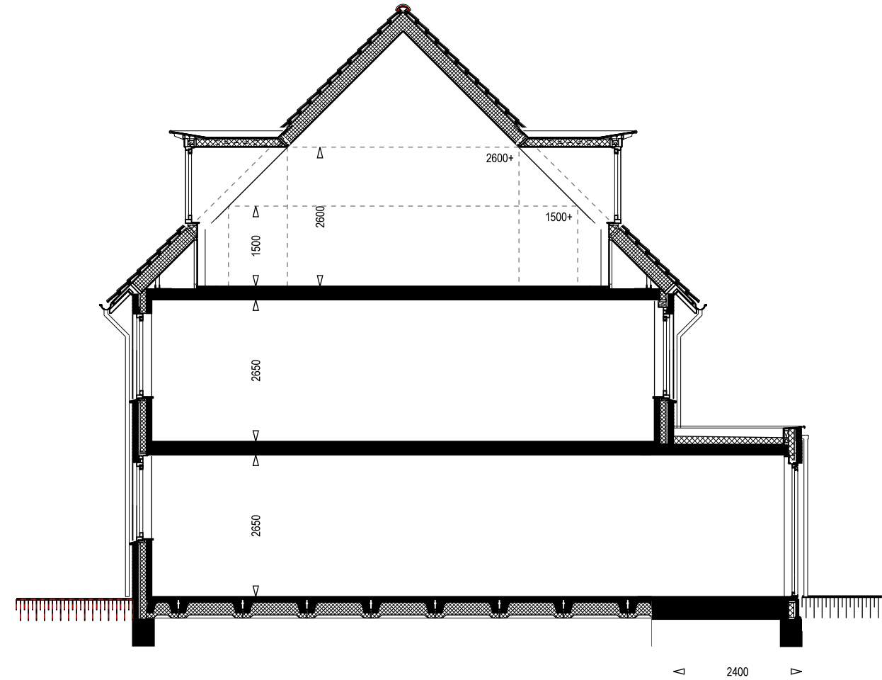
type U1 uitbouw 2400 mm optie dakkapel voor optie dakkapel achter
