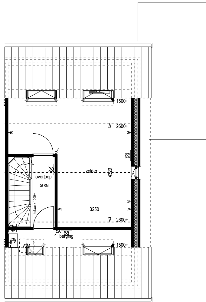
type U1/U2 optie indeling zolder optie dakraam groot (3x) optie dakraam klein (1x)
