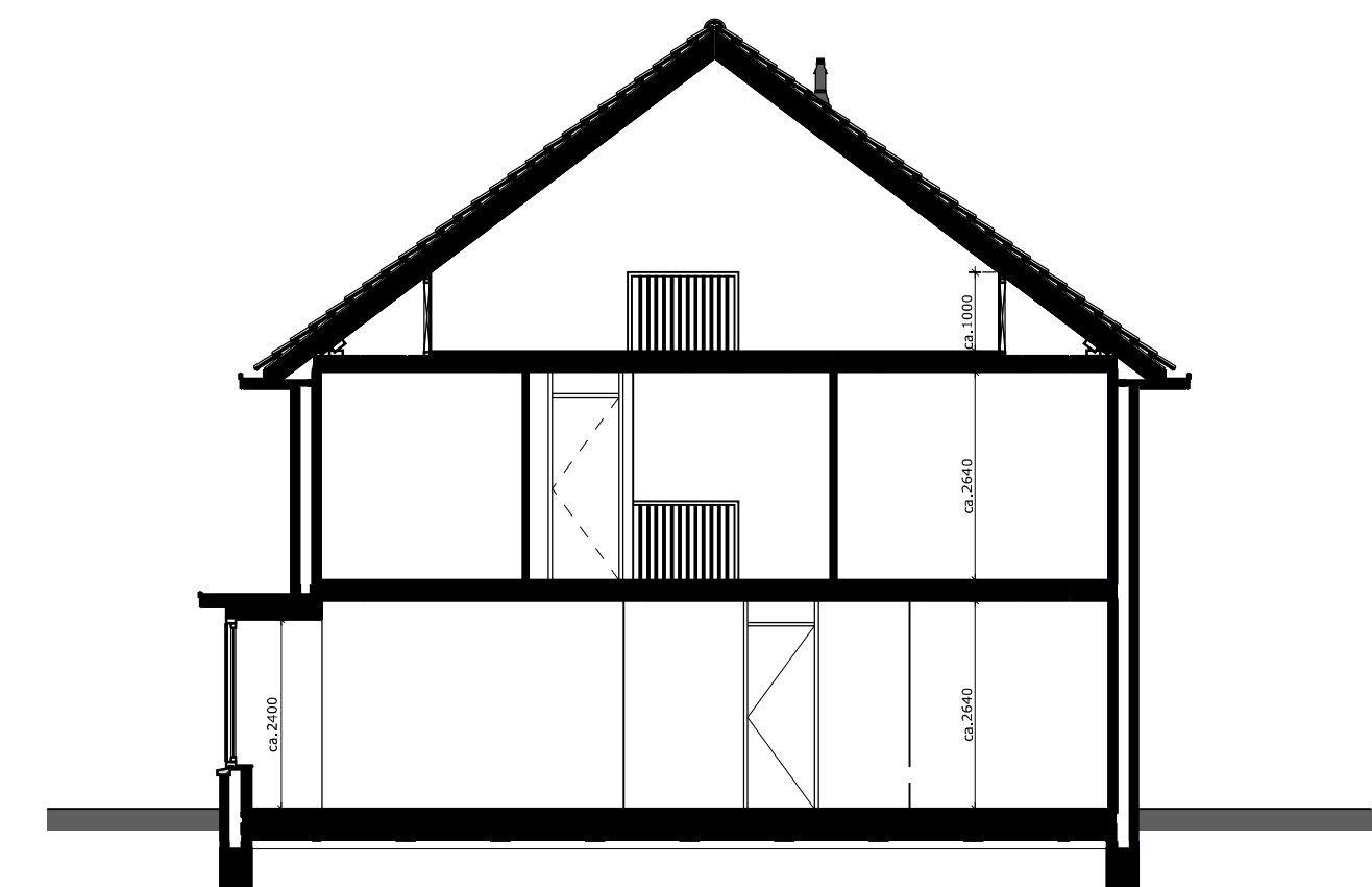
Principe doorsnede
