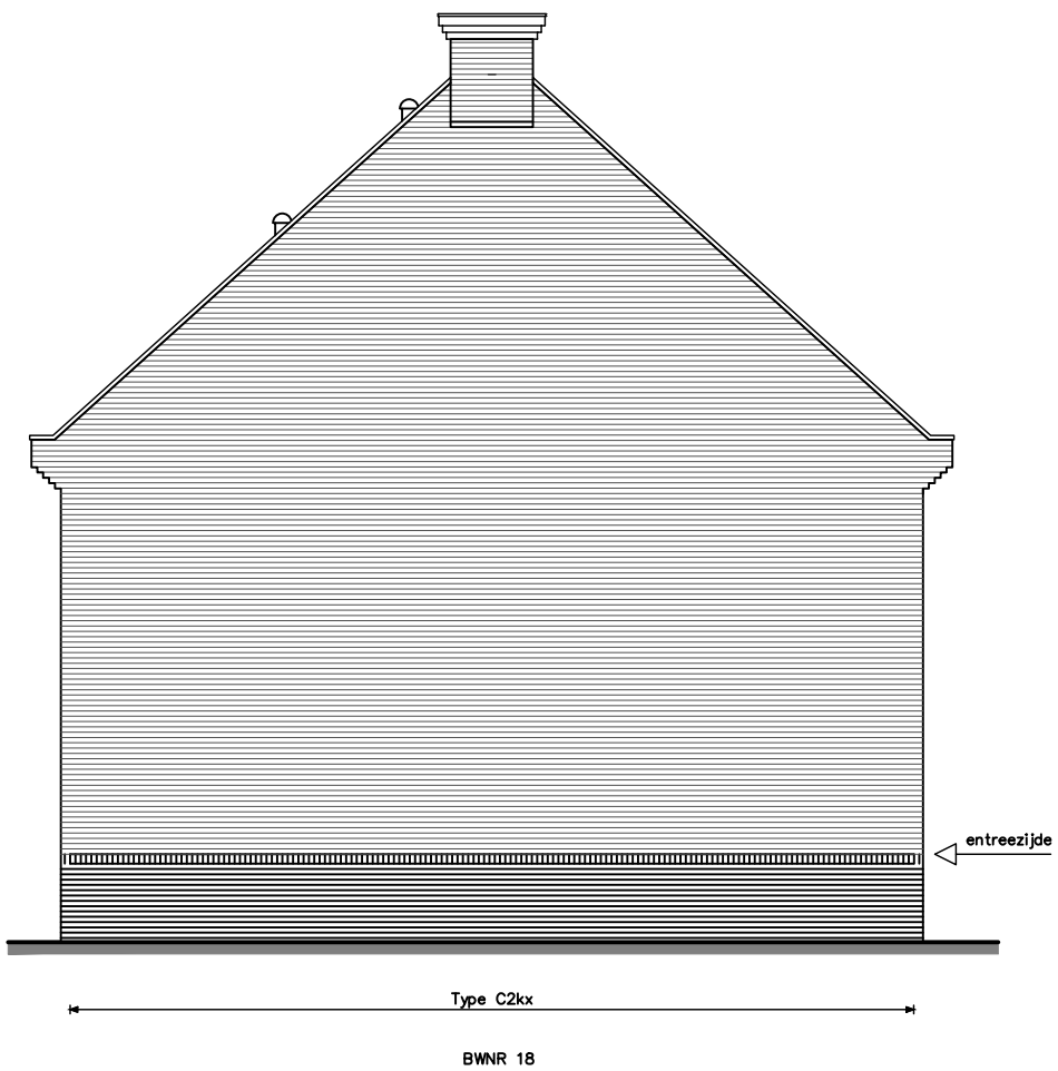
ZIJGEVEL links
