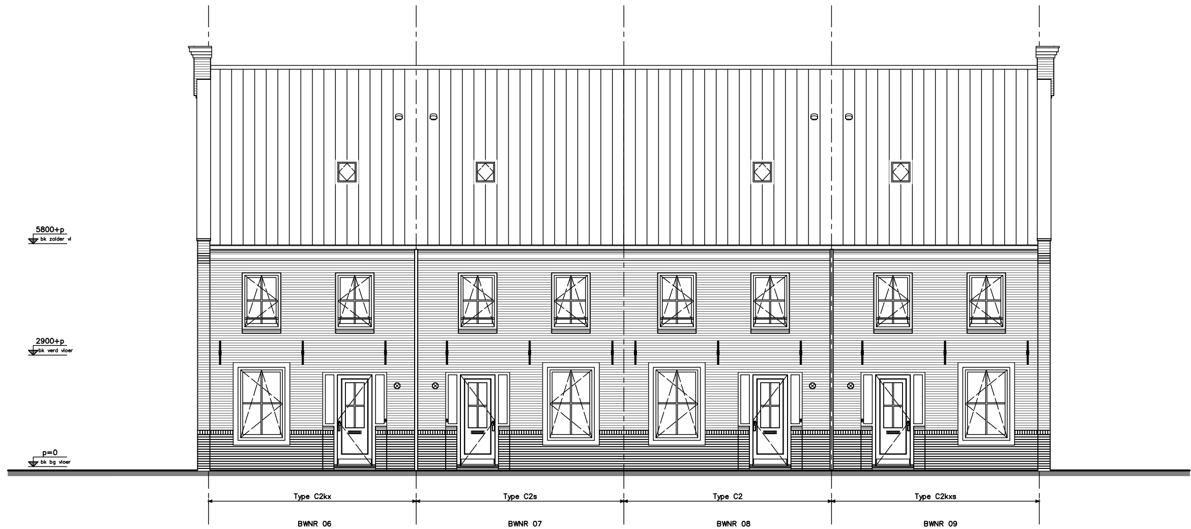
VOORGEVEL
