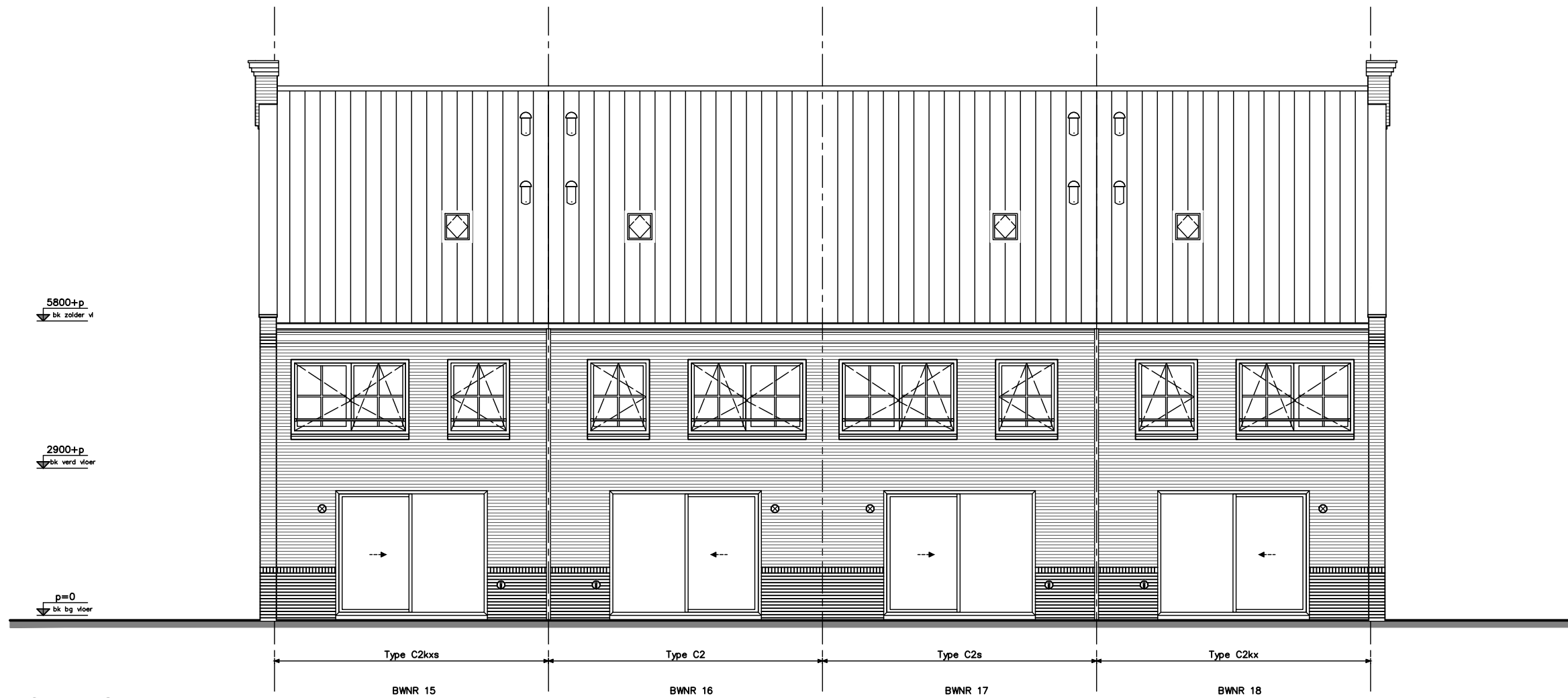
ACHTERGEVEL
