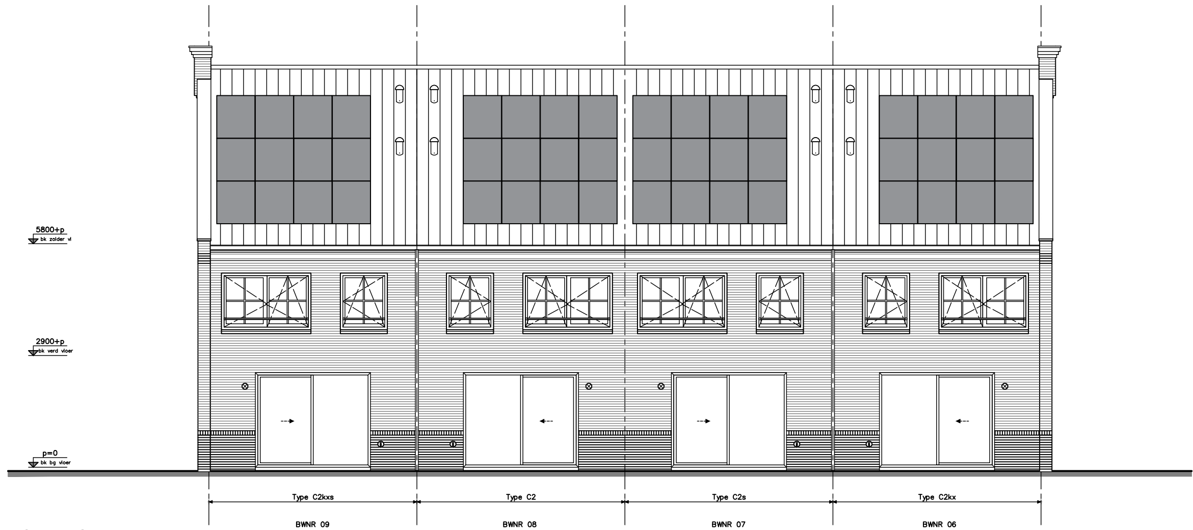
ACHTERGEVEL
