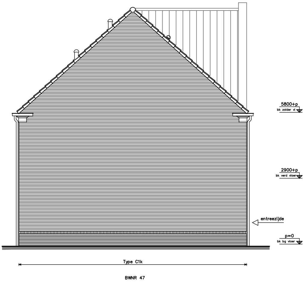
ZIJGEVEL links
