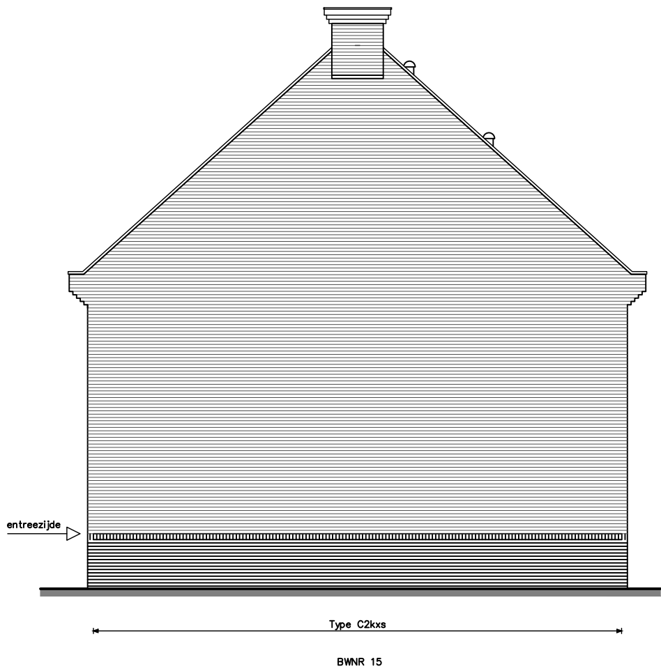
ZIJGEVEL rechts
