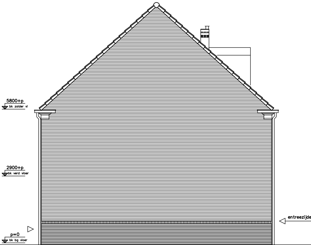
linkerzijgevel Type C2k bouwnr. 36
