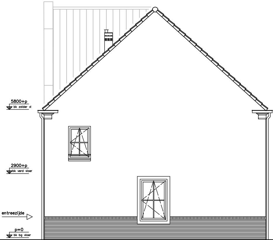
rechterzijgevel Type C1xkks bouwnr. 43
