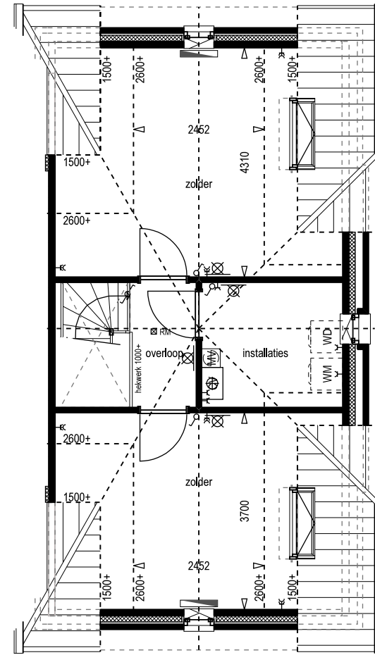
type W1 optie indeling zolder optie dakraam zijgevel (2x)
