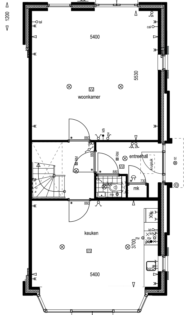
type W1 optie uitbouw 1200 mm optie afsluiten keuken/woonkamer optie erker voorgevel
