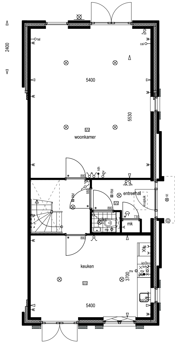
type W1 optie uitbouw 2400 mm optie afsluiten keuken/woonkamer
