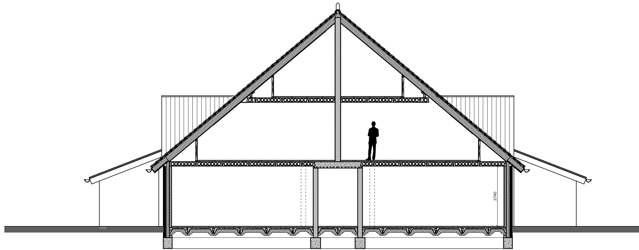
Principe doorsnede
