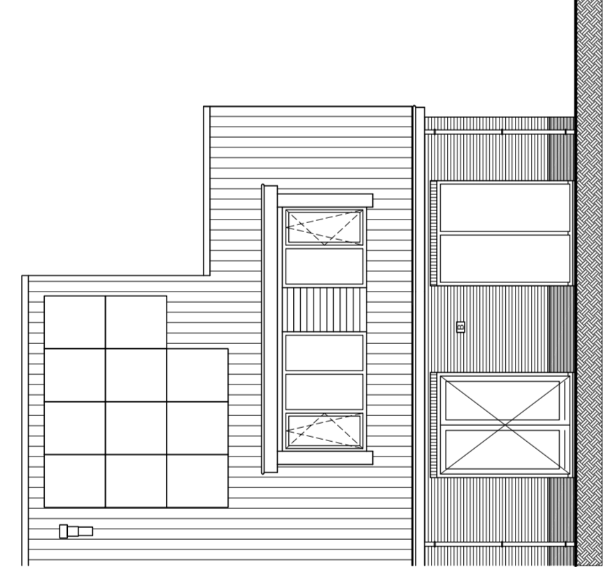
Kopgevel schaal 1:100 bouwnummer: 28 bouwnummer gespiegeld: 10 / 24
