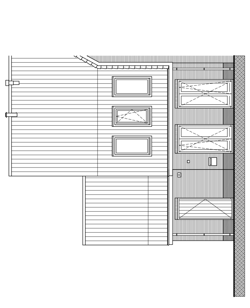
Doorsnede B10 schaal 1:100 bouwnummer: 28 bouwnummer gespiegeld: 10 / 24
