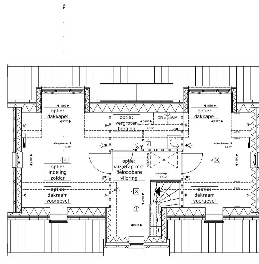
1:100 2e verdieping
