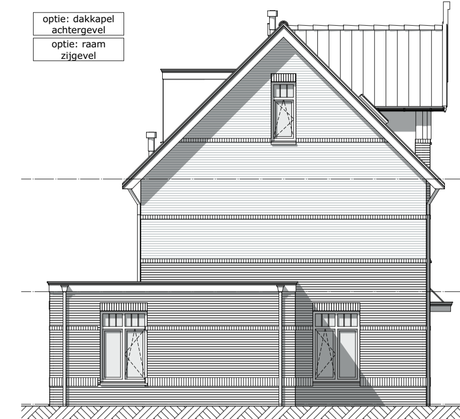
1:100 Linkergevel
