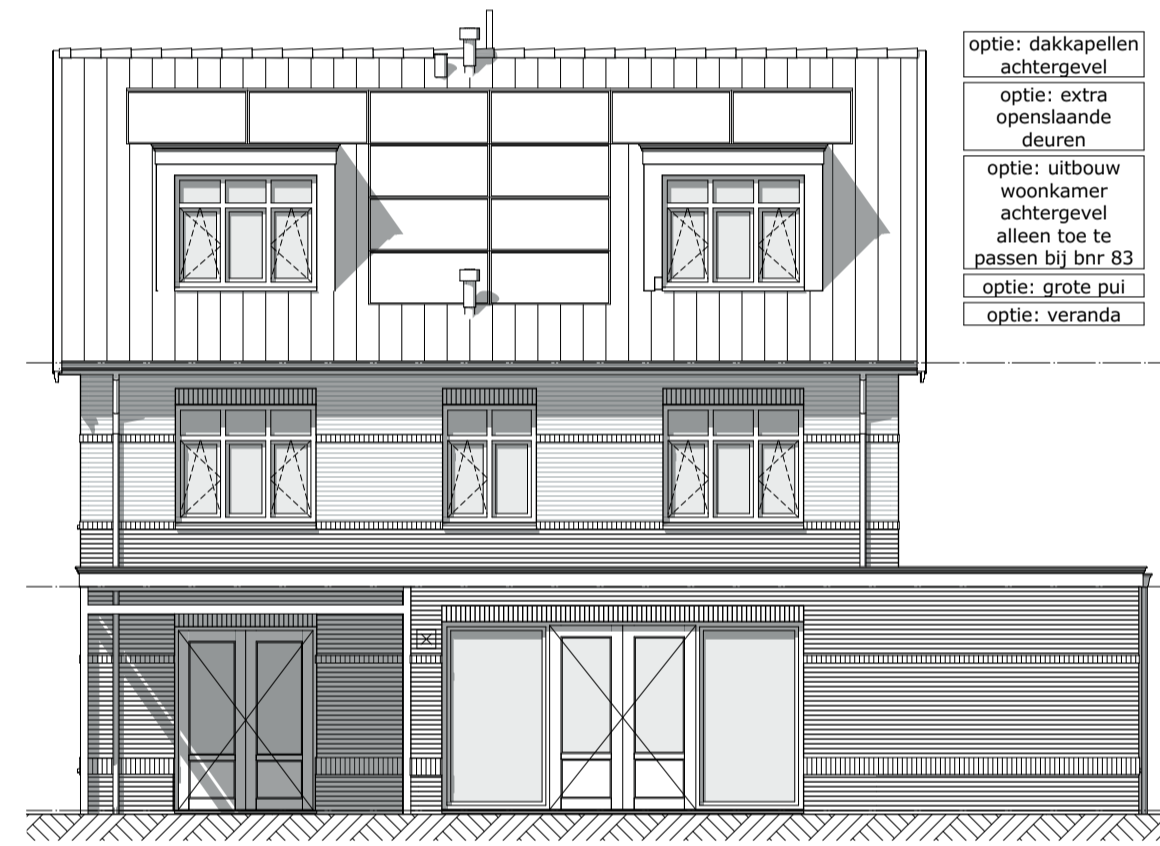
1:100 Achtergevel
