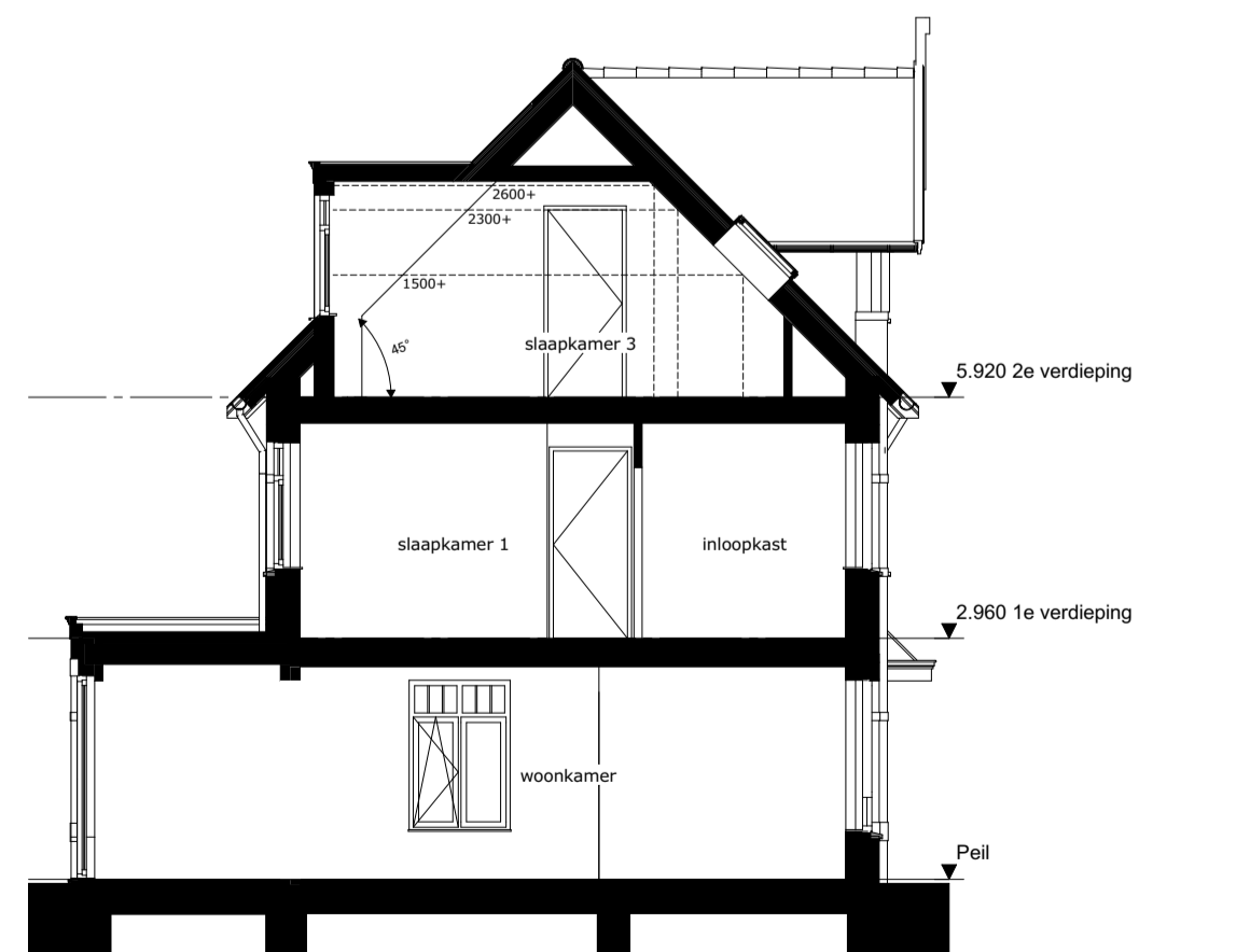
1:100 Doorsnede B-B
