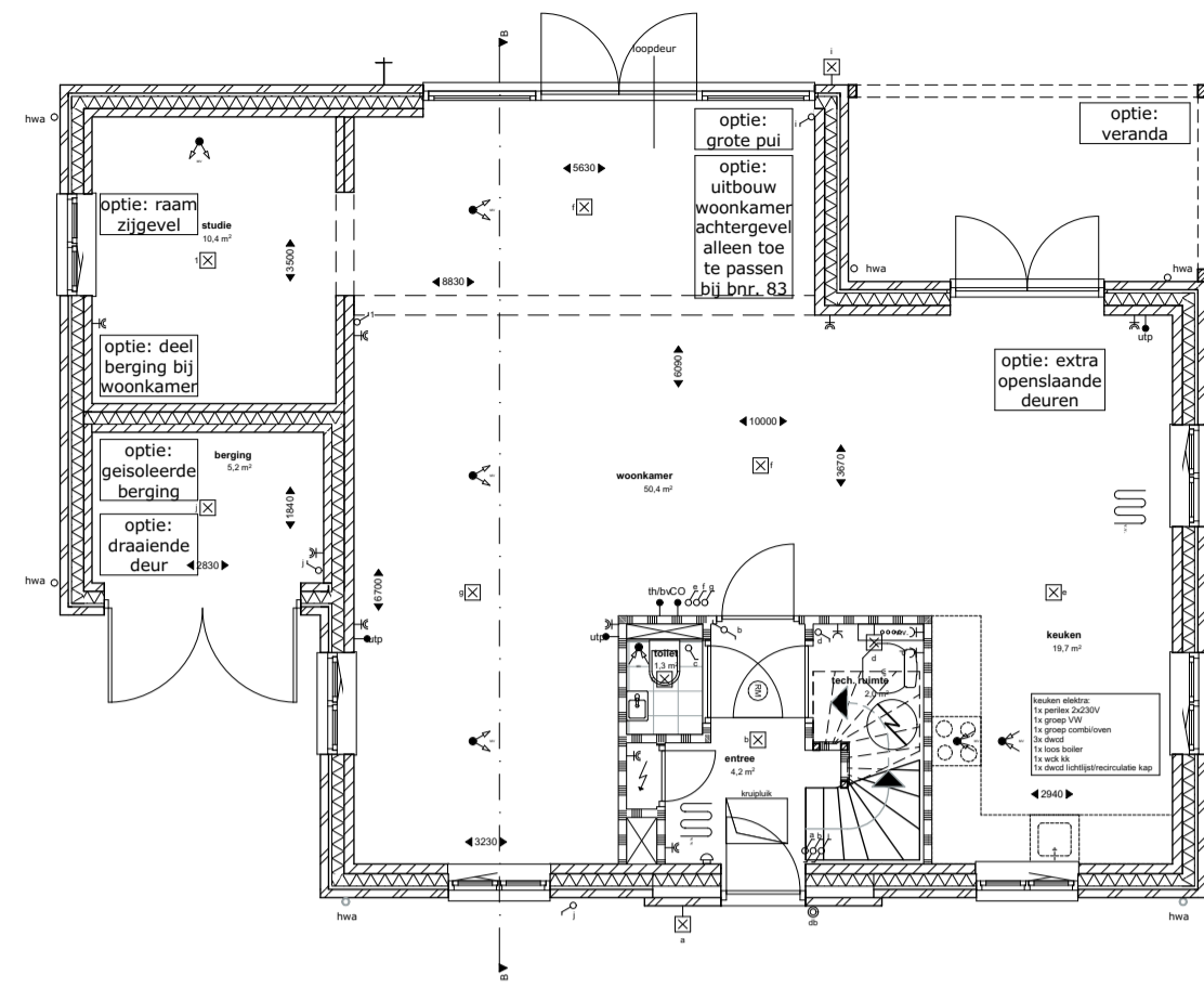
1:100 Begane grond
