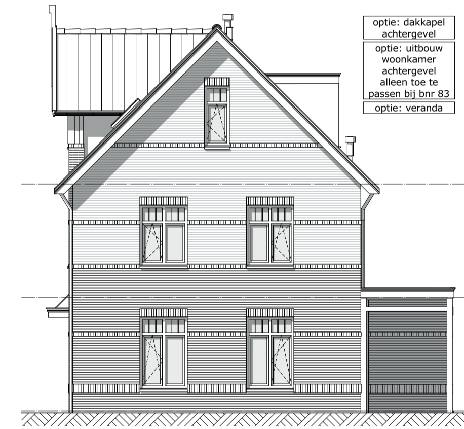
1:100 Rechtergevel
