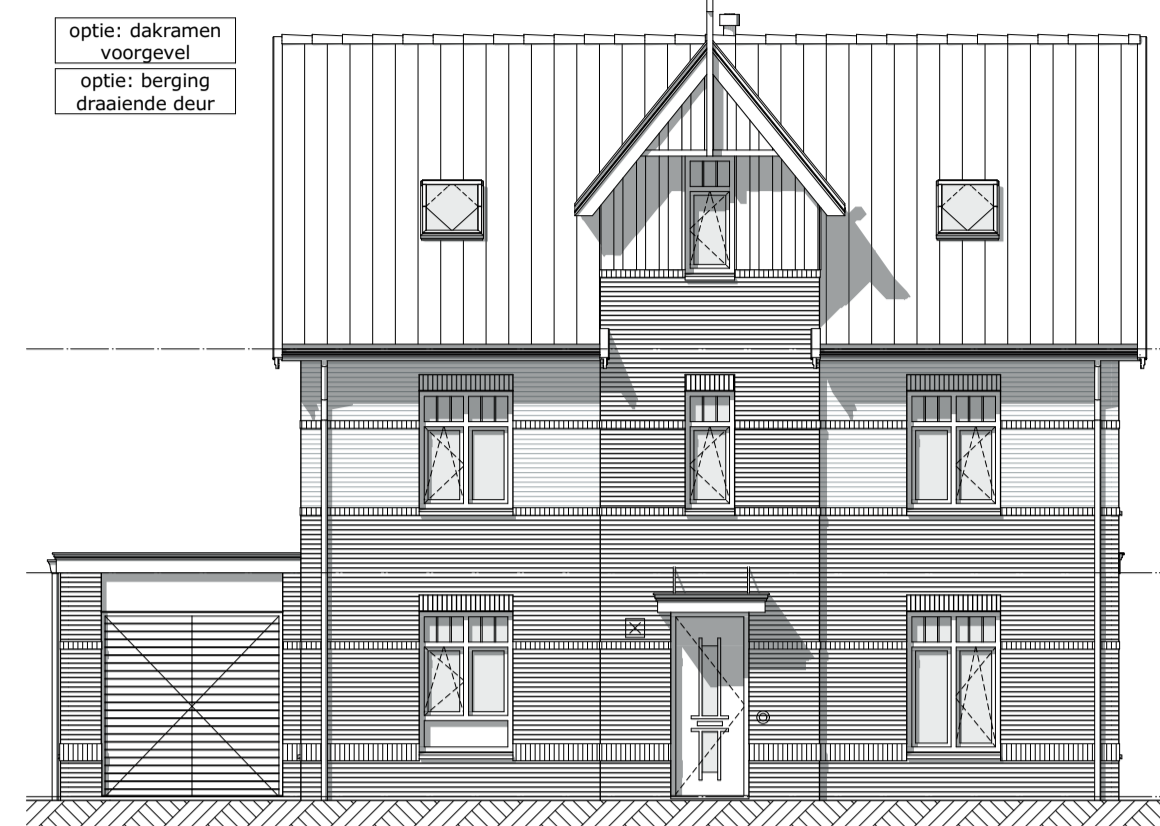
1:100 Voorgevel
