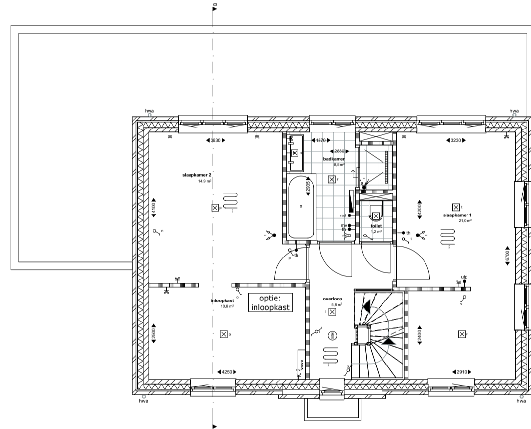
1:100 1e verdieping
