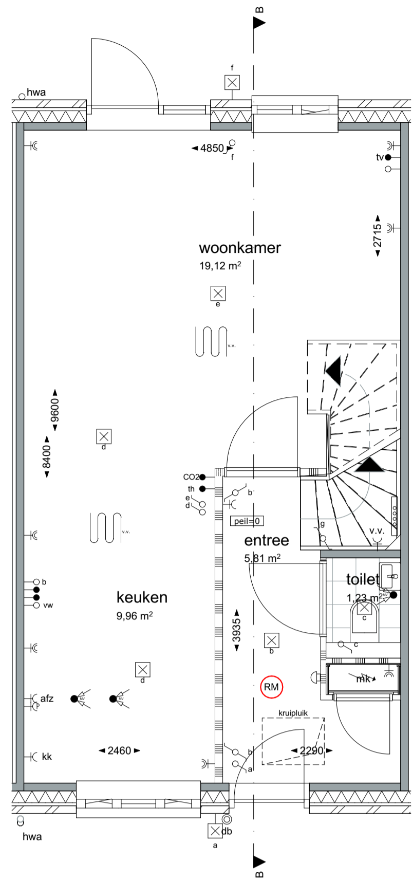
1:50 Begane grond
