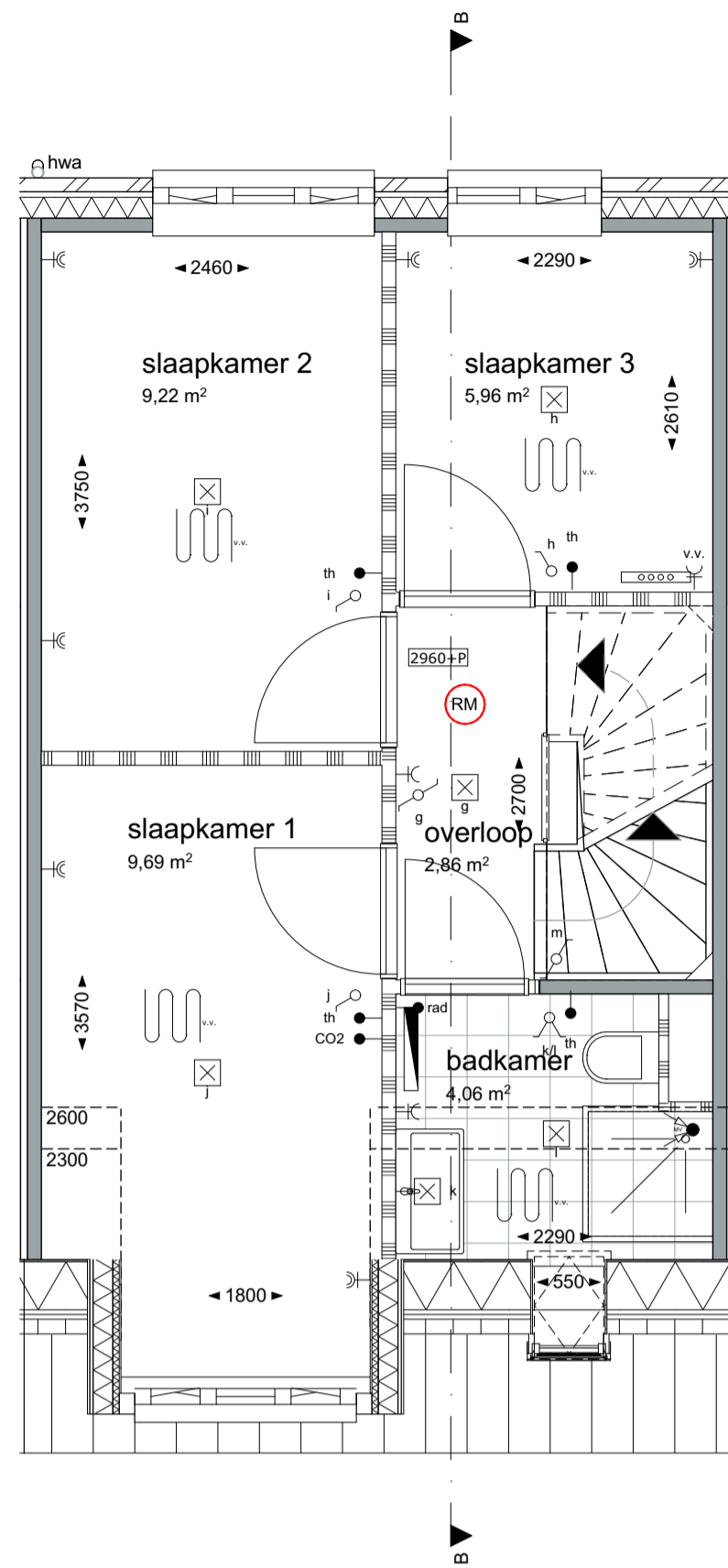
1:50 1e verdieping
