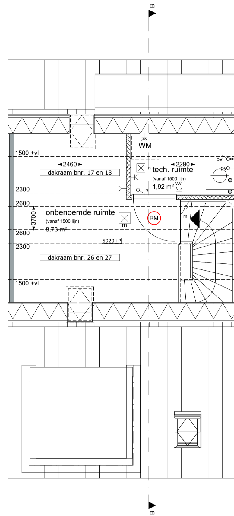
1:50 2e verdieping
