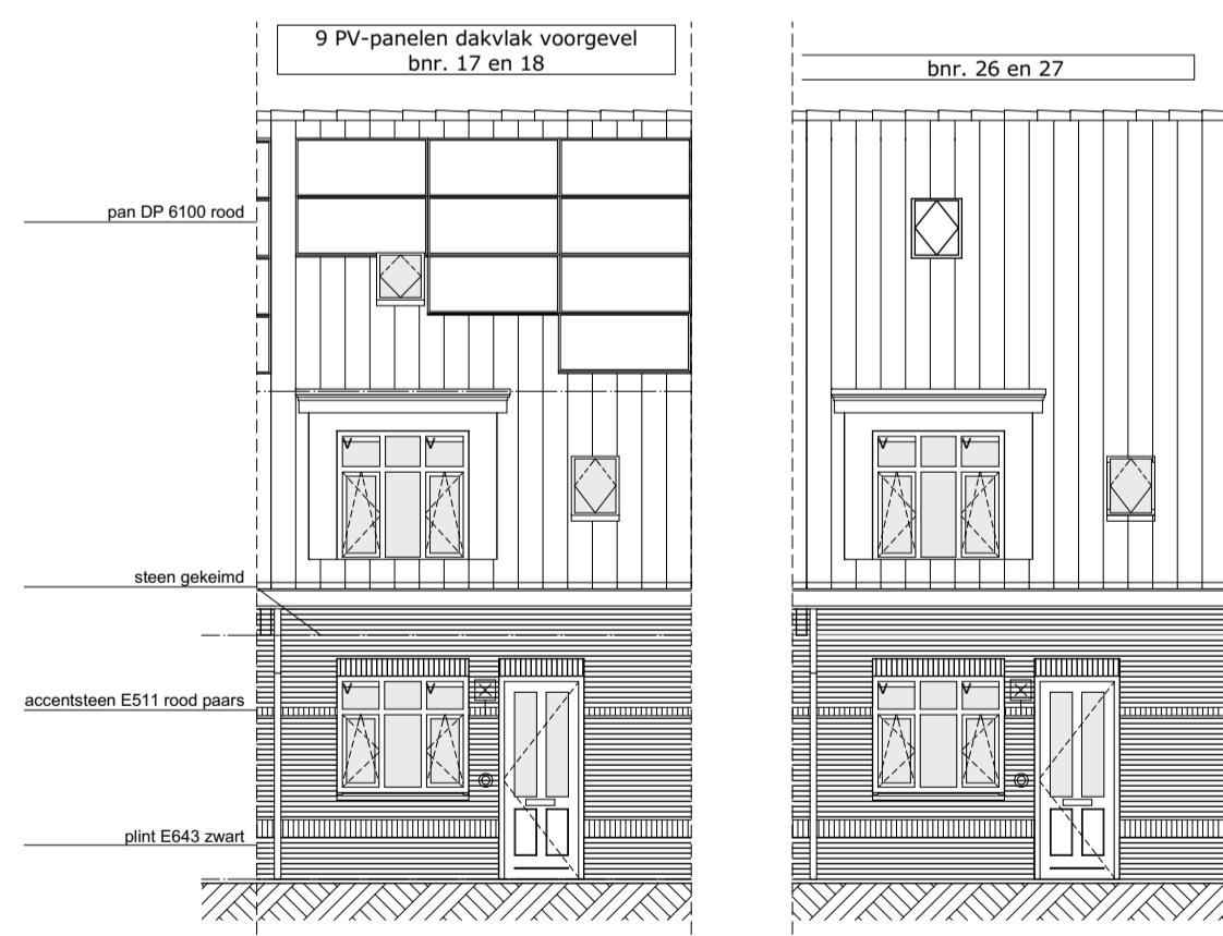
1:100 Voorgevel
