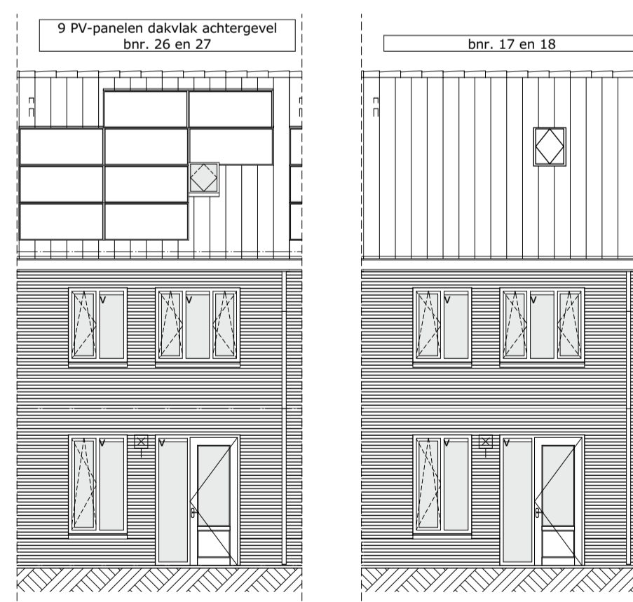
1:100 Achtergevel
