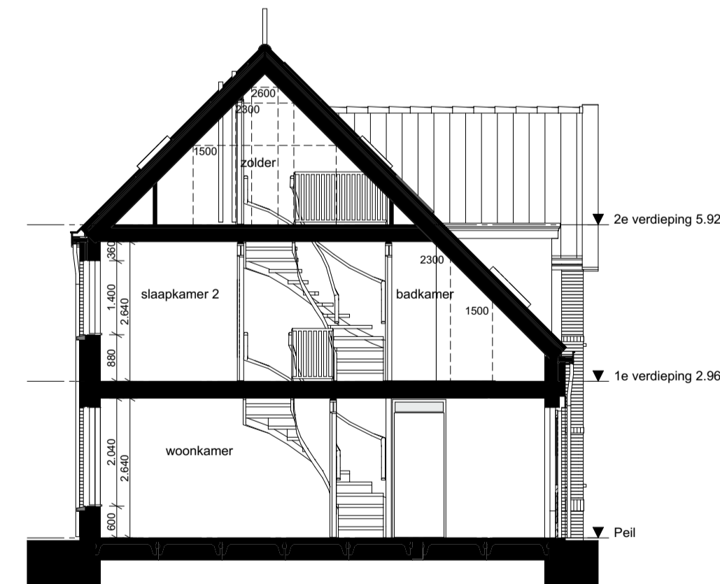
1:100 Doorsnede B-B A1T
