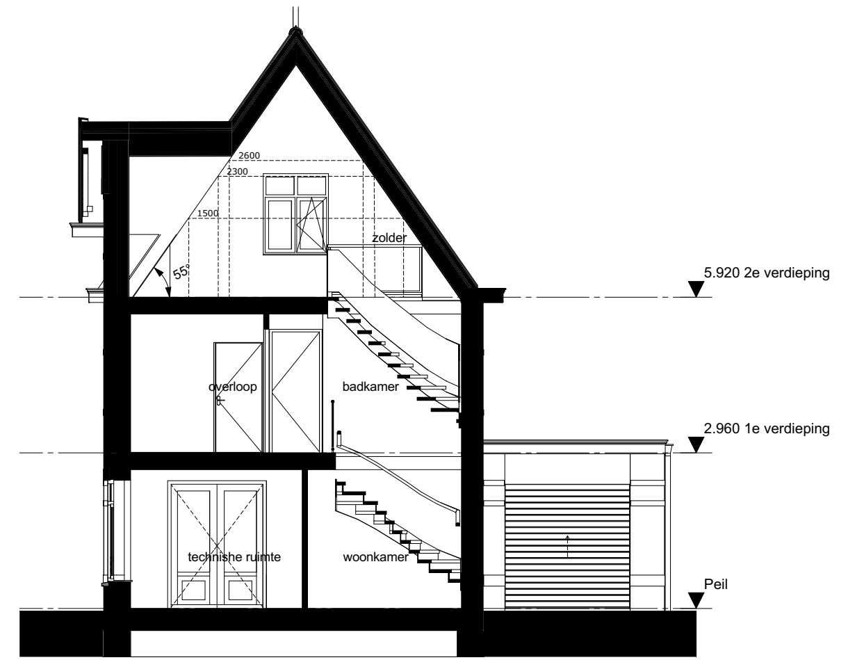
Doorsnede A-A 1:100
