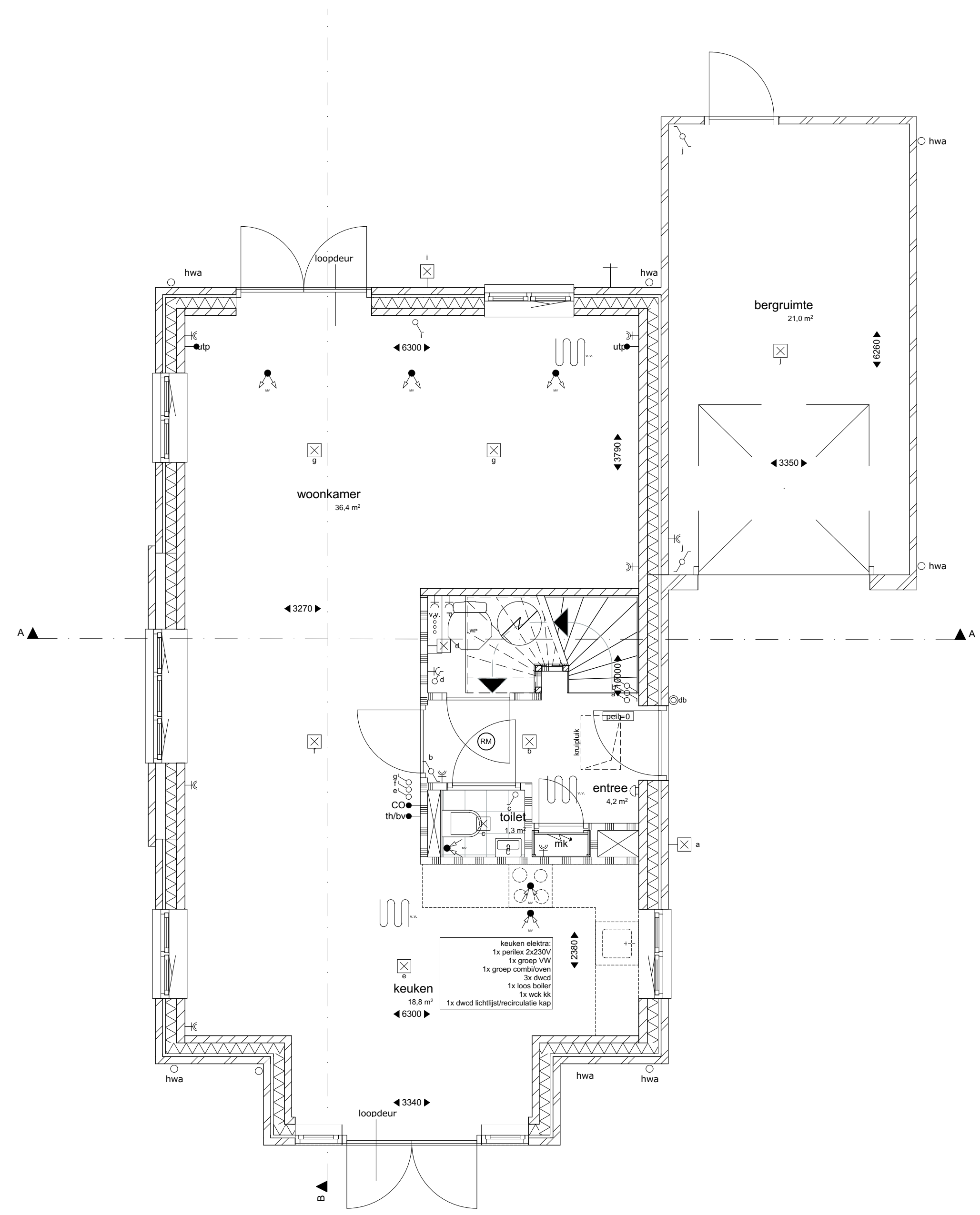
1:50 Begane grond
