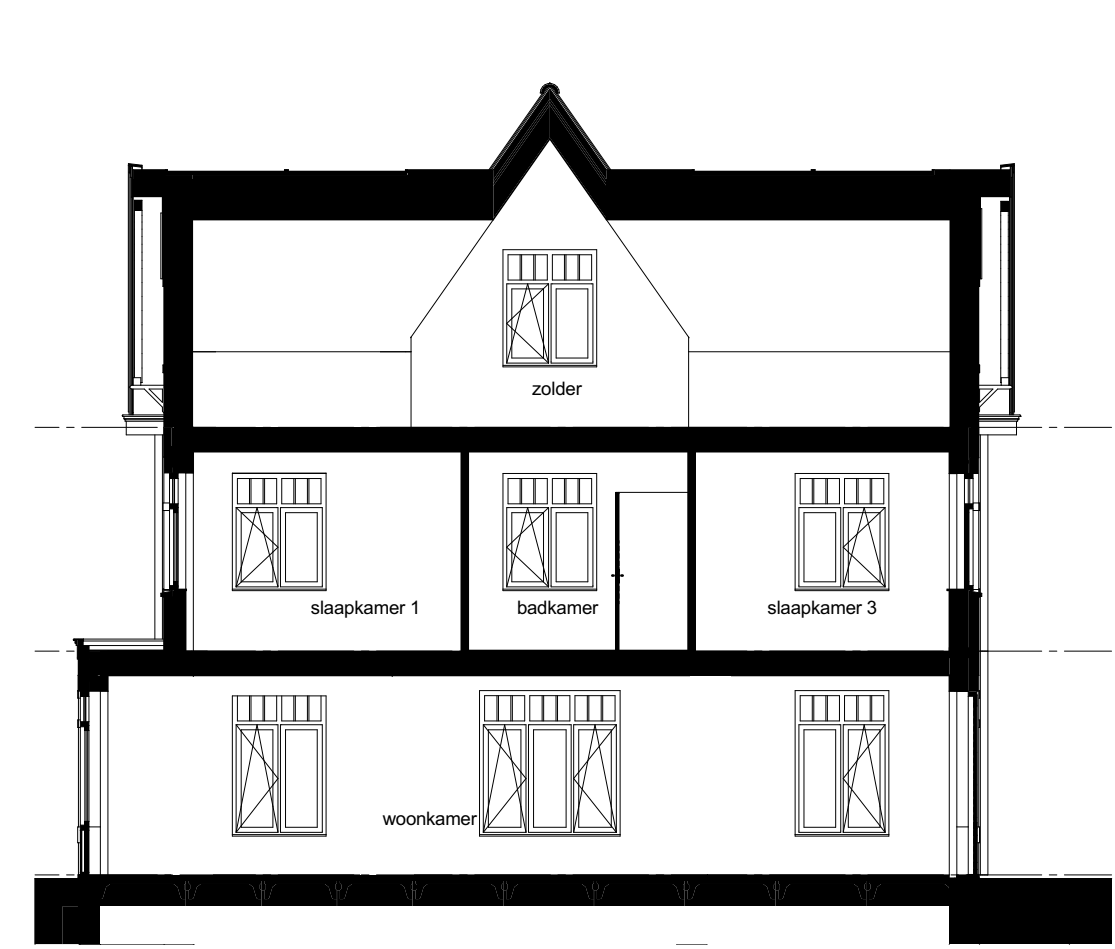
Doorsnede B-B 1:100
