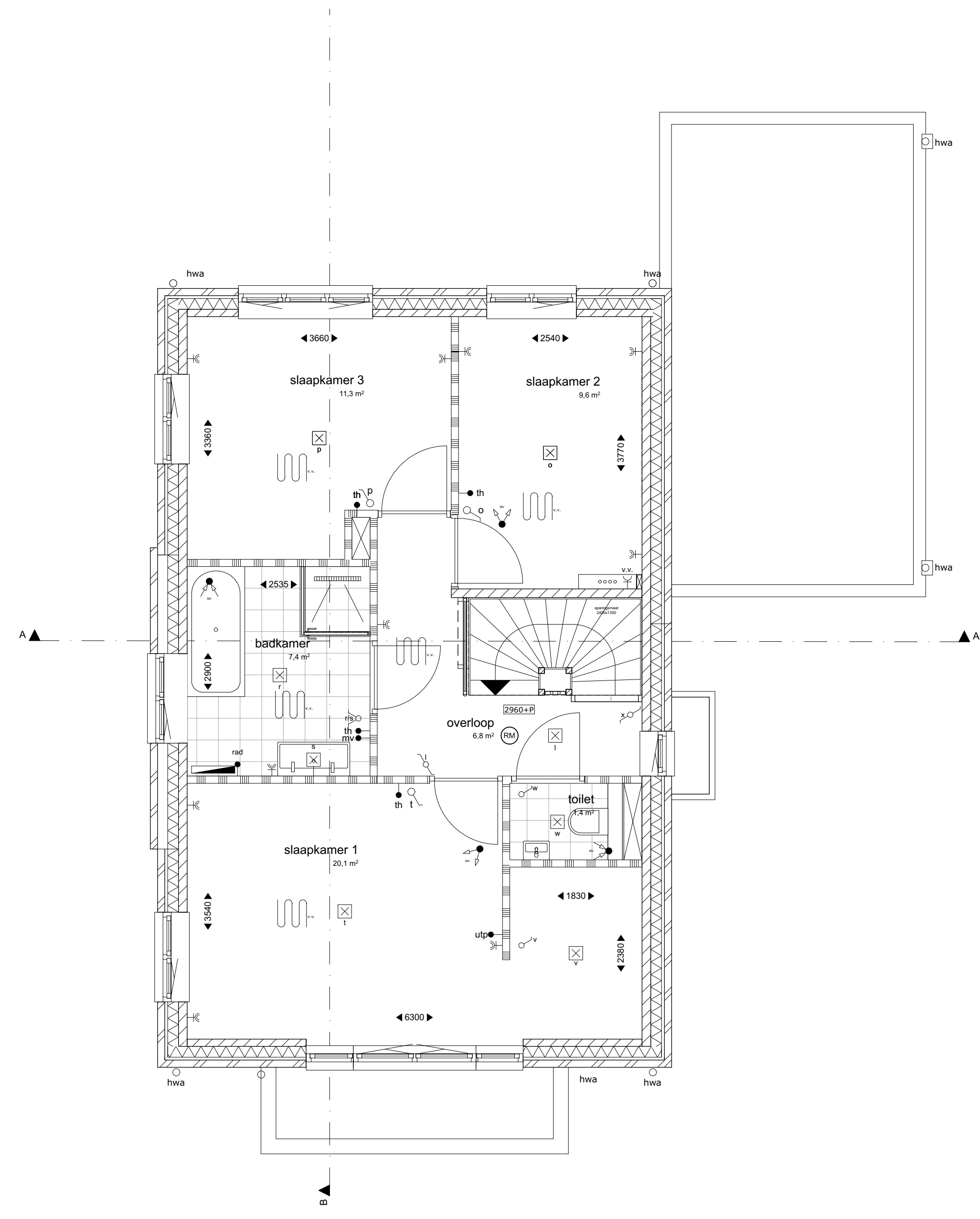
1:50 1e verdieping
