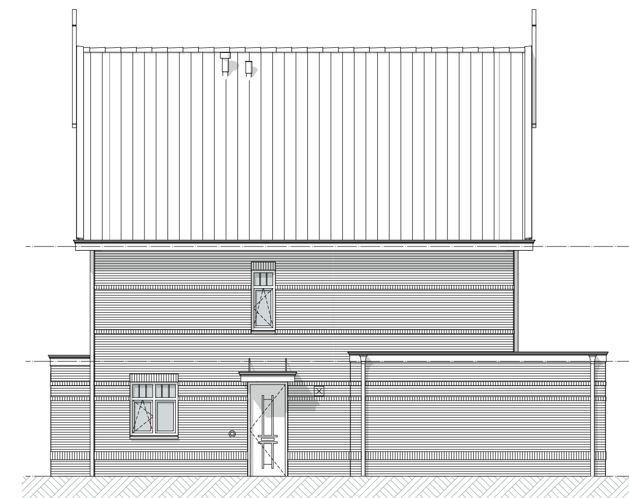
Rechtergevel 1:100
