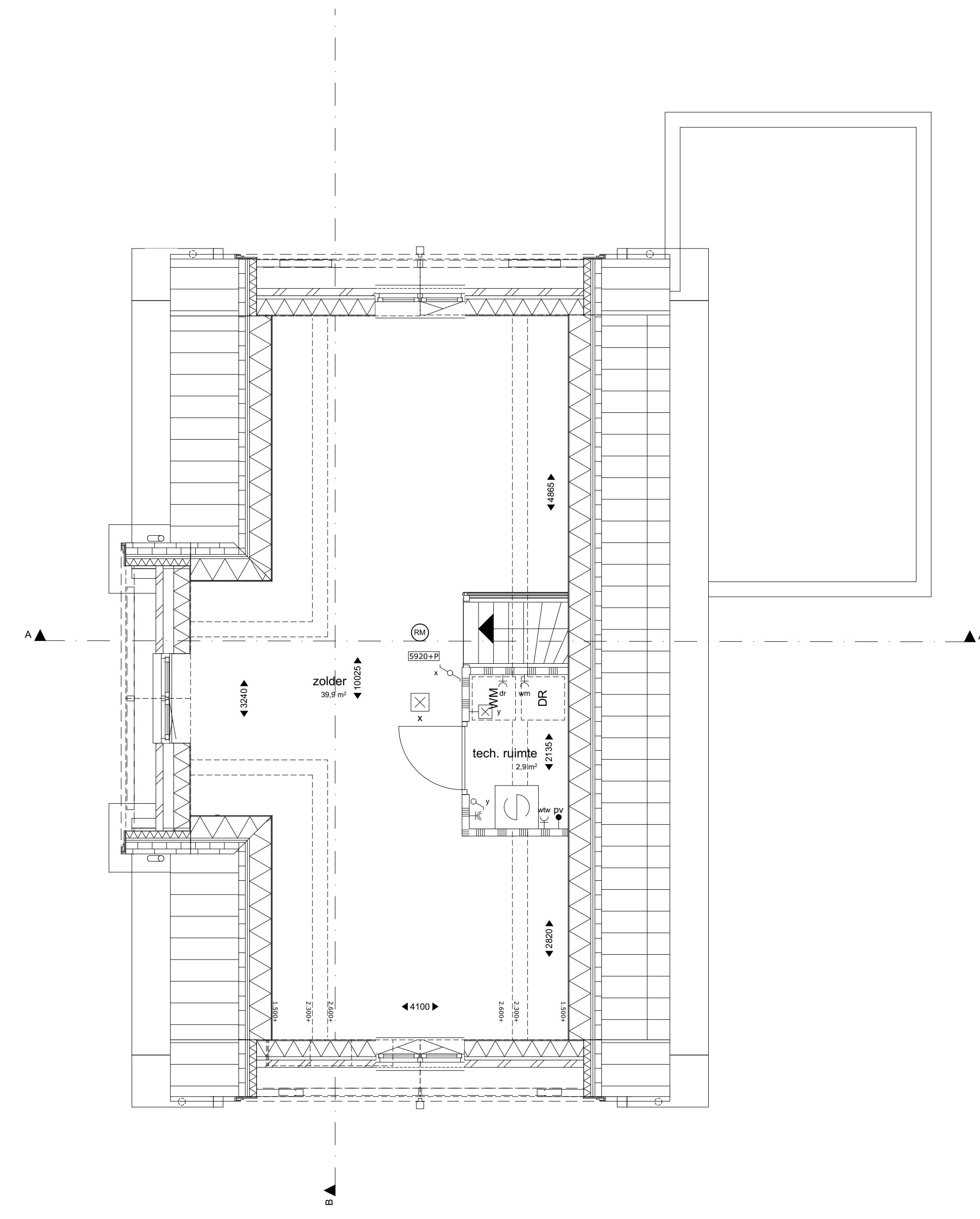
1:50 2e verdieping
