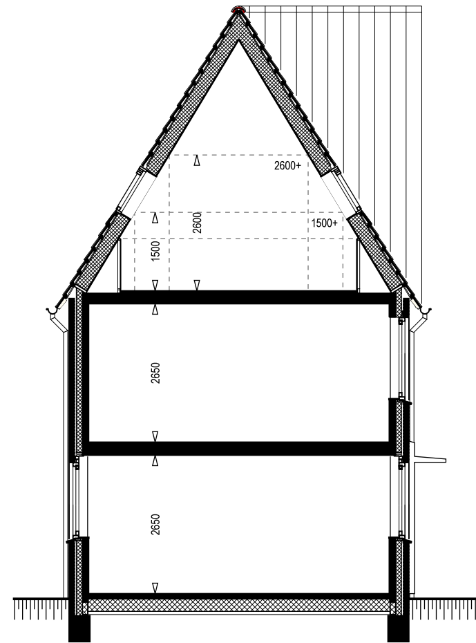
type Y optie dakraam zijgevel
