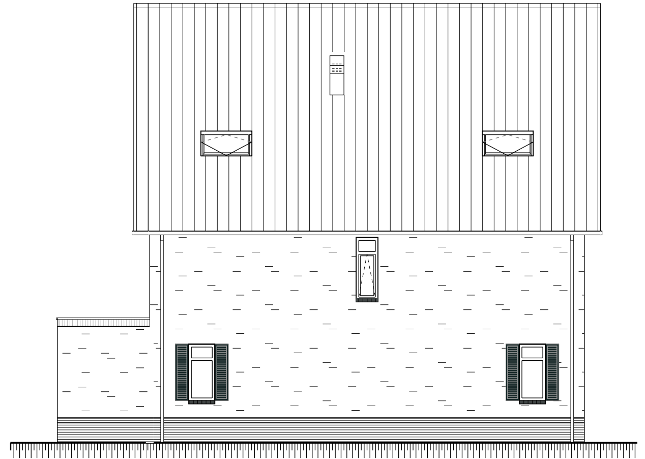
type Y optie uitbouw 2400mm optie dakraam groot (2x)
