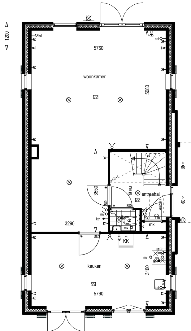
type Y optie uitbouw 1200 mm optie afsluiten keuken/woonkamer
