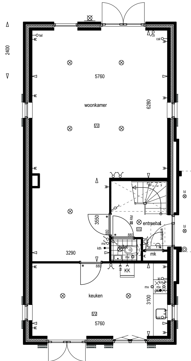
type Y optie uitbouw 2400 mm optie afsluiten keuken/woonkamer
