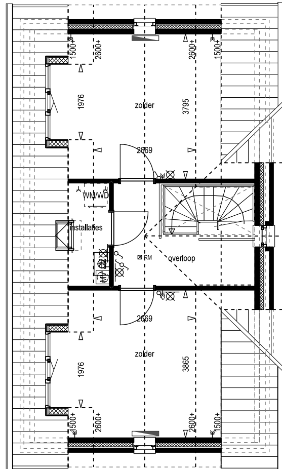
type Y optie indeling zolder optie dakkapel zijgevel (2x) optie dakraam klein
