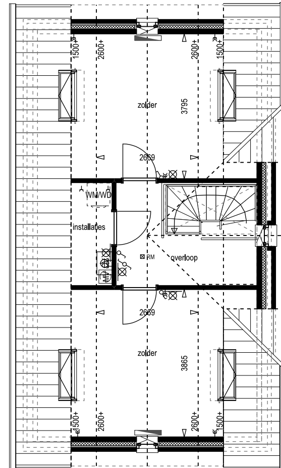
type Y optie indeling zolder optie dakraam groot (4x)
