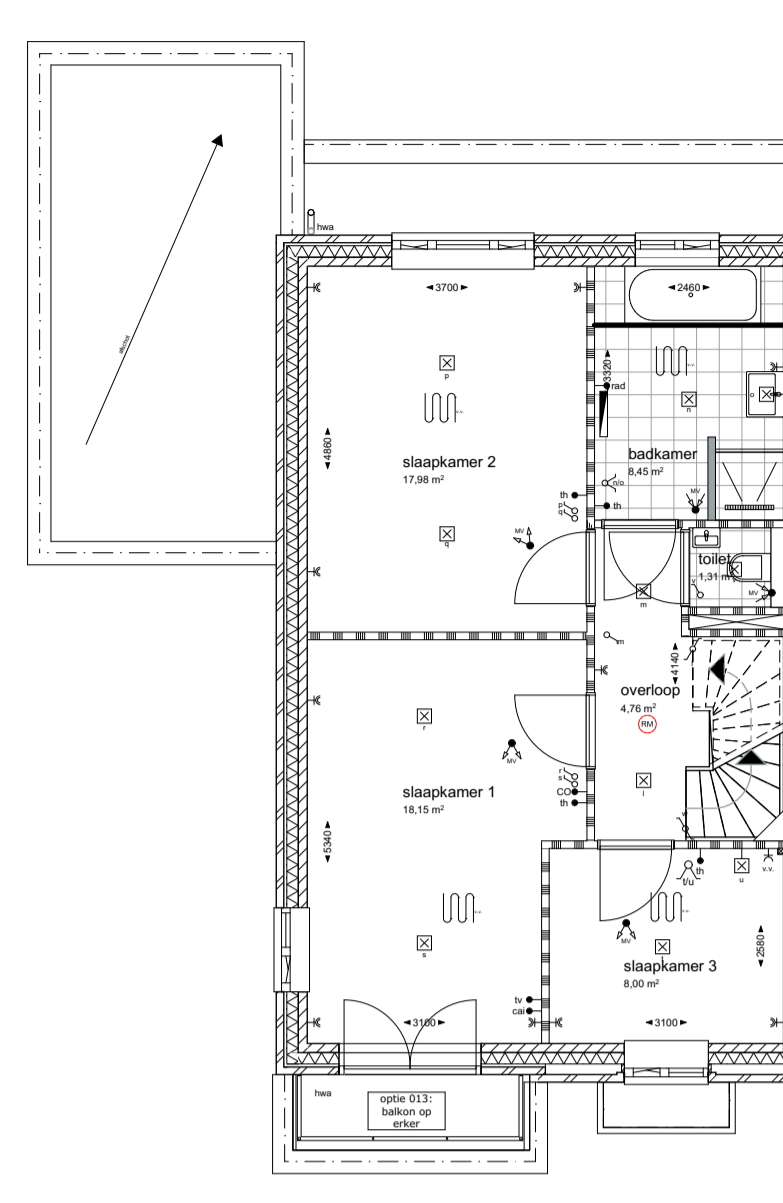
1:100 1e verdieping
