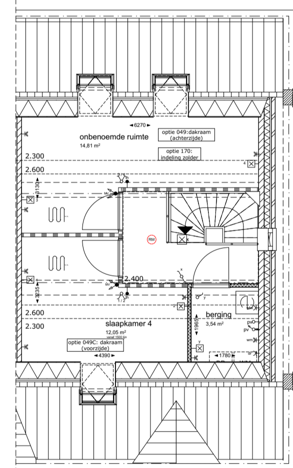
1:100 2e verdieping
