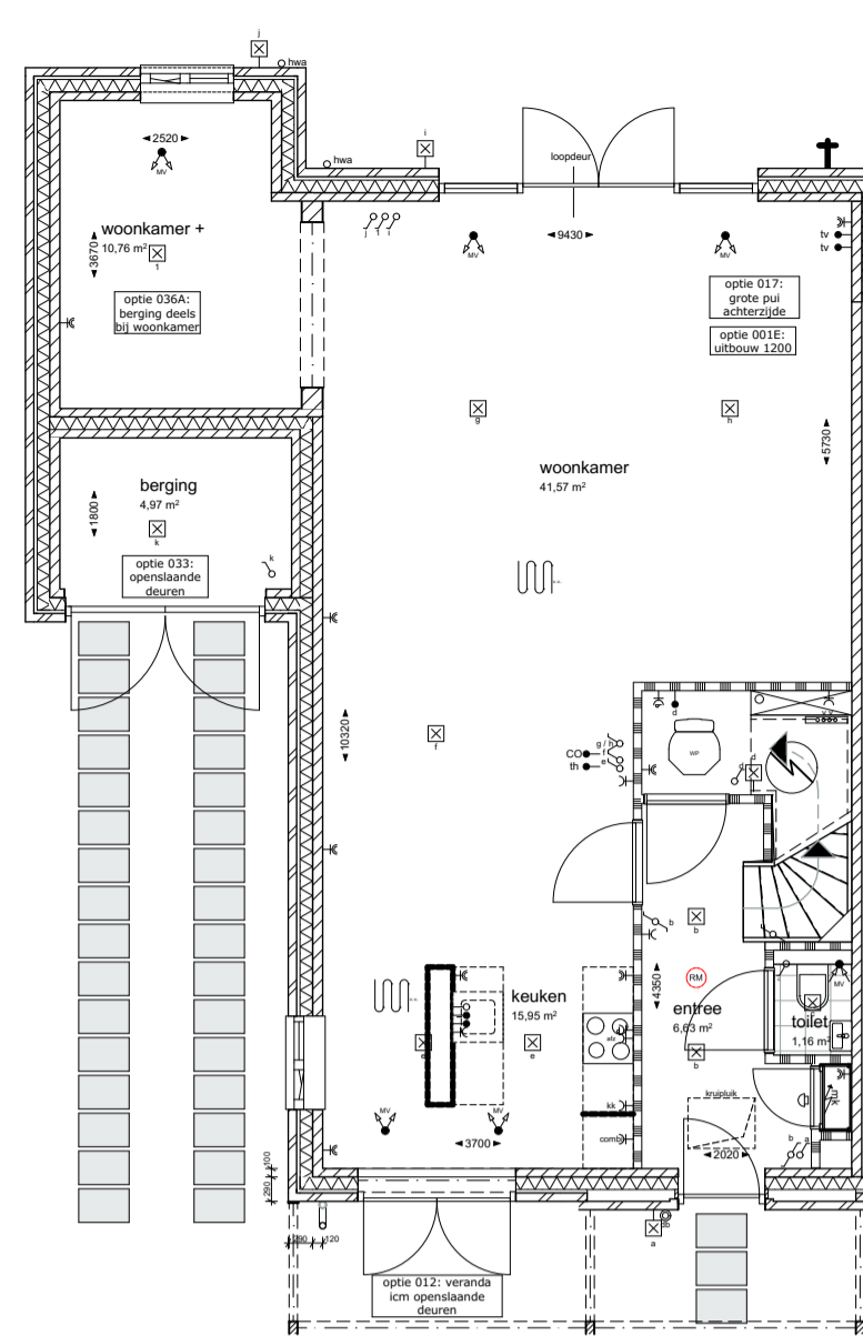
1:100 Begane grond veranda niet mogelijk in combinatie met erker
