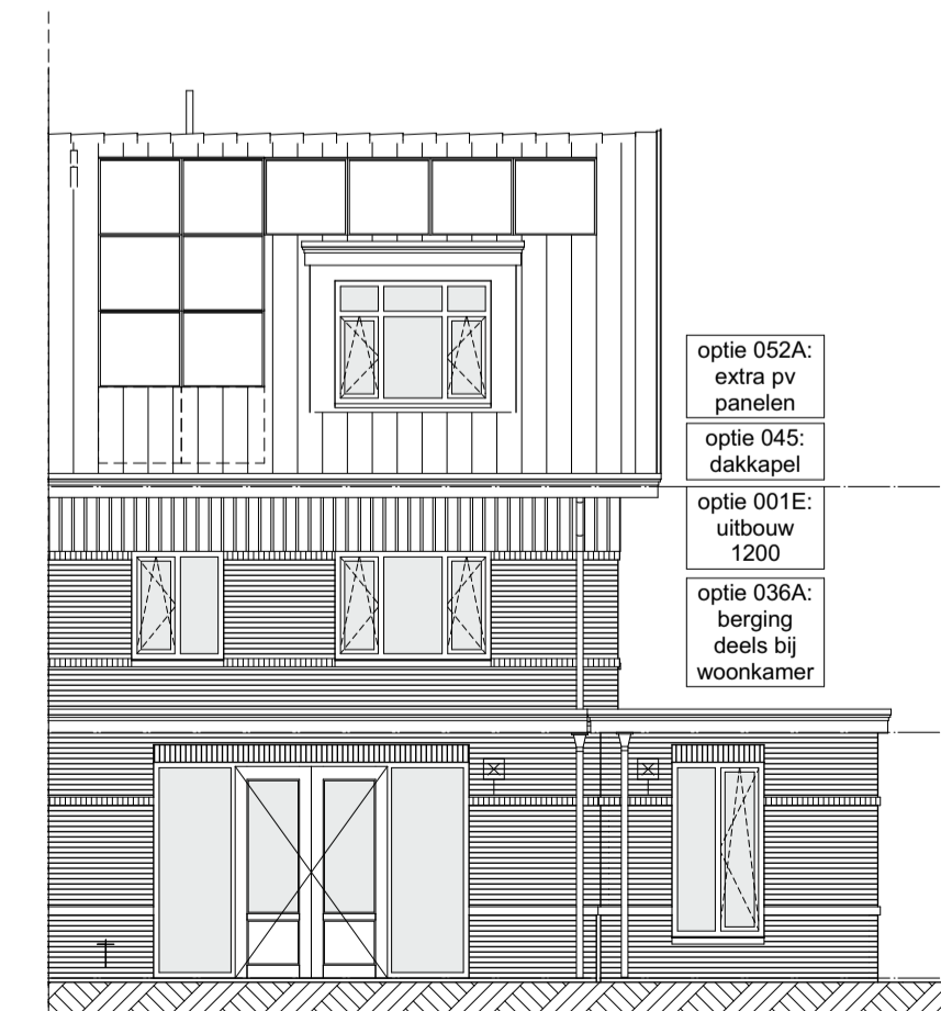
1:100 Achtergevel
