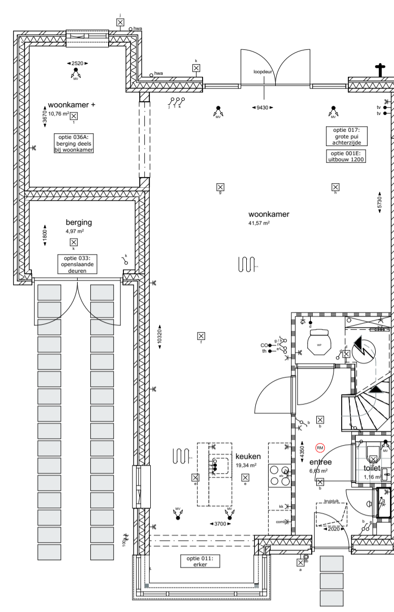
1:100 Begane grond erker niet mogelijk in combinatie met veranda
