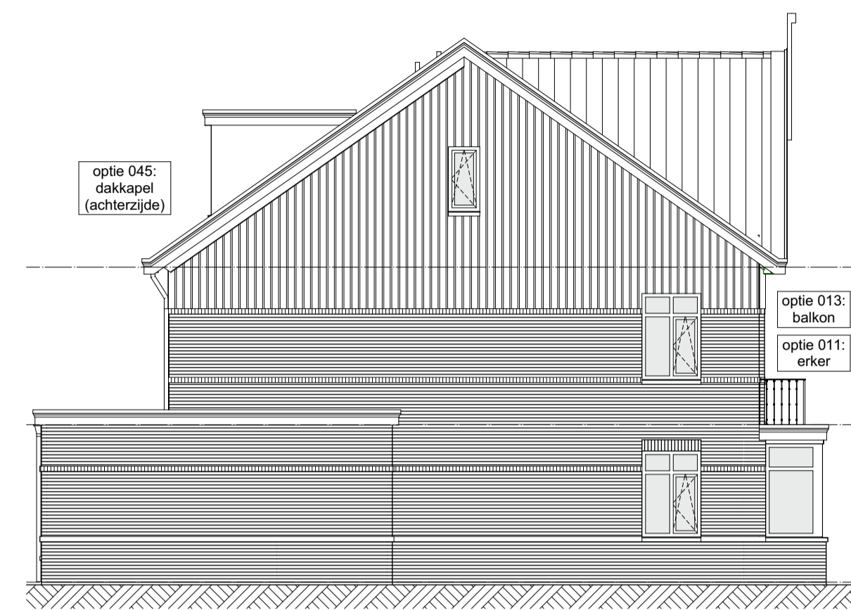
1:100 Linkergevel
