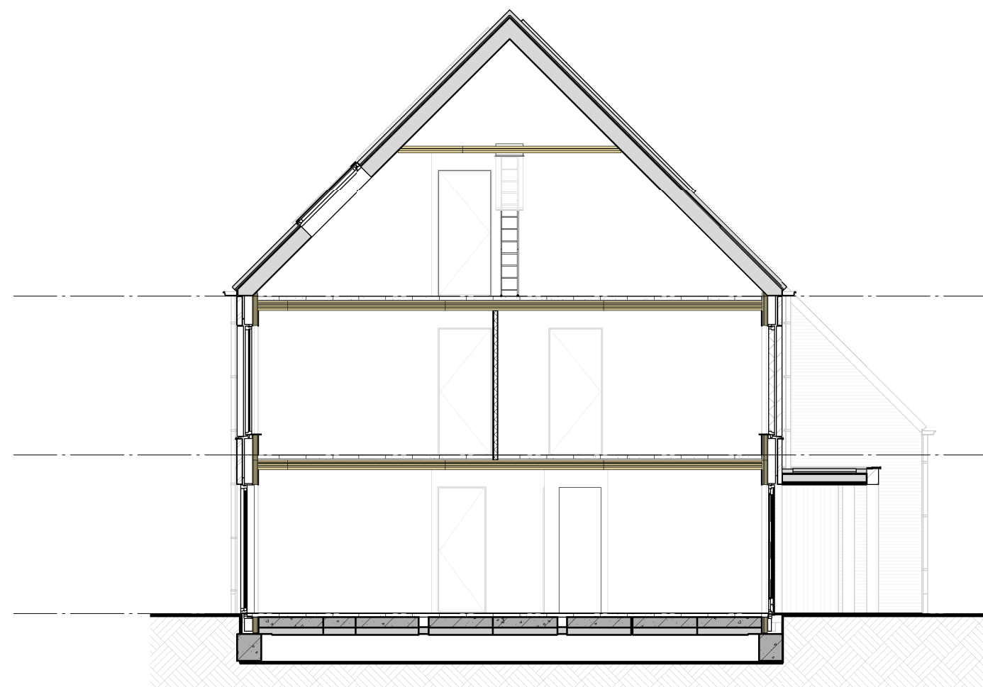
Doorsnede NN2 1 : 100
