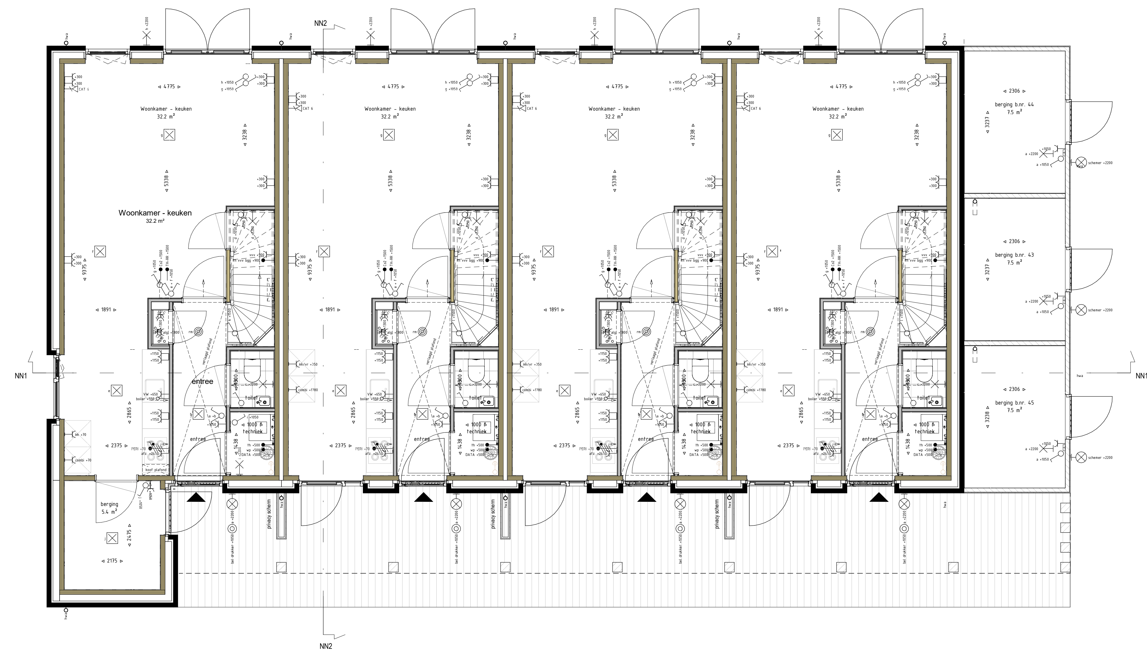
Begane grond 1:50
