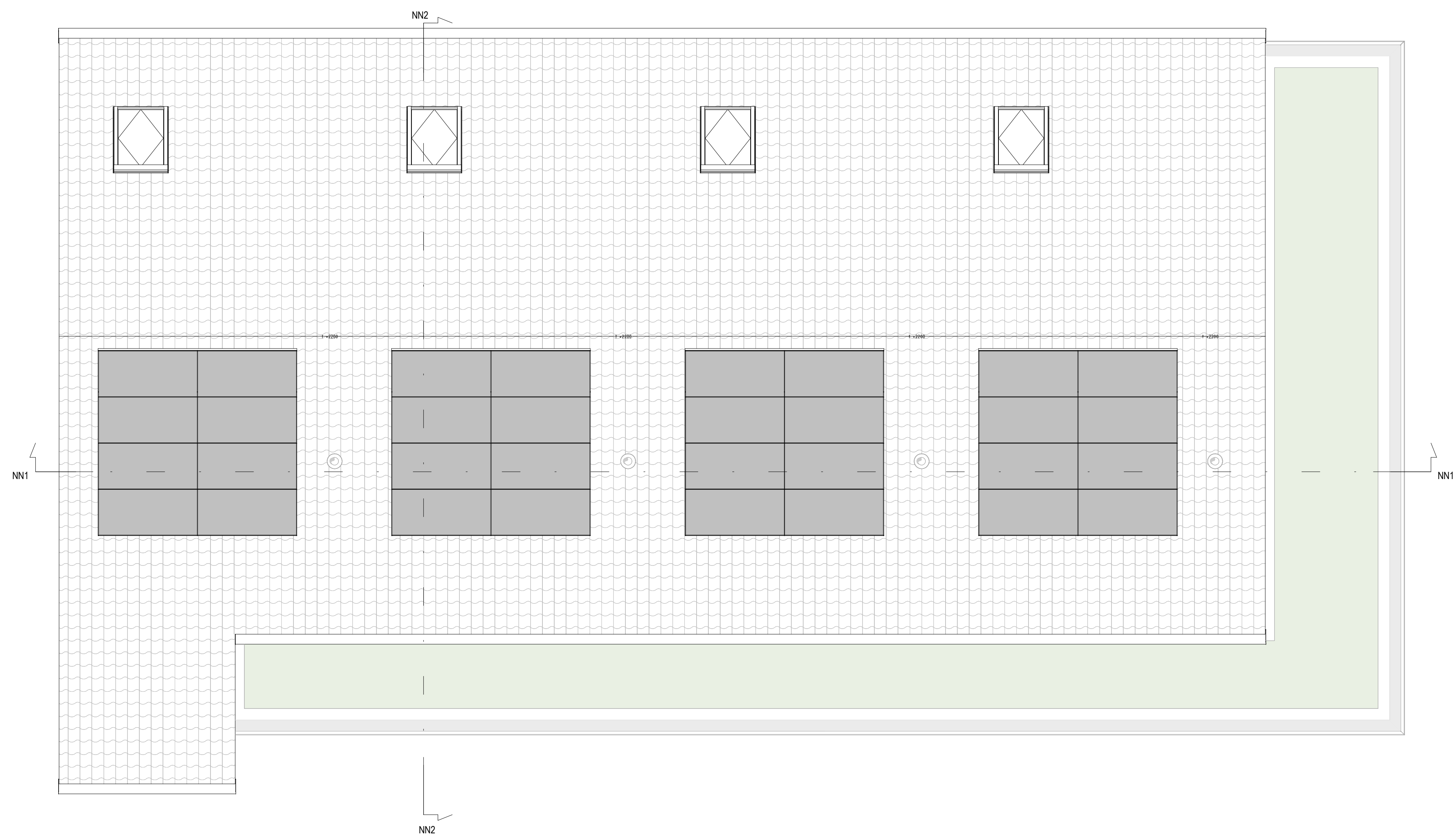
Dak blok N 1:50
