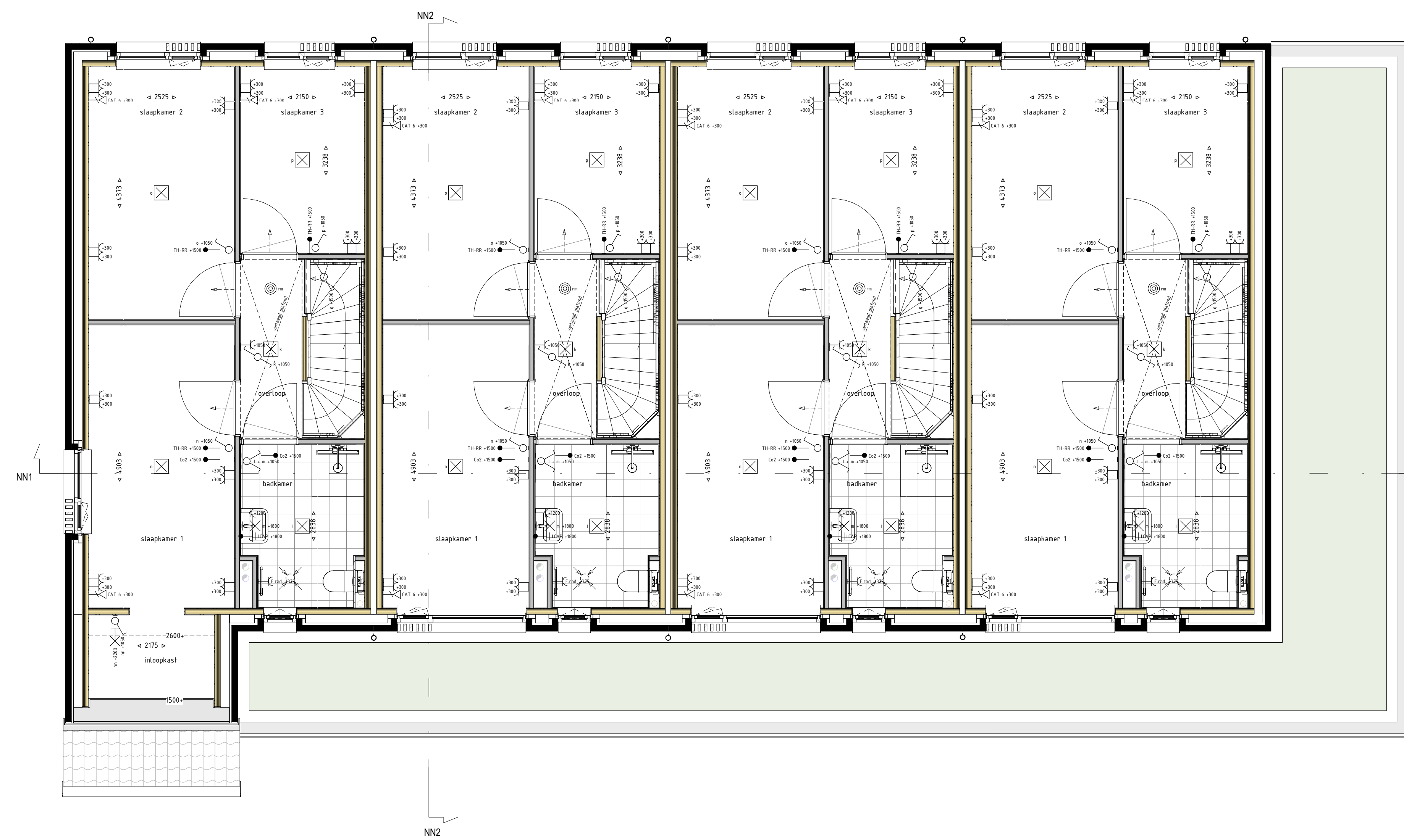
Eerste verdieping 1:50
