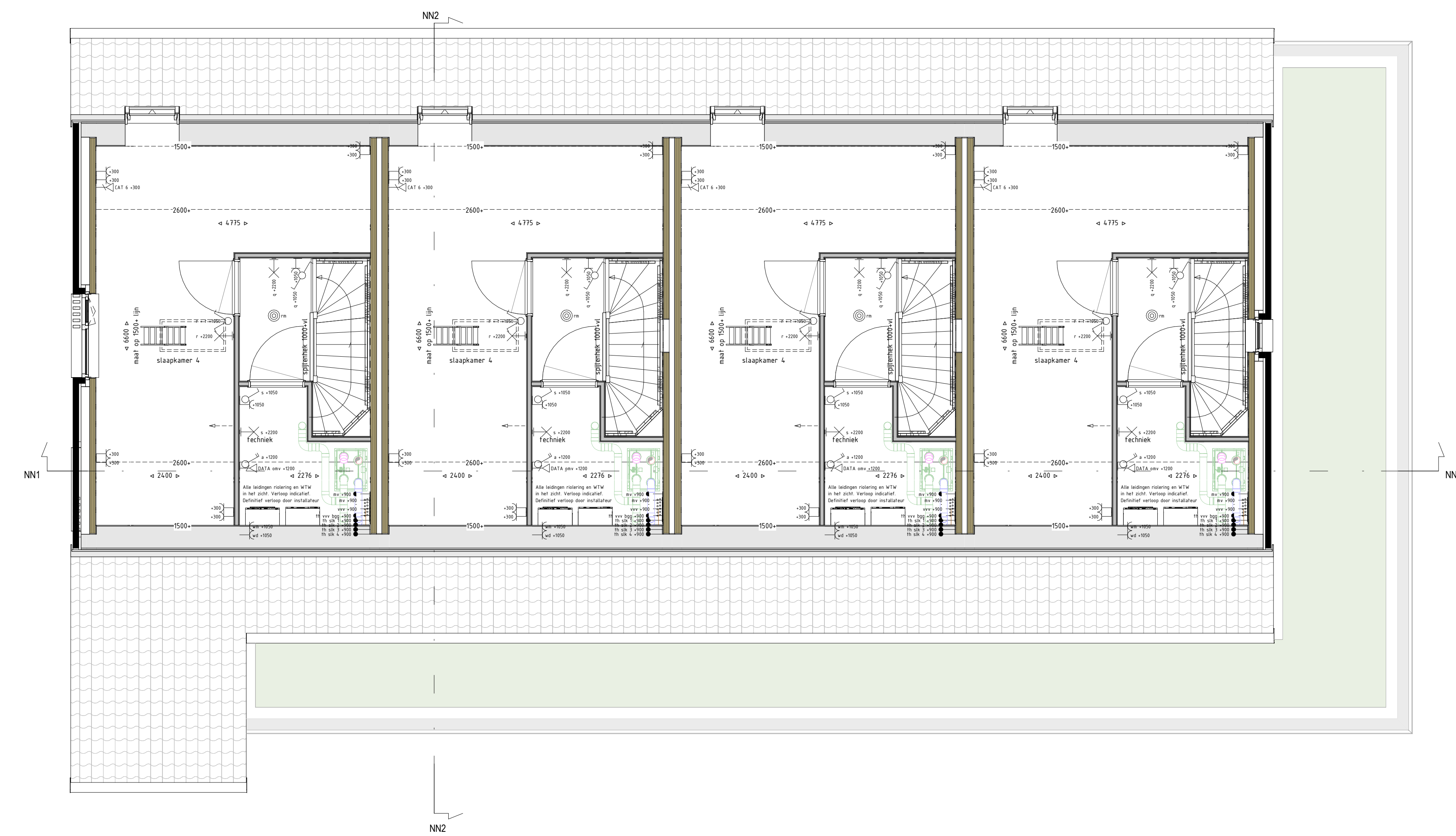
Tweede verdieping 1:50
