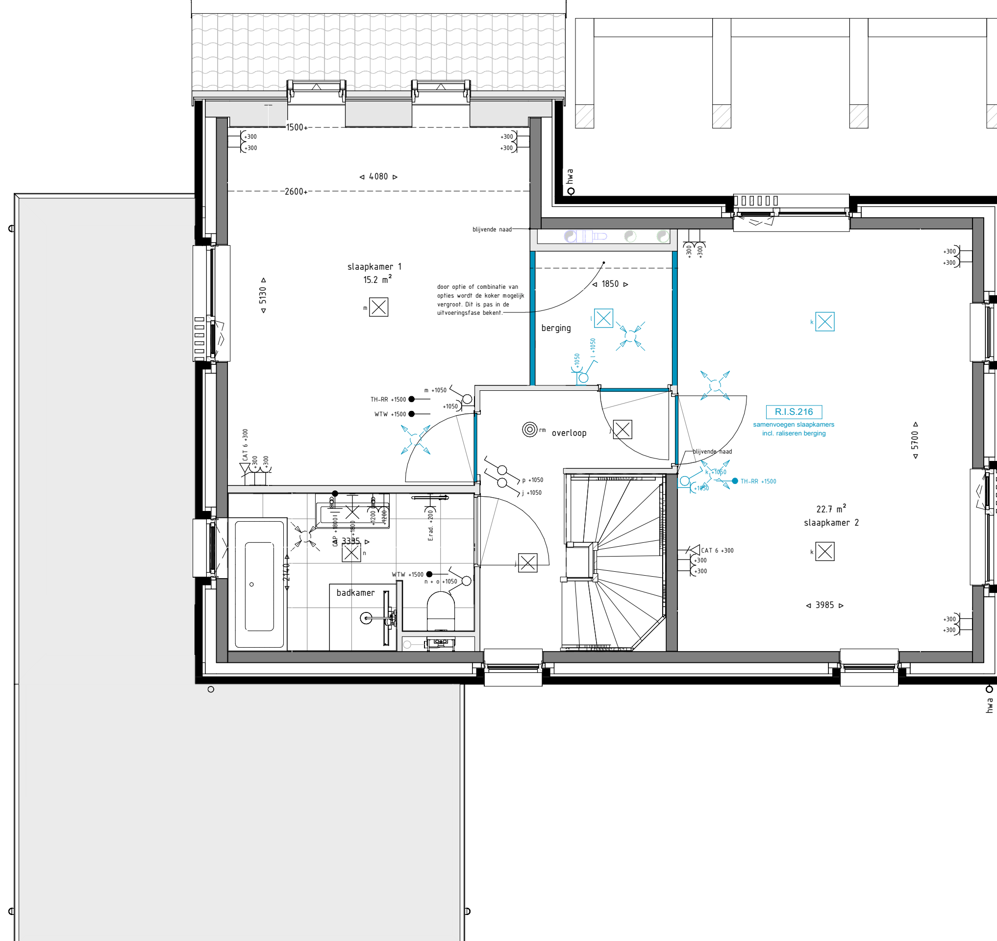
Eerste verdieping - berging en slaapkamers samenvoegen 1 : 50
