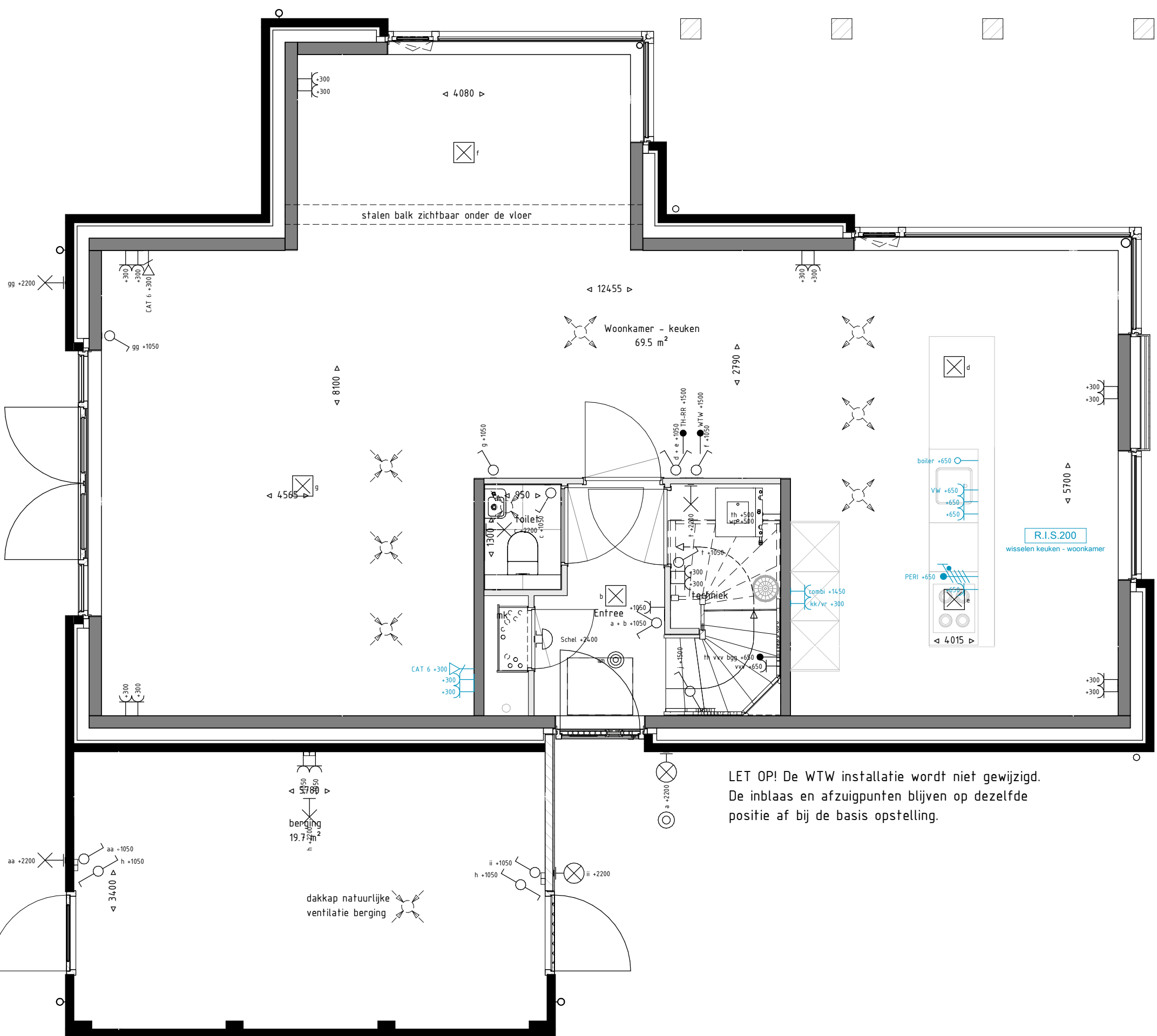
Begane grond - keuken 1 : 50
