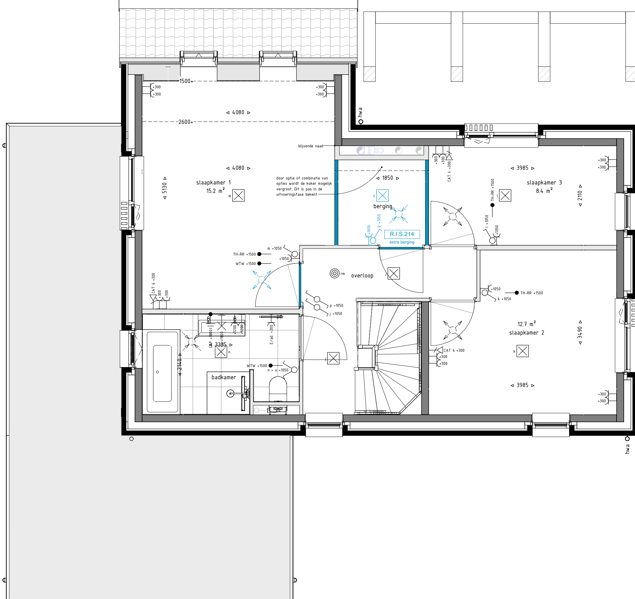
Eerste verdieping - berging 1 : 50
