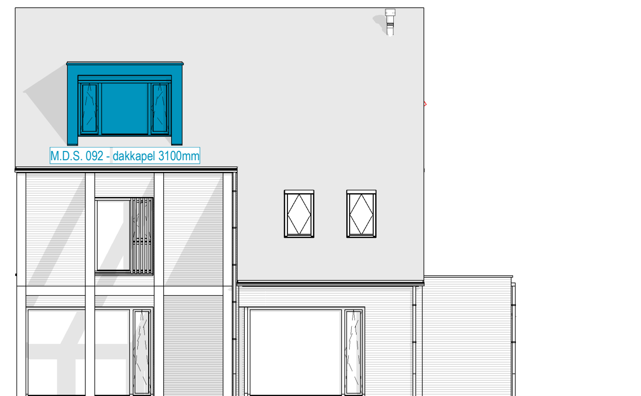
Achtergevel - dakkapel 1 : 100
