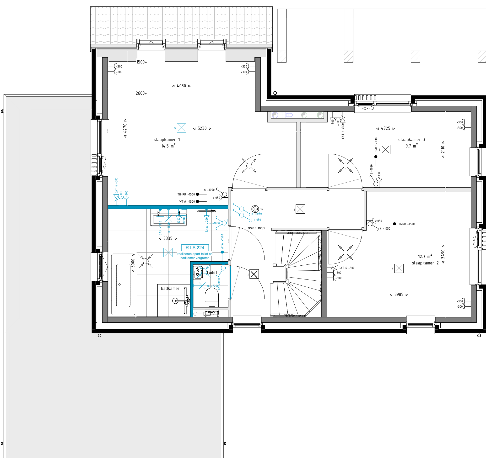
Eerste verdieping - toilet en badkamer apart 1 : 50
