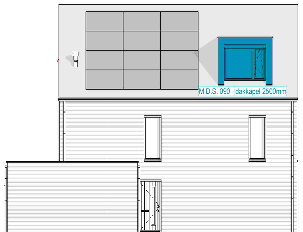
Voorgevel - dakkapel 1 : 100
