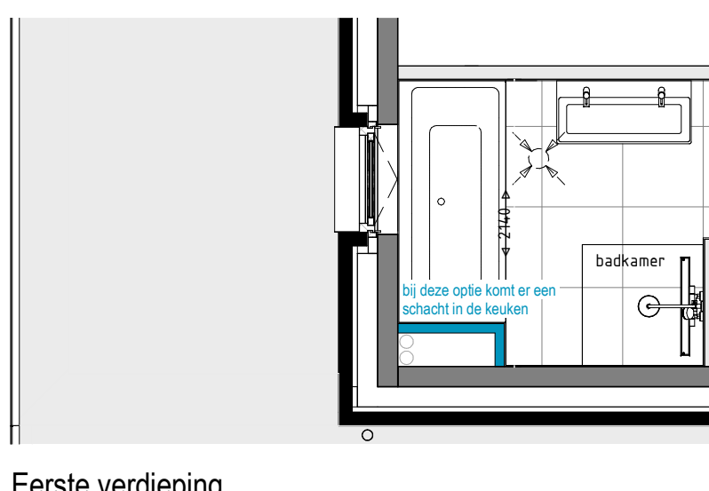
Eerste verdieping
