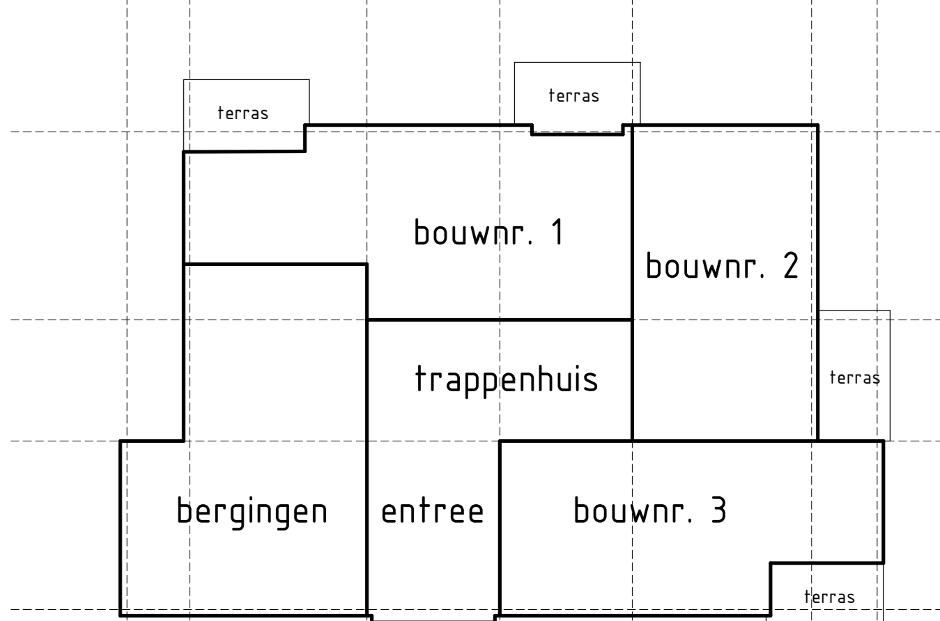
Situatie begane grond 1 : 250
