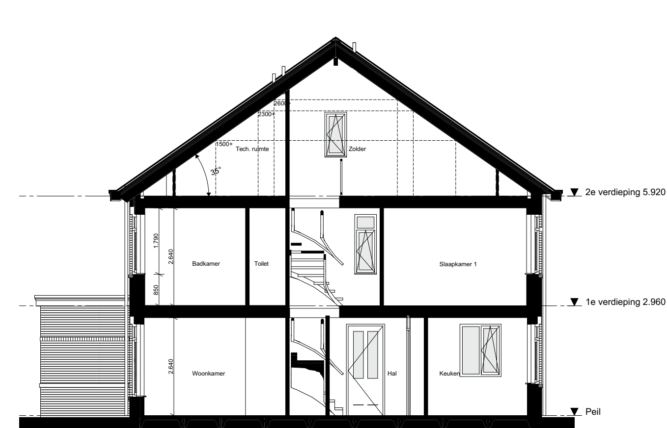
1:100 Doorsnede B-B
