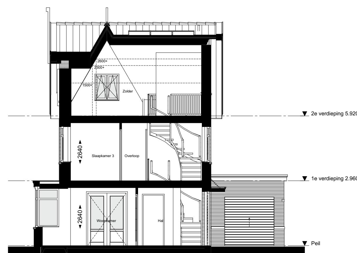
1:100 Doorsnede A-A
