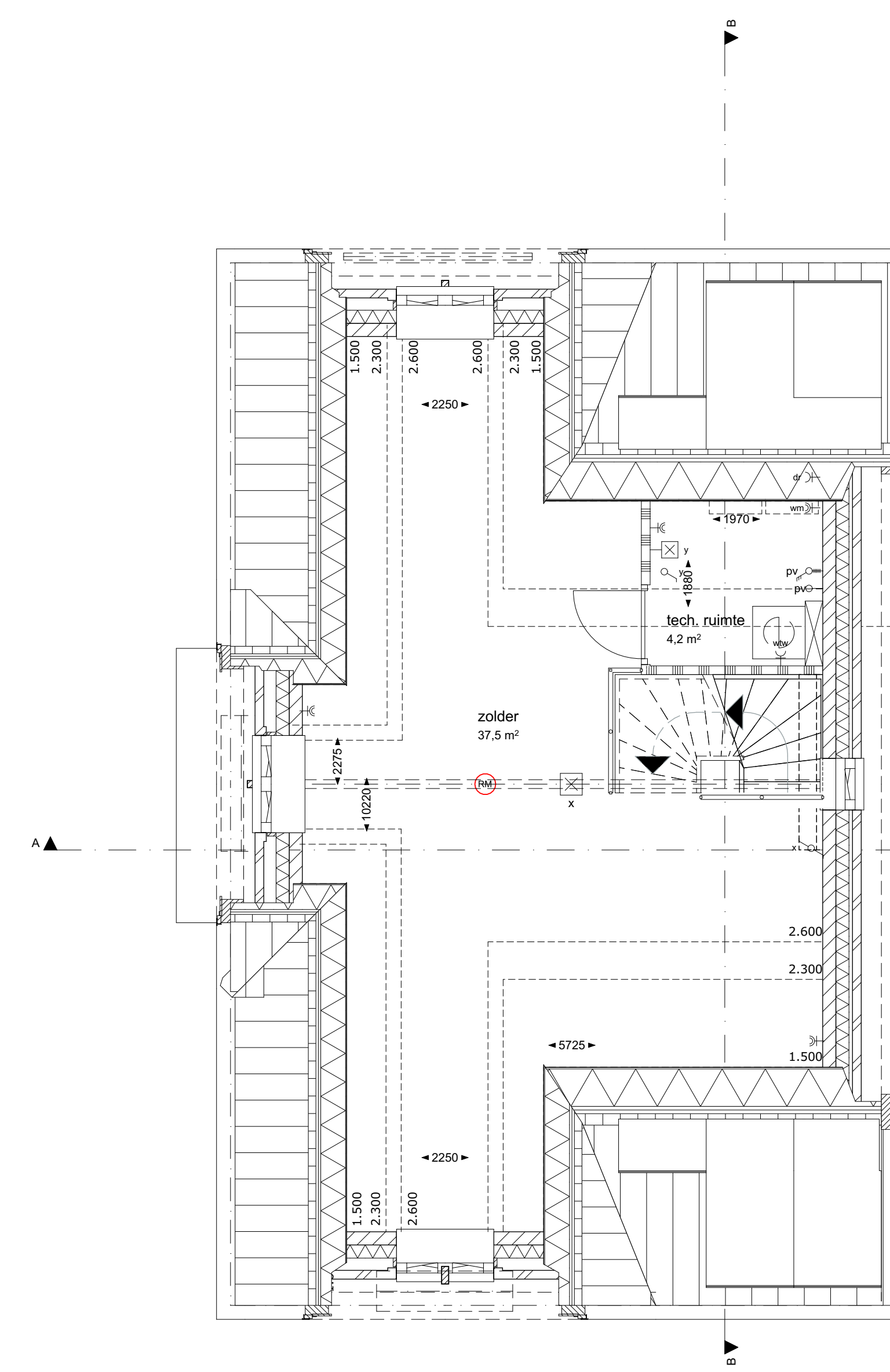
1:50 2e verdieping
