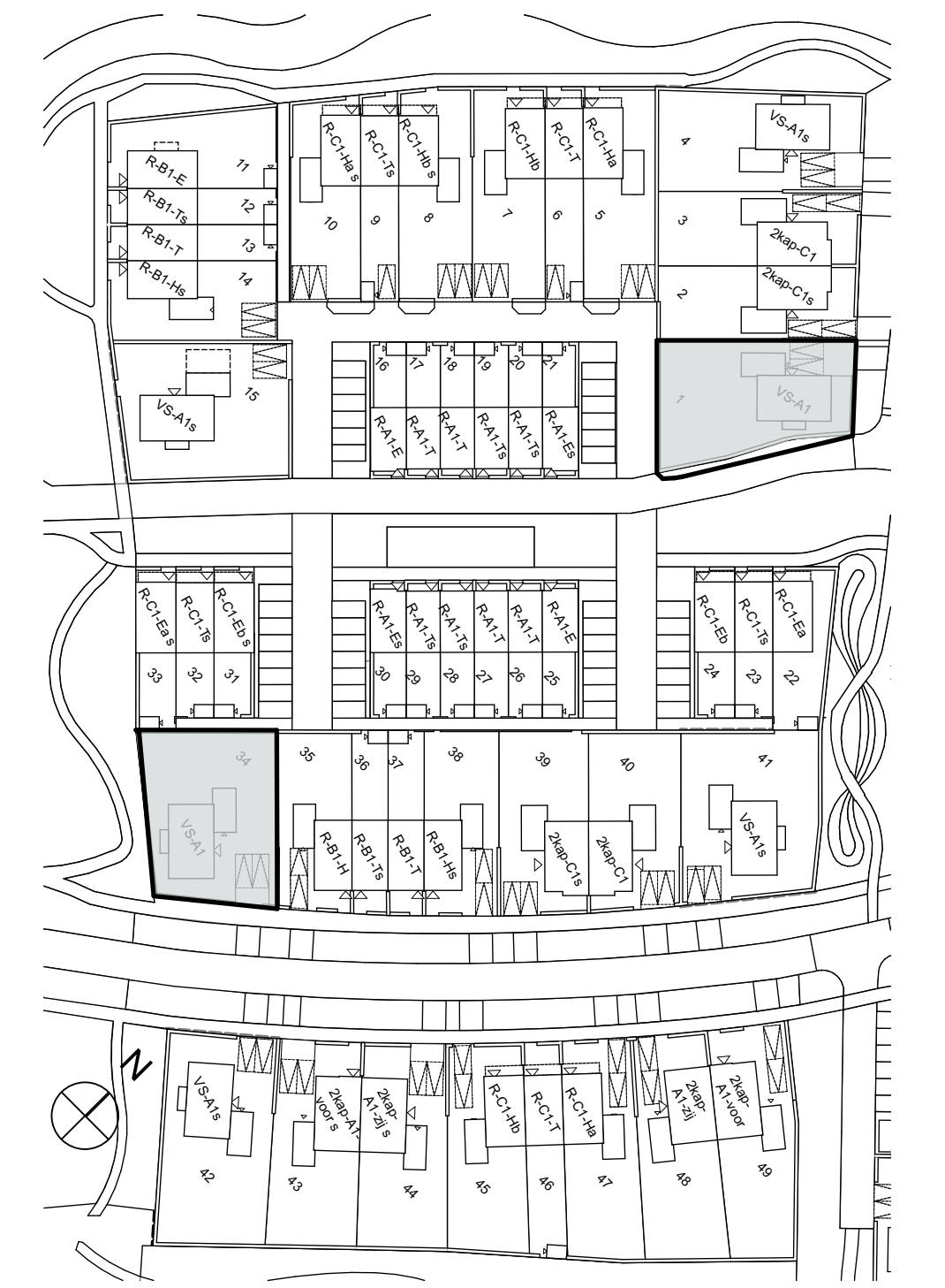
1:1000 Situatie
