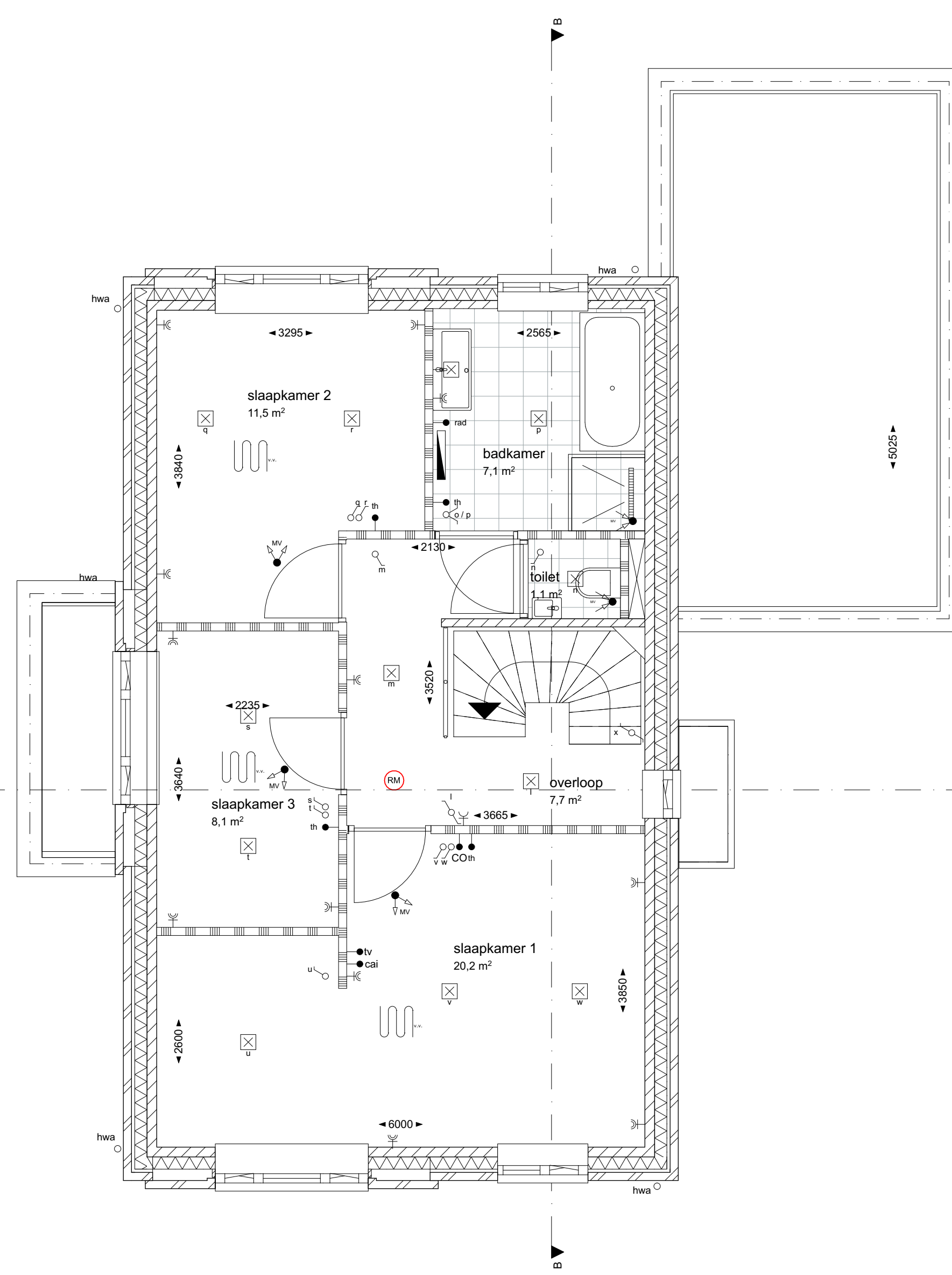
1:50 1e verdieping
