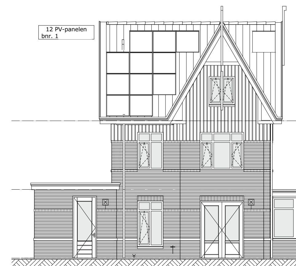
1:100 Achtergevel
