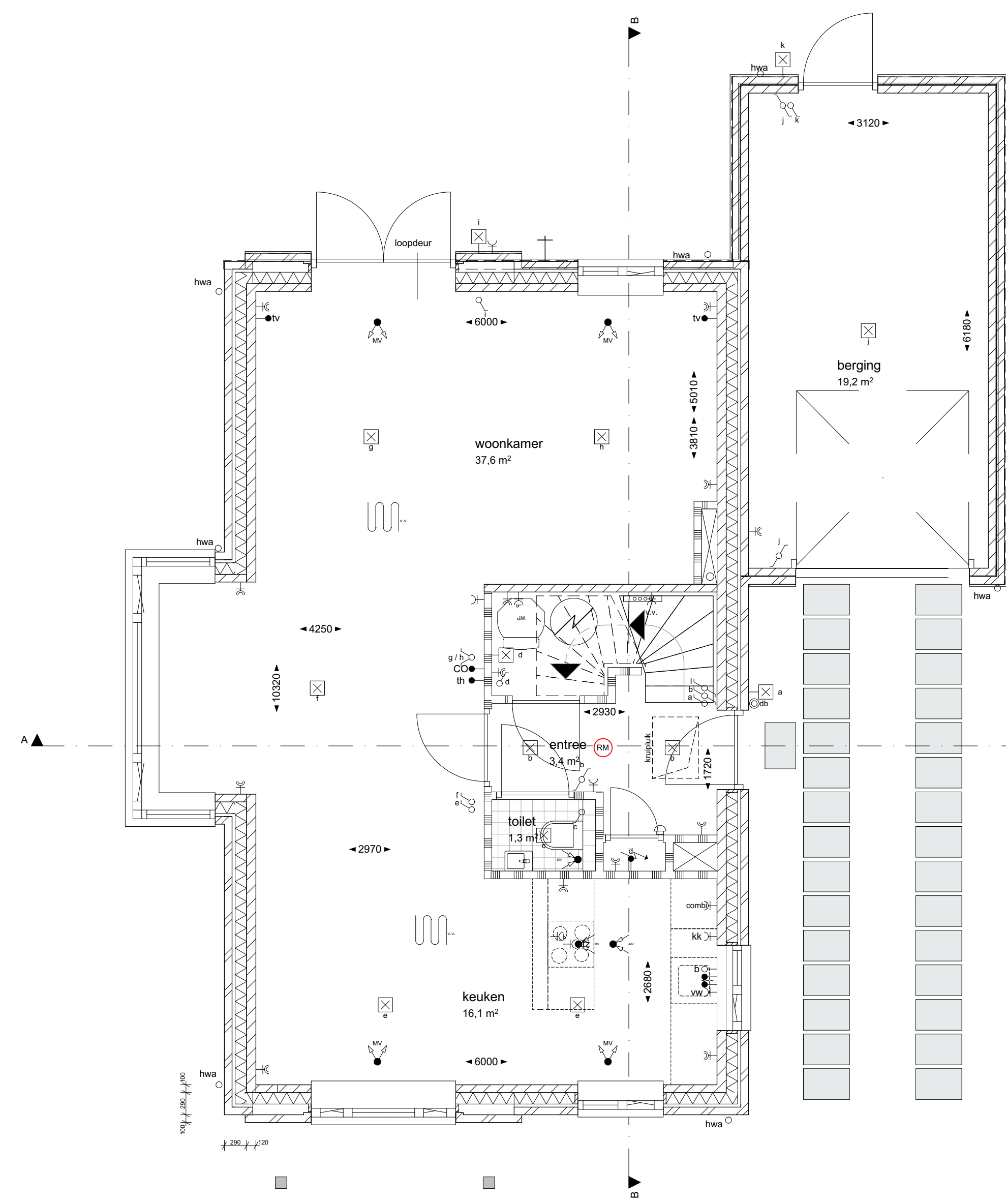
1:50 Begane grond
