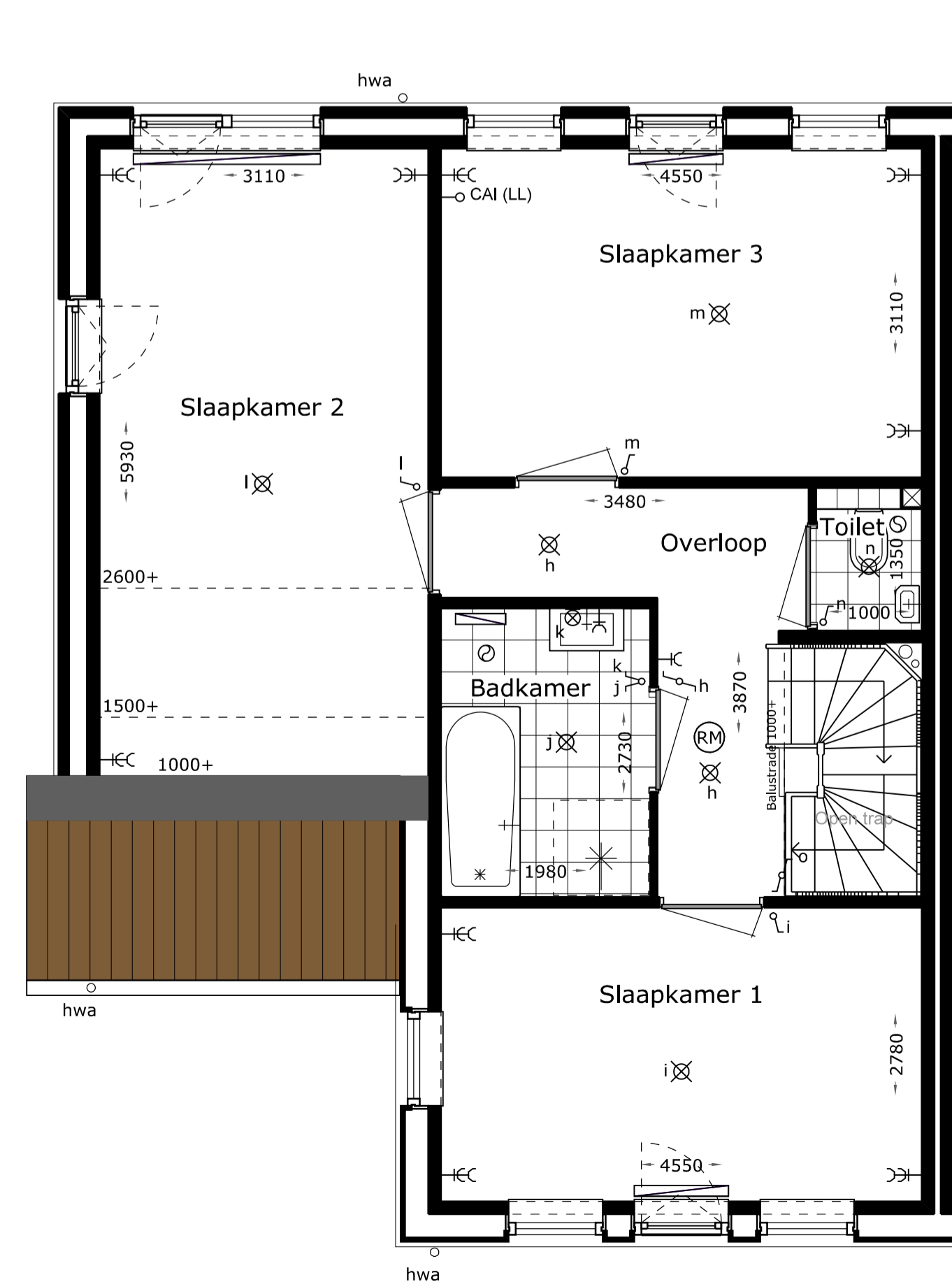
Verdieping
