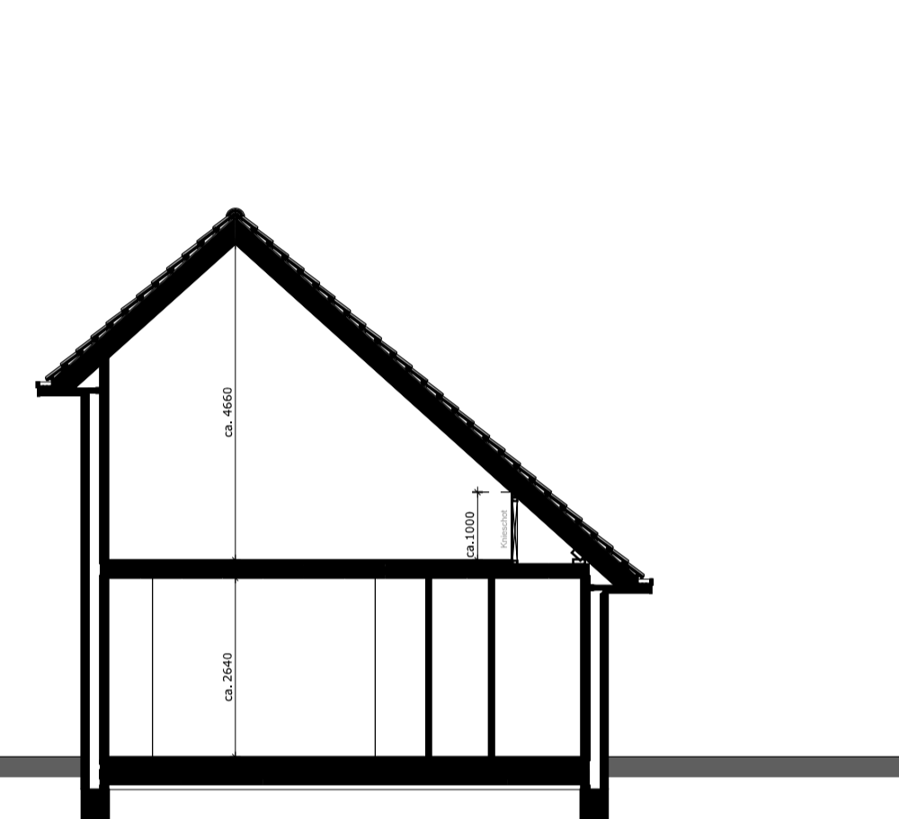
Principe doorsnede
