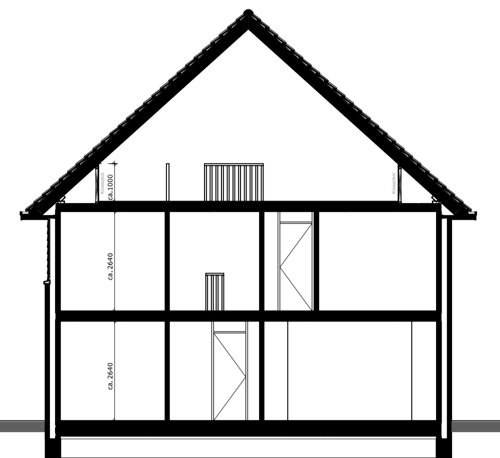
Principe doorsnede
