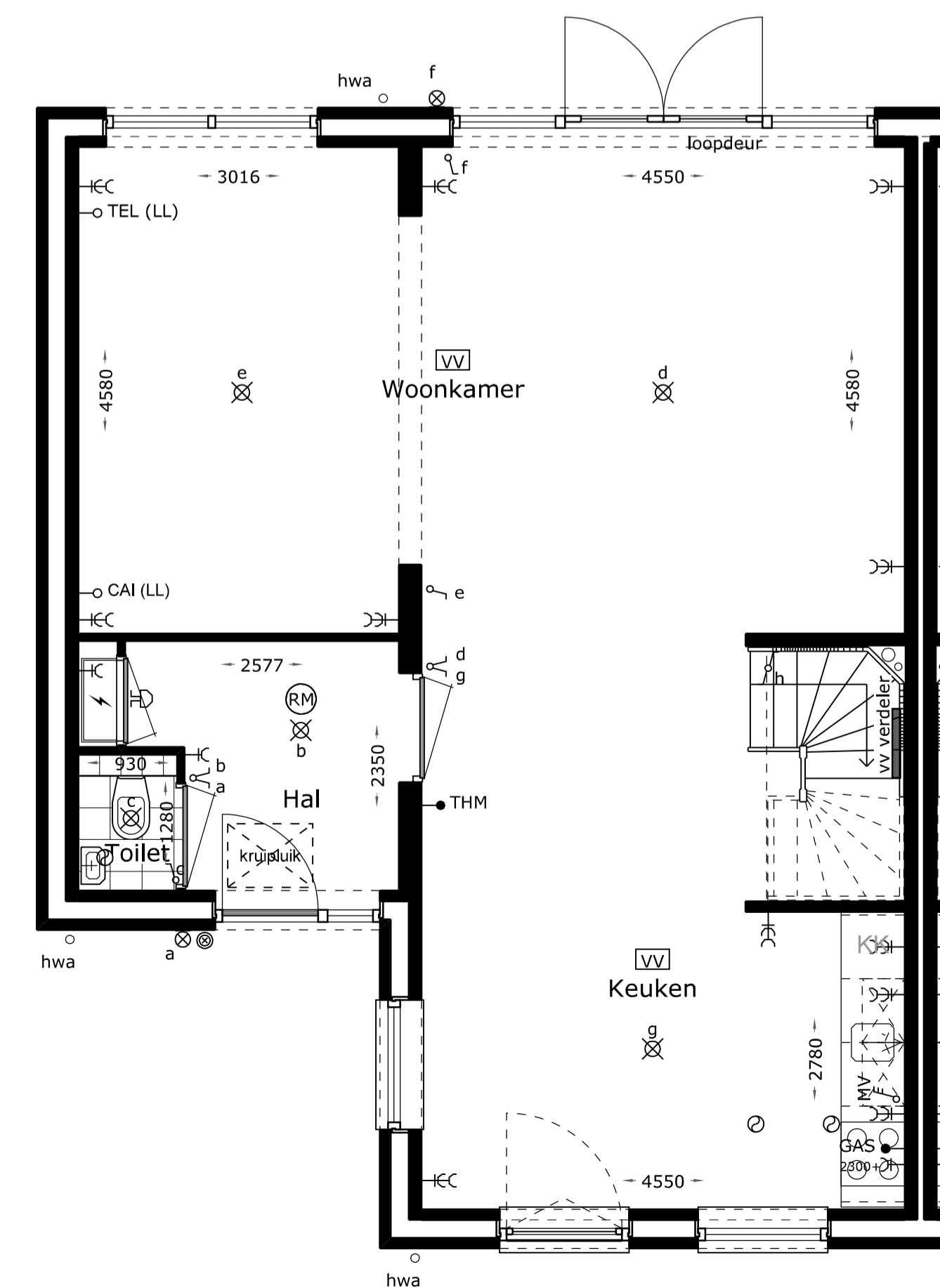
Begane grond
